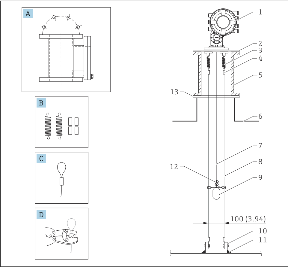
3 Führungsdraht; Maßangabe mm (in)
