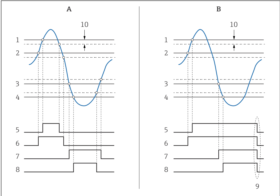
34 Prinzip der Grenzwertauswertung
