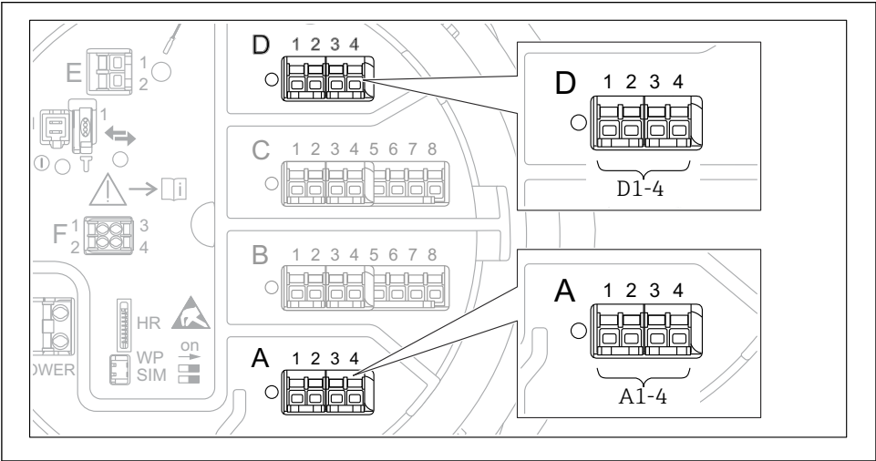
36 Mögliche Positionen der Modbus-Module (Beispiele); diese Module können je nach Geräteausführung auch in den Slots B oder C sitzen → 32.
