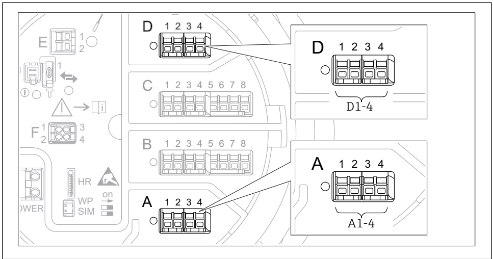
11 Bezeichnung der "Modbus"-, "V1"- oder "WM550"-Module (Beispiele); diese Module können je nach Geräteausführung auch in den Slots B oder C sitzen.
