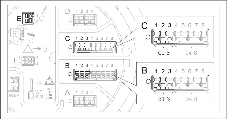
29 Mögliche Anschlüsse für HART-Loops
