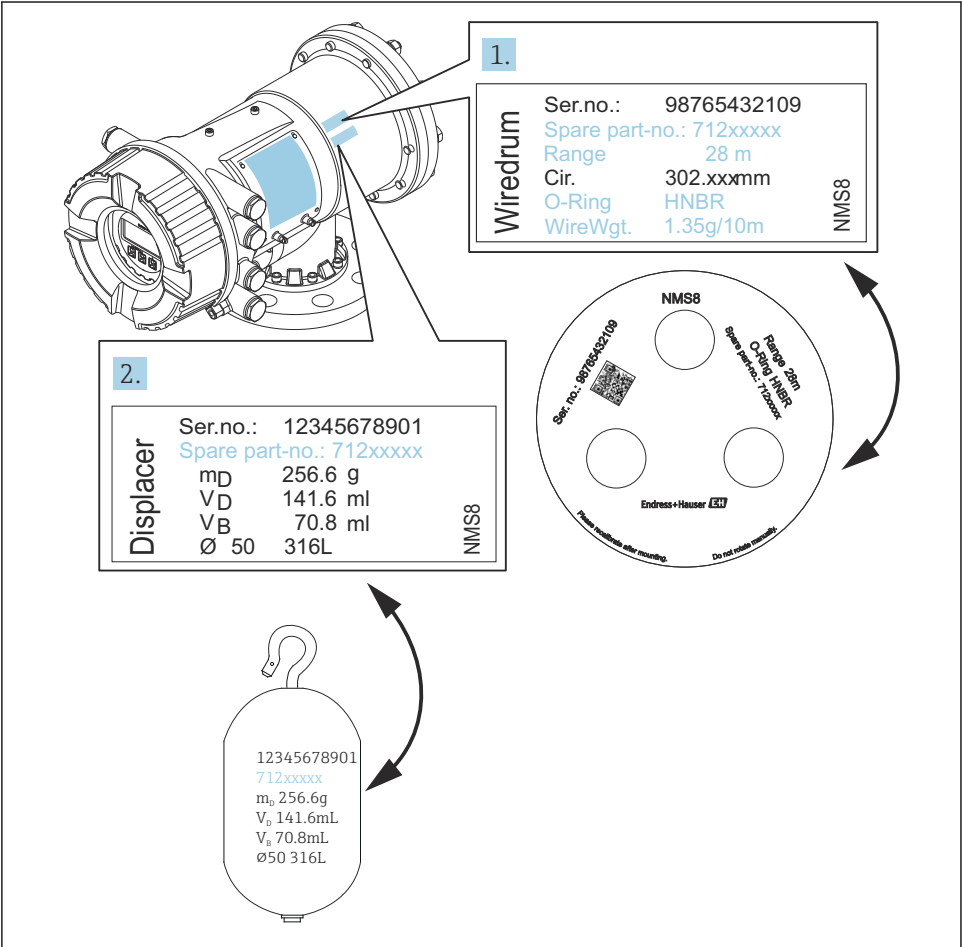
4 Verifizierung von Verdränger und Messtrommel
