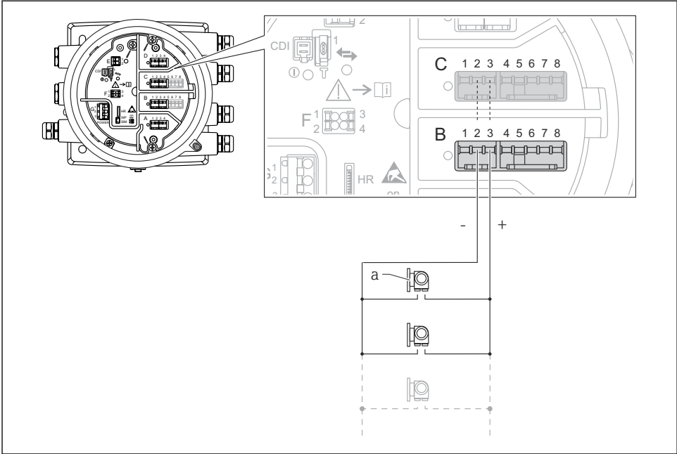
17 Aktive Nutzung des Analog I/O-Moduls im HART-Master-Modus
