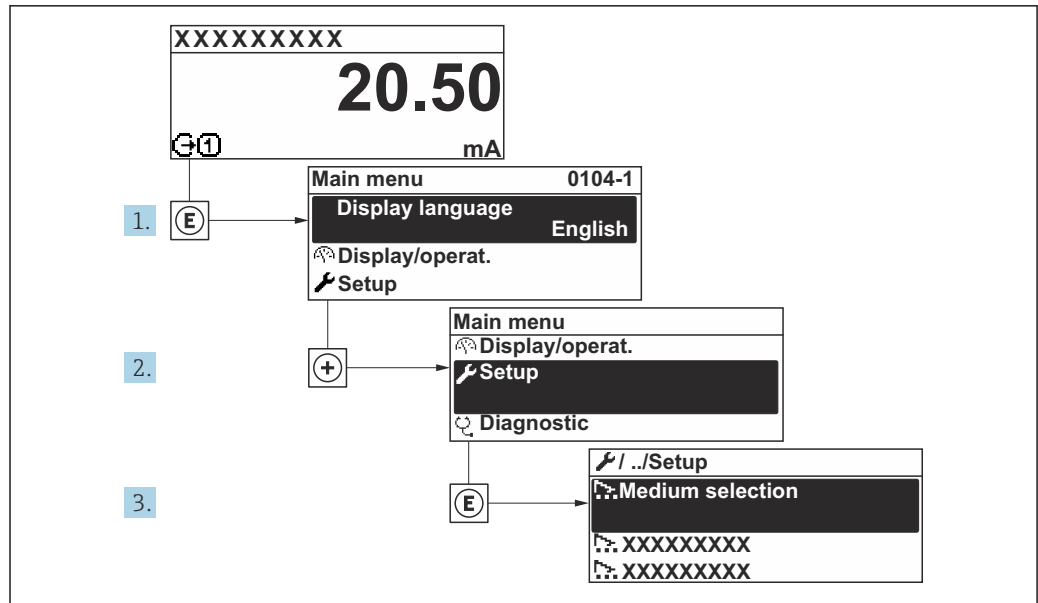
図 41 現場表示器の表示例
