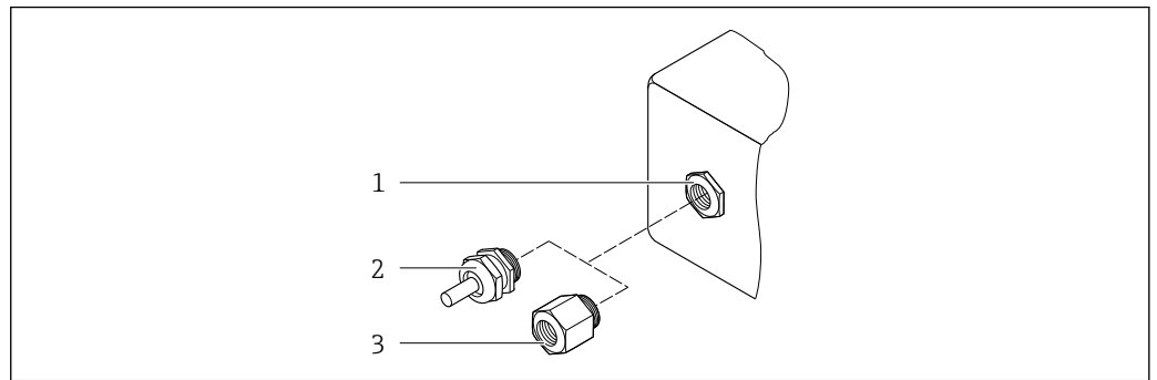
図 49 可能な電線管接続口/ケーブルグランド
