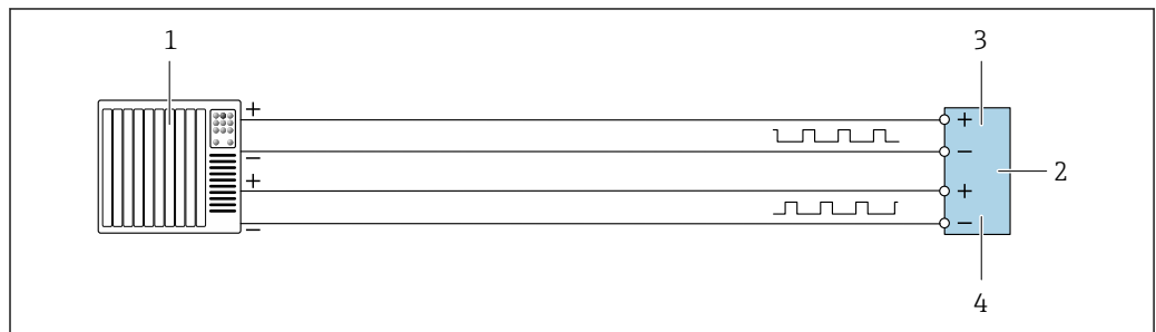
図 27 ダブルパルス出力 (アクティブ) の接続例
