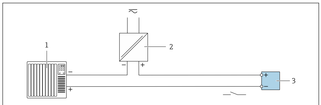
図 29 リレー出力（パッシブ）の接続例
