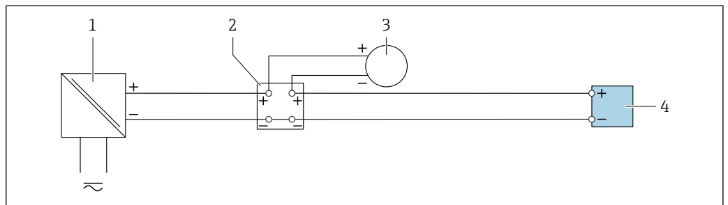
図 30 4~20 mA 電流入力の接続例
