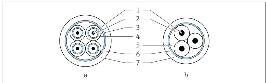
图 9 电缆横截面
