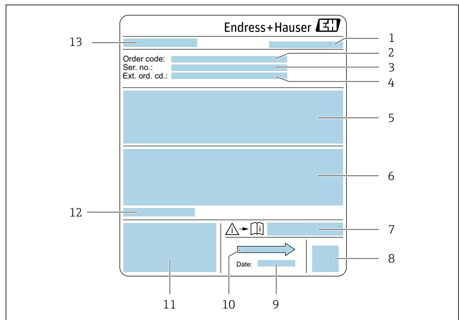
2 Exemplo de uma etiqueta de identificação de sensor
