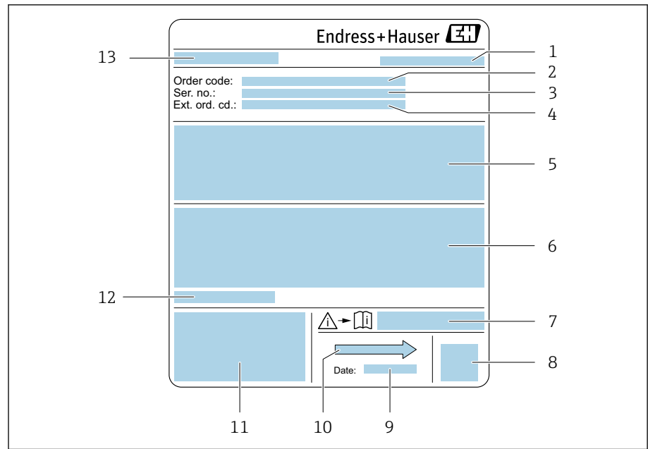
图 2 传感器的铭牌示意图
