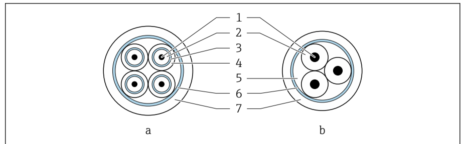
图 8 电缆横截面
