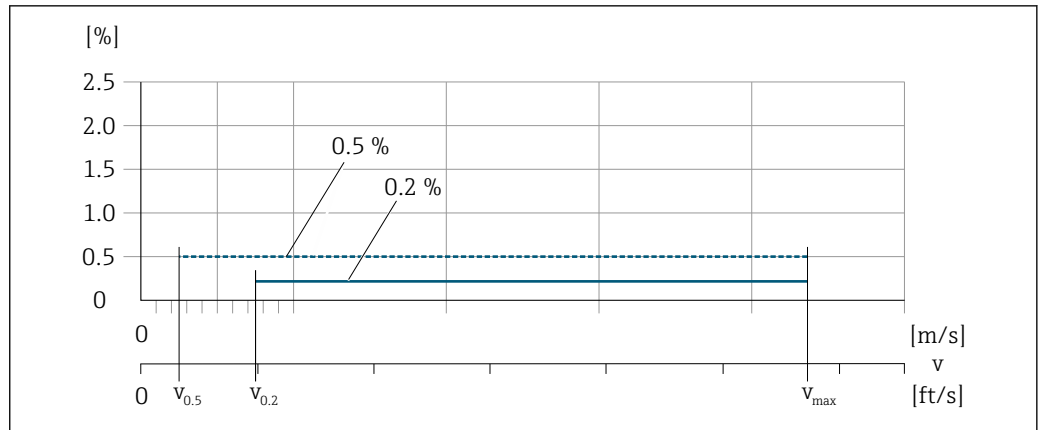
图 31 设计测量精度 (% o.r.)
