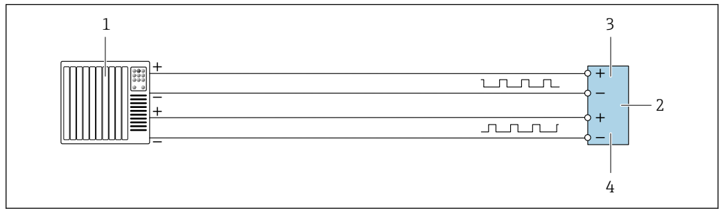
图 13 接线实例：双脉冲输出（有源信号）
