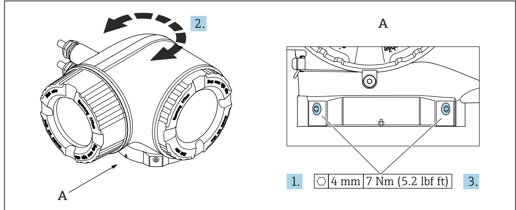
图 6 防爆型外壳
