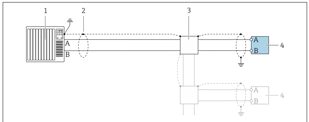
图 8 接线实例：Modbus RS485，非危险区和 Zone 2/Div. 2 防爆场合
