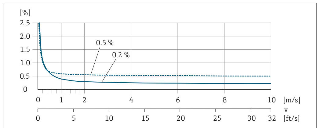
30 最大测量误差 (% o.r.)
