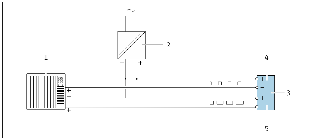
图 14 接线实例：双脉冲输出（无源信号）
