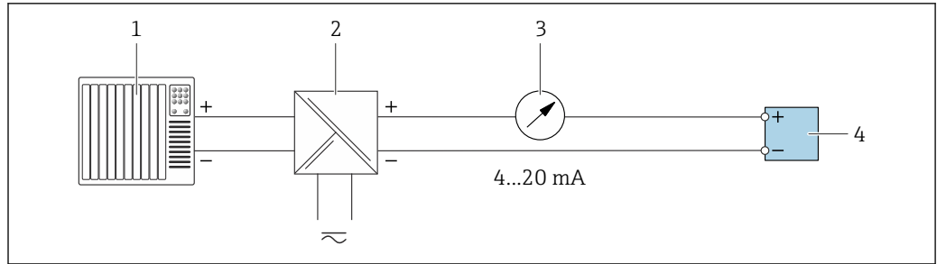
图 10 接线实例：4...20 mA 电流输出（无源信号）
