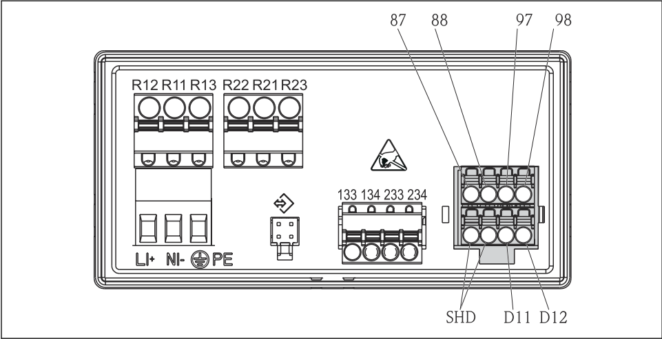
图 2 变送器的电气连接示意图
