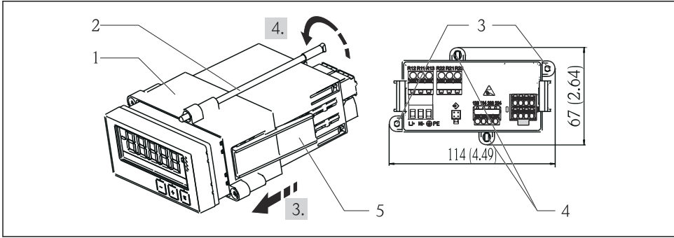
图 1 安装在面板中
