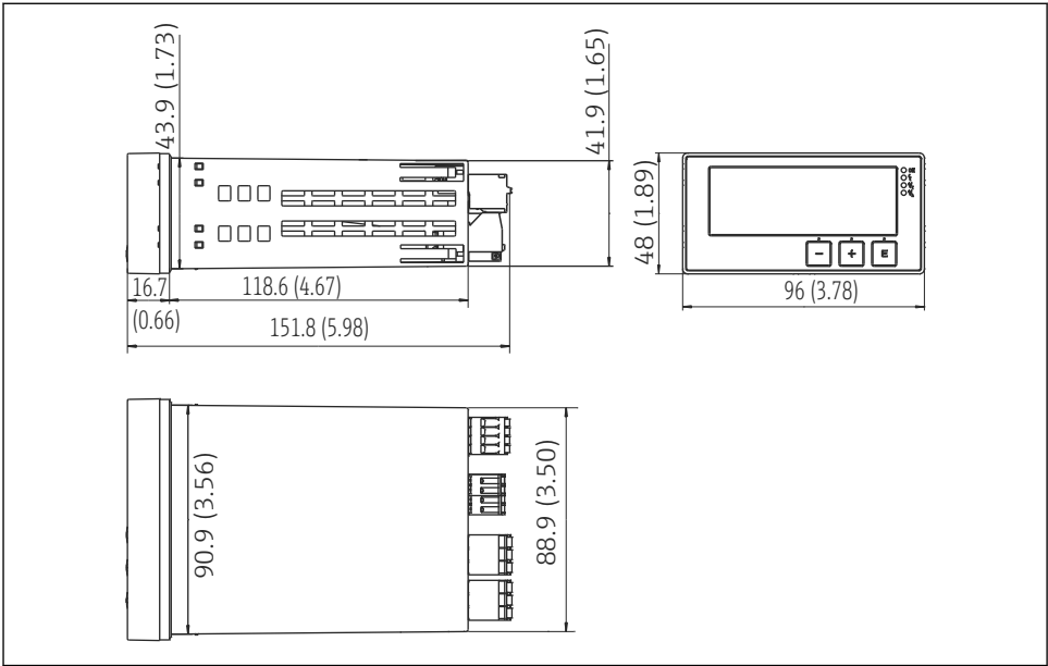
图 6 变送器的外形尺寸示意图；单位：mm (in)
