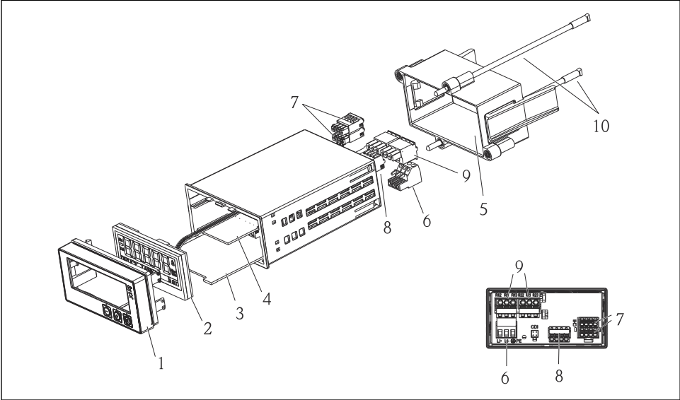
4 备件示意图
