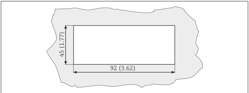
图 5 安装孔口的外形尺寸示意图; 单位: mm (in)
