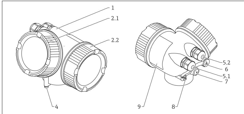
36 Material; GT19 housing
