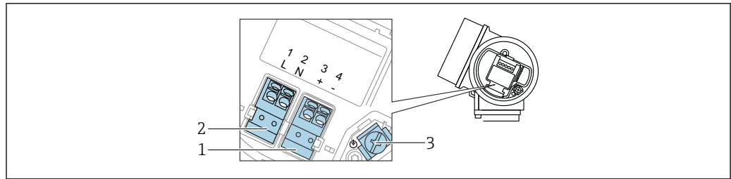
14 Klemmenbelegung 4-Draht: 4 ... 20 mA HART (90 ... 253 V AC )
