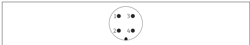
21 Pinbelegung Stecker 7/8"
