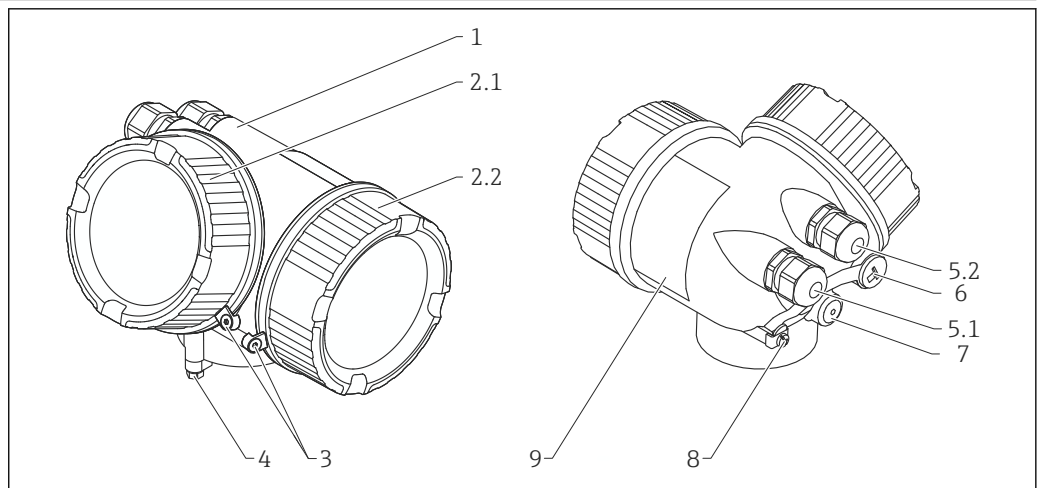
42 Material; Gehäuse GT20
