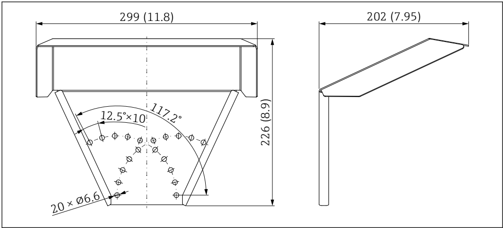
52 Abmessungen. Maßeinheit mm (in)
