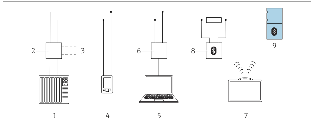
47 Möglichkeiten der Fernbedienung via HART-Protokoll
