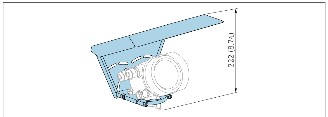
51 Bauhöhe. Maßeinheit mm (in)
