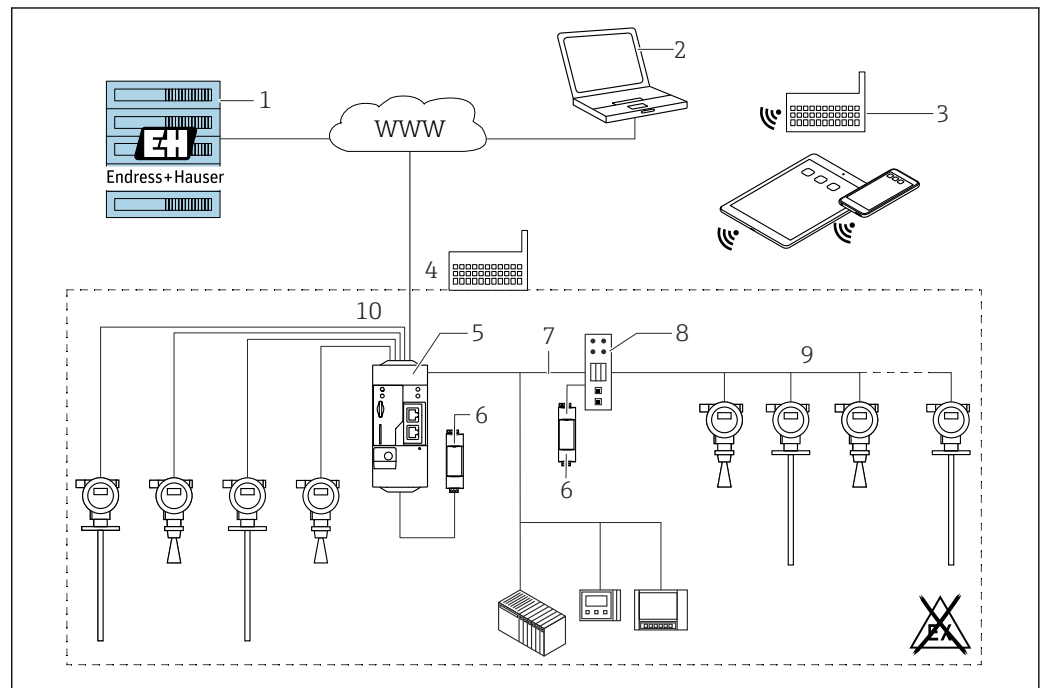
50 Beispielhafte Bestandsführungsplattform mit SupplyCare Hosting SCH30
