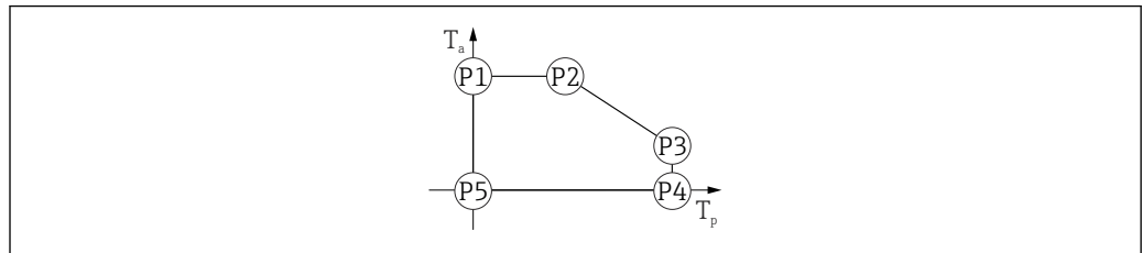
14 Obudowa z tworzywa sztucznego; zakres temperatur medium: 0 \dots +150 \text{ }^\circ\text{C} ( +32 \dots +302 \text{ }^\circ\text{F} ) z zatwierdzeniem CSA C/US
