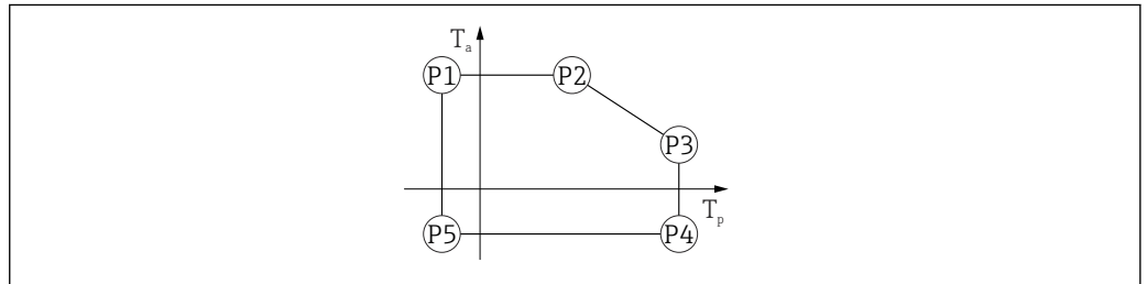
29 Materiał obudowy: stal k.o. 316L; zakres temperatury medium procesowego: -40 \dots +280 \text{ }^\circ\text{C} ( -40 \dots +536 \text{ }^\circ\text{F} )
