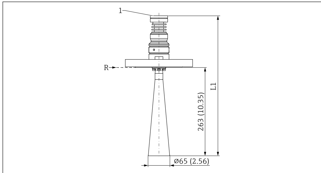
35 Wymiary anteny stożkowej DN65 - kołnierzowe przyłącze procesowe. Jednostka miary mm (in)
