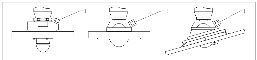
9 Antena z adapterem przyłącza do przedmuchu
