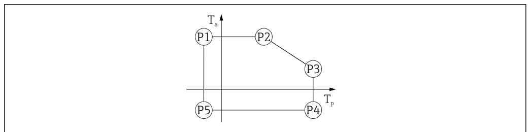
30 Materiał obudowy: stal k.o. 316L; zakres temperatury medium procesowego: -40 \dots +450 \text{ }^\circ\text{C} ( -40 \dots +842 \text{ }^\circ\text{F} )
