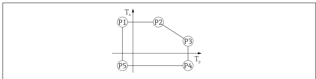
15 Obudowa z tworzywa sztucznego; zakres temperatur medium: -40 \dots +200 \text{ }^\circ\text{C} ( -40 \dots +392 \text{ }^\circ\text{F} )
