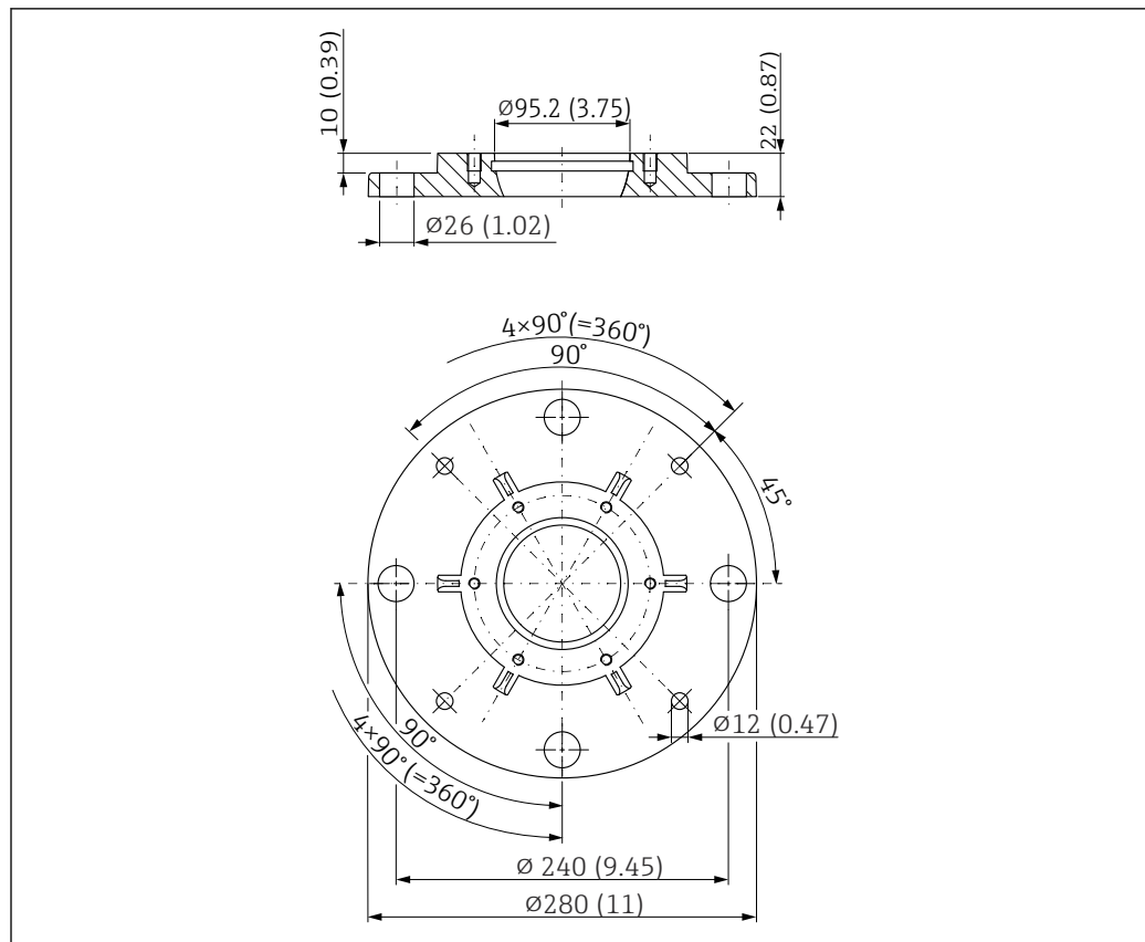
51 Wymiary kołnierza UNI 6"/DN150/150A dla anten z pozycjonerem. Jednostka miary mm (in)
