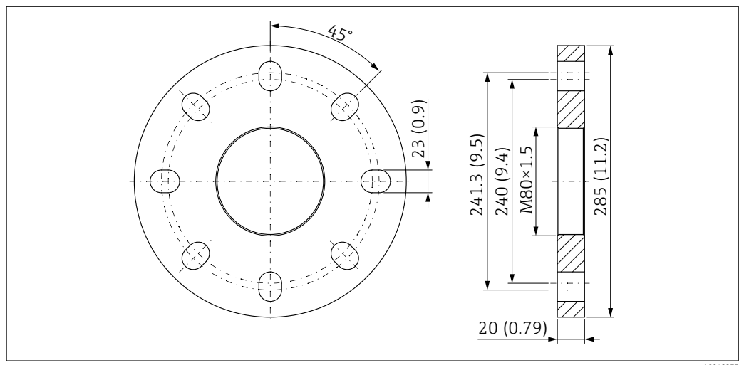
44 Kołnierz UNI 6"/DN150/150A do anteny soczewkowej, wypukłej, 50 mm (2 in) z przyłączem do przedmuchu anteny. Jednostka miary mm (in)
