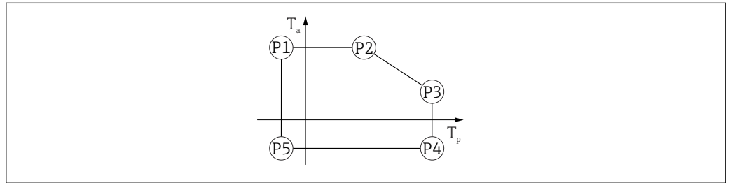
11 Obudowa z tworzywa sztucznego; zakres temperatur medium: -40 ... +80 °C (-40 ... +176 °F)
