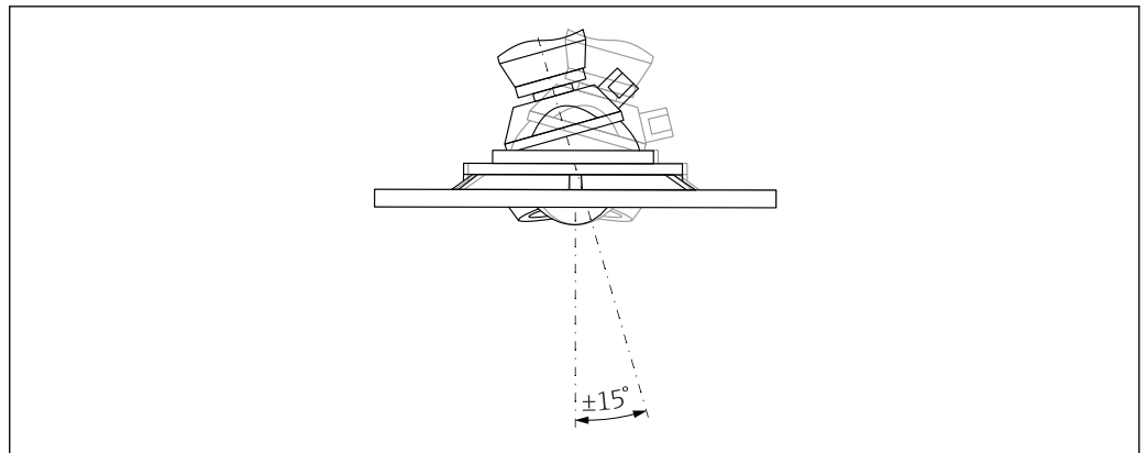
8 Antena do montażu czołowego z pozycjonerem
