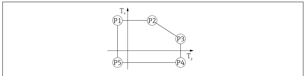
17 Materiał obudowy: tworzywo sztuczne; zakres temperatury medium procesowego: -40 ... +280 °C (-40 ... +536 °F)
