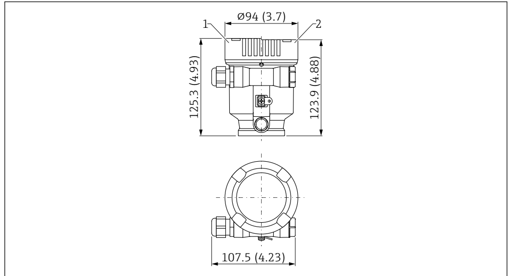
31 Wymiary obudowy jednokomorowej z tworzywa sztucznego (PBT)
