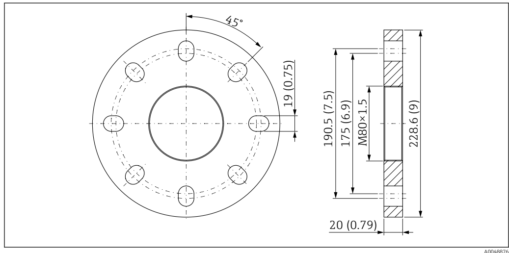
43 Kołnierz UNI 4"/DN100/100A do anteny soczewkowej, wypukłej, PTFE, 50 mm (2 in) z przyłączem do przedmuchu anteny. Jednostka miary mm (in)
