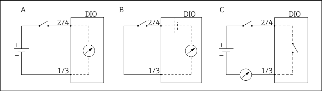
図 14 デジタル I/O モジュールの操作モード
