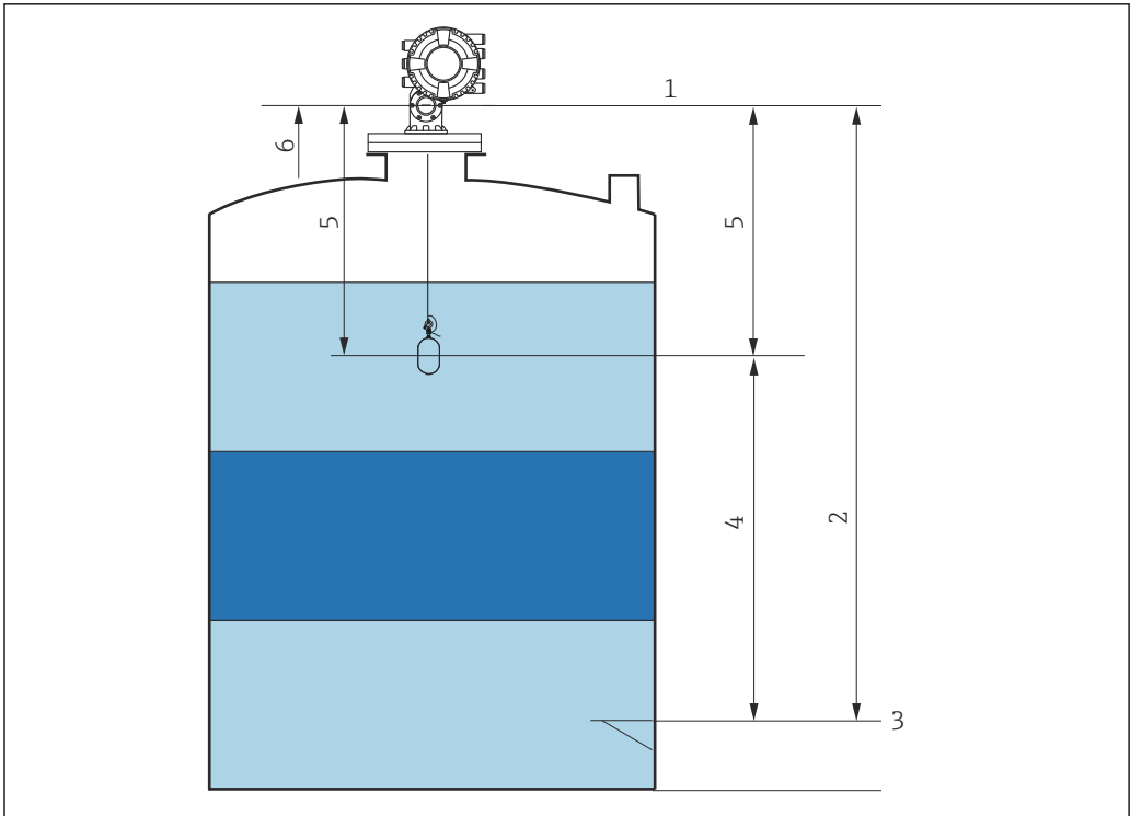
図 7 液面計測スタンバイゲージコマンドの実行時に液面上昇を待機するディスプレイサ 1 機器基準高さ 2 空 3 基準プレート 4 スタンバイレベル 5 スタンバイ距離 6 リファレンスポジション
