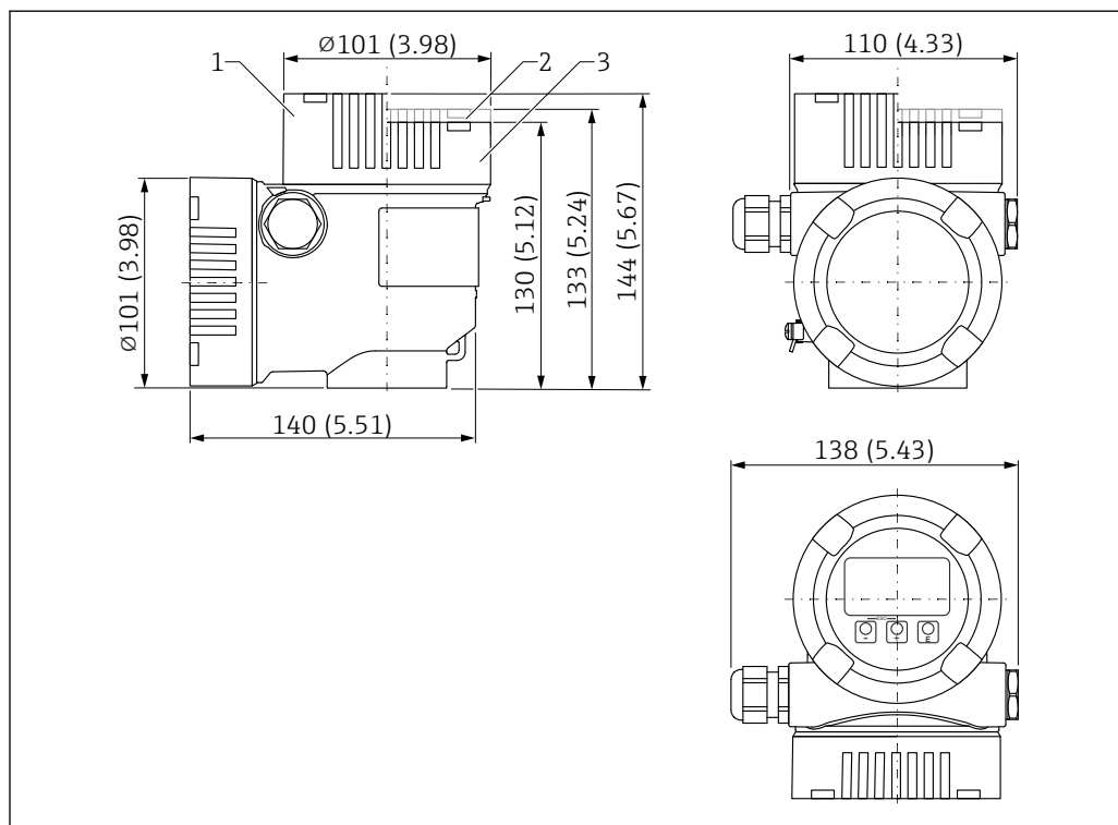
41 Размеры корпуса с двумя отсеками, L-образная форма. Единица измерения мм (дюйм)
