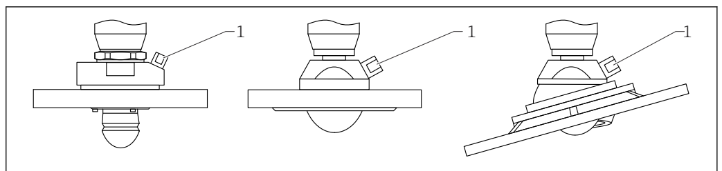
10 Антенна с переходником для подачи продувочного воздуха
