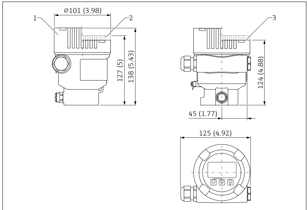
38 Размеры алюминиевого корпуса с одним отсеком. Единица измерения мм (дюйм)
