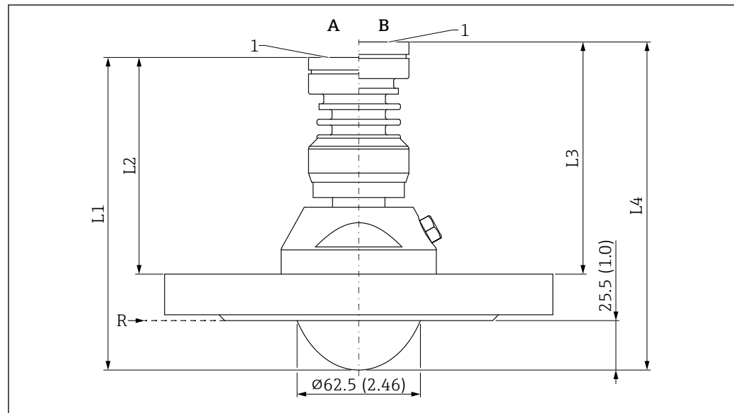
52 Размеры монтируемой заподлицо антенны, плакированной материалом PTFE, 80 мм (3 дюйм), со стандартным фланцем и соединением для продувочного воздуха. Единица измерения мм (дюйм)
