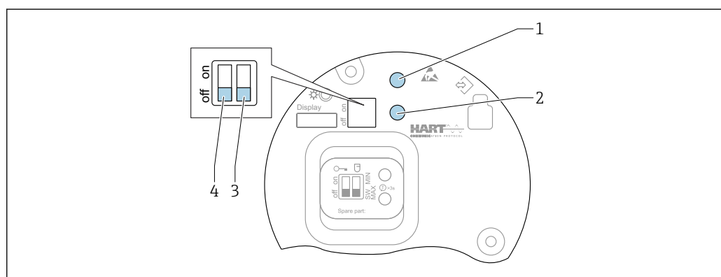
67 Кнопки управления и DIP-переключатели на электронной вставке HART
