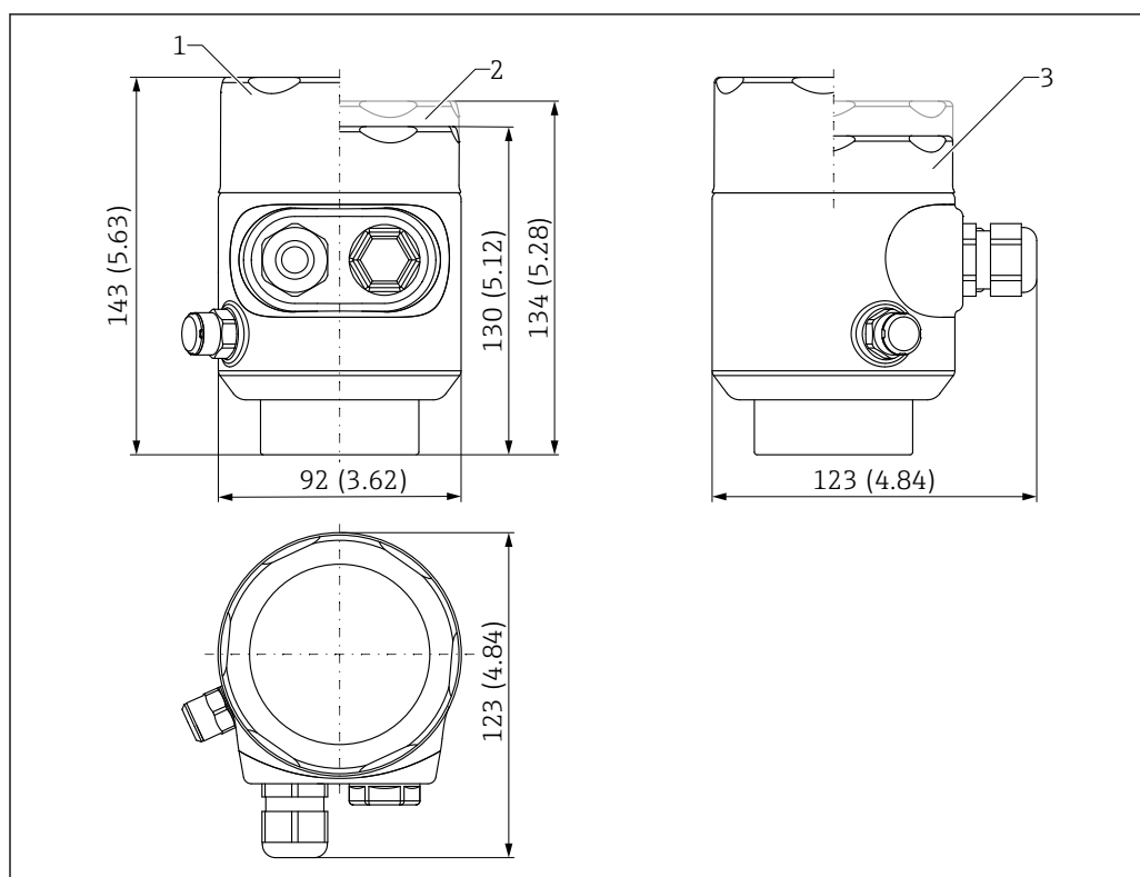
▣ 39 Размеры гигиенического корпуса с одним отсеком 316L. Единица измерения мм (дюйм)
