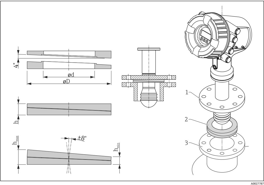
图 23 可调角度密封圈用于调节天线位置，角度调节范围为±8°
