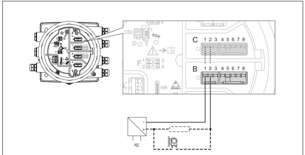
图 7 无源输入或无源输出：使用接线端子 1 和 2
