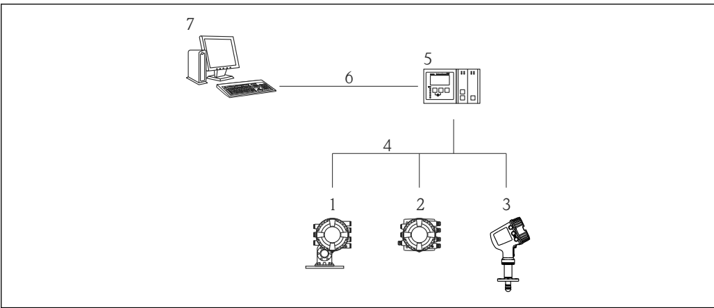
19 储罐计量仪表的远程操作
