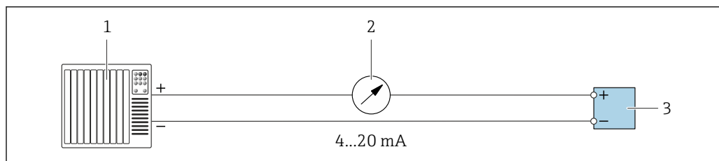
13 Przykład podłączenia dla wyjścia prądowego 4...20 mA (aktywnego)
