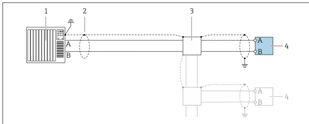
12 Przykład podłączenia dla wersji Modbus RS485, strefa niezagrożona wybuchem i Strefa 2; Klasa I, Div. 2
