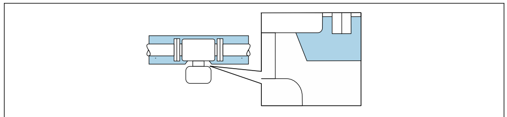
7 Izolacja termiczna rurociągu i szyjka wydłużona nieosłonięta
