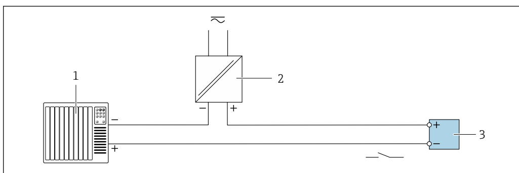
16 Przykład podłączenia wyjścia dwustanowego (pasywnego)
