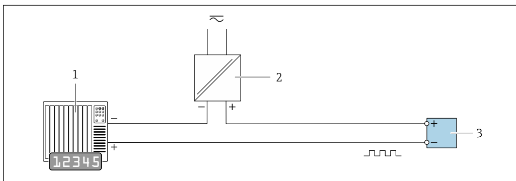
15 Przykład podłączenia dla wyjścia impulsowego/częstotliwościowego (pasywnego)
