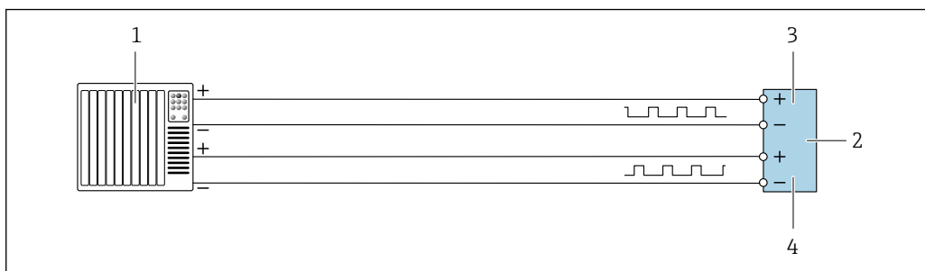
17 Przykład podłączenia dla podwójnego wyjścia impulsowego (aktywnego)
