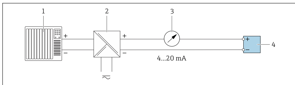
14 Przykład podłączenia dla wyjścia prądowego 4...20 mA (pasywnego)
