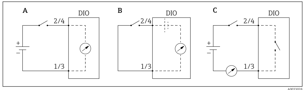
49 Modes de fonctionnement du module Digital I/O
