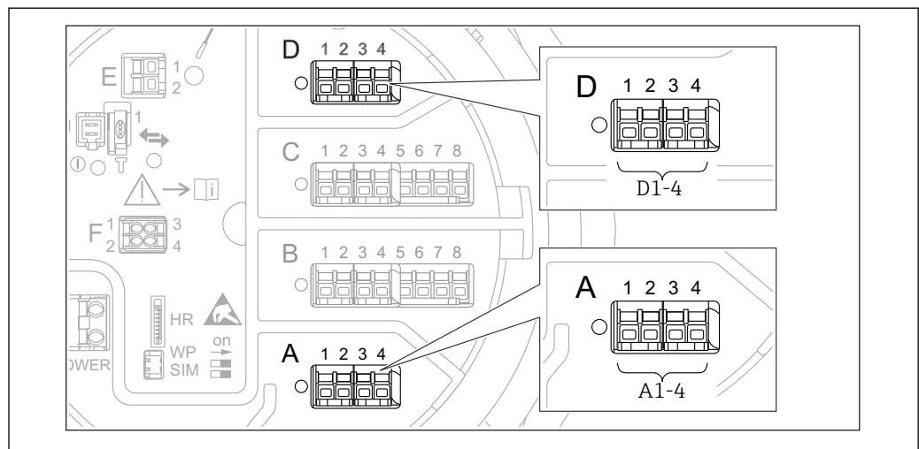
41 Emplacements possibles des modules WM550 (exemples) ; selon la version d'appareil, ces modules peuvent également se trouver dans le slot B ou C → 21.
