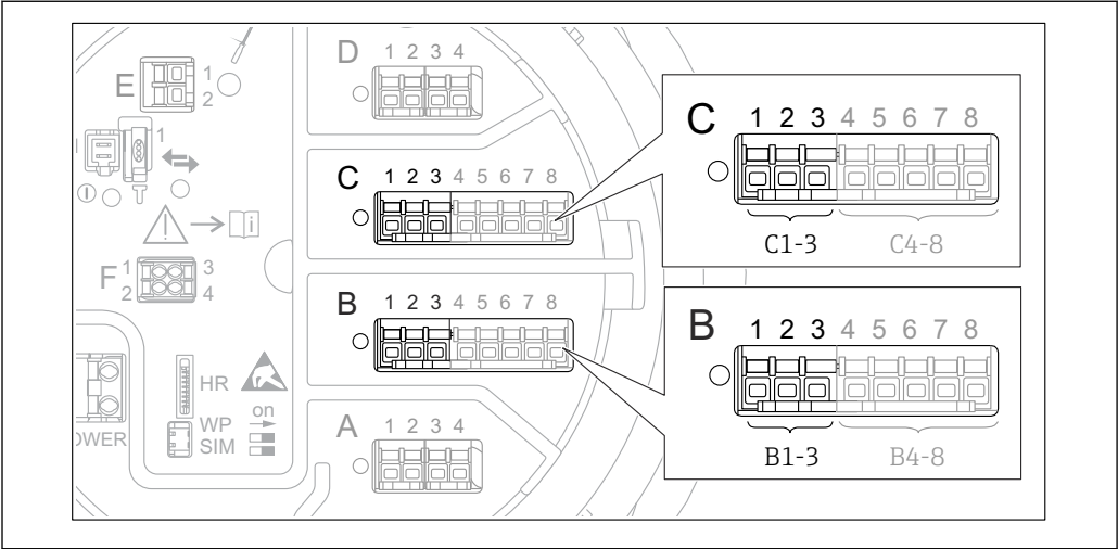
47 Bornes pour le sous-menu "Analog I/O" ("B1-3" ou "C1-3", respectivement)
