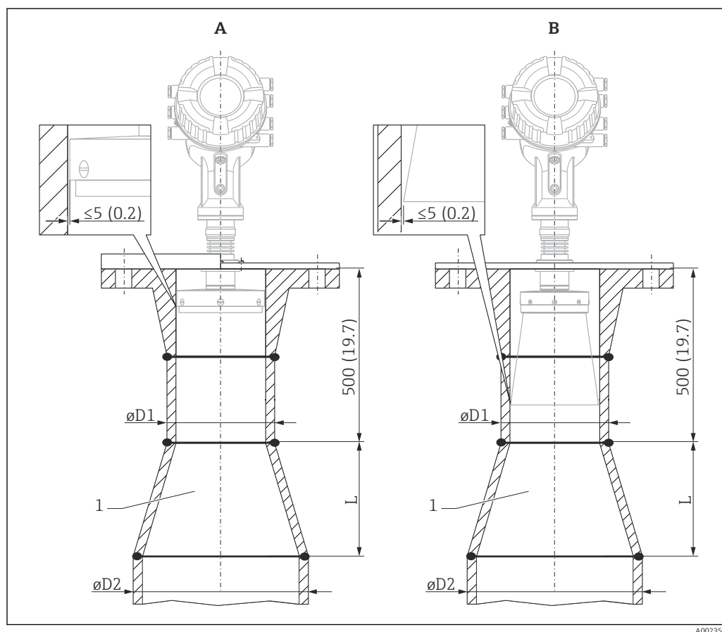
3 Montage du NMR84 dans des tubes de mesure avec un diamètre plus grand
