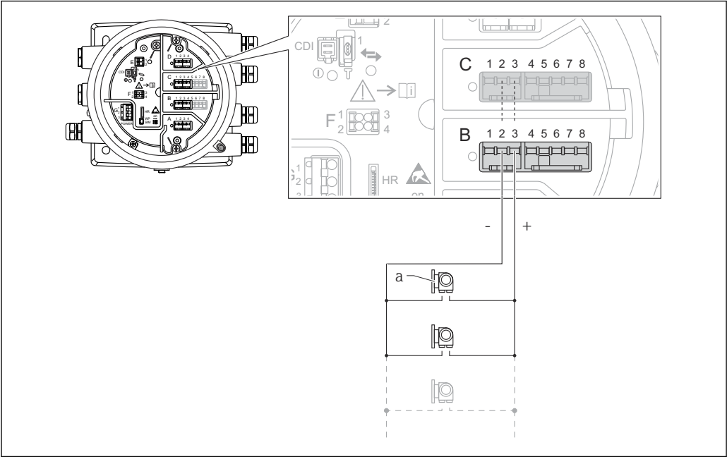
13 Utilisation active du module Analog I/O en mode maître HART
