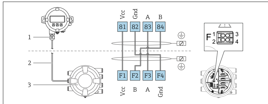
6 Raccordement du module d'affichage et de configuration séparé DKX001 à l'appareil de jaugeage de cuves (NMR8x, NMS8x ou NRF8x)
