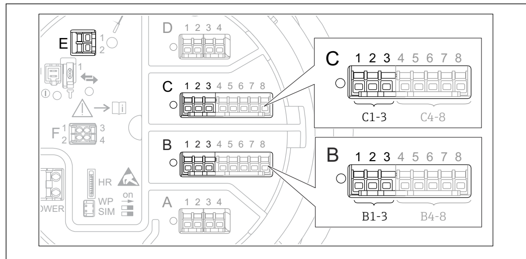
26 Bornes possibles pour les boucles HART
