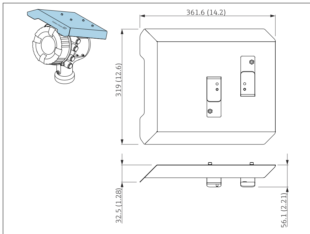
45 Capot de protection climatique ; dimensions en : mm (in)
