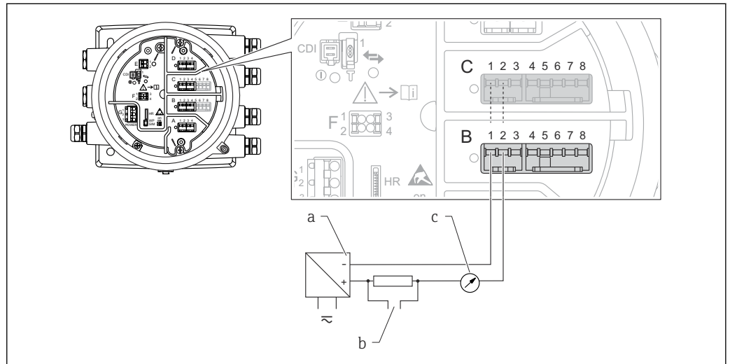
8 Utilisation passive du module Analog I/O en mode sortie
