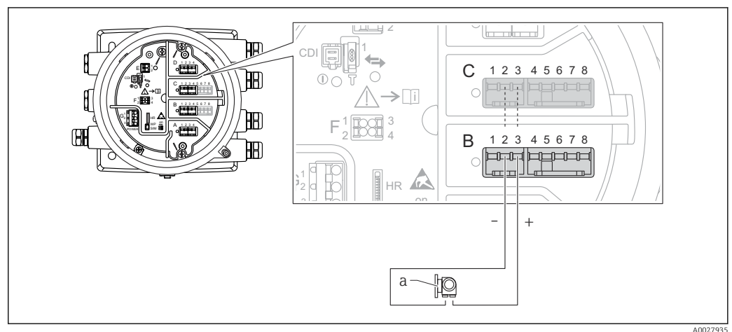
12 Utilisation active du module Analog I/O en mode entrée
