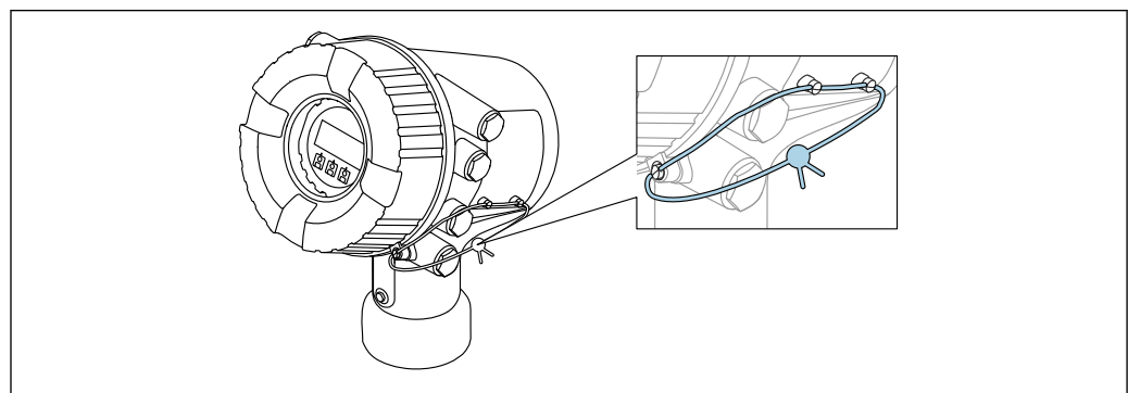
21 Plombage du cache du compartiment de raccordement
