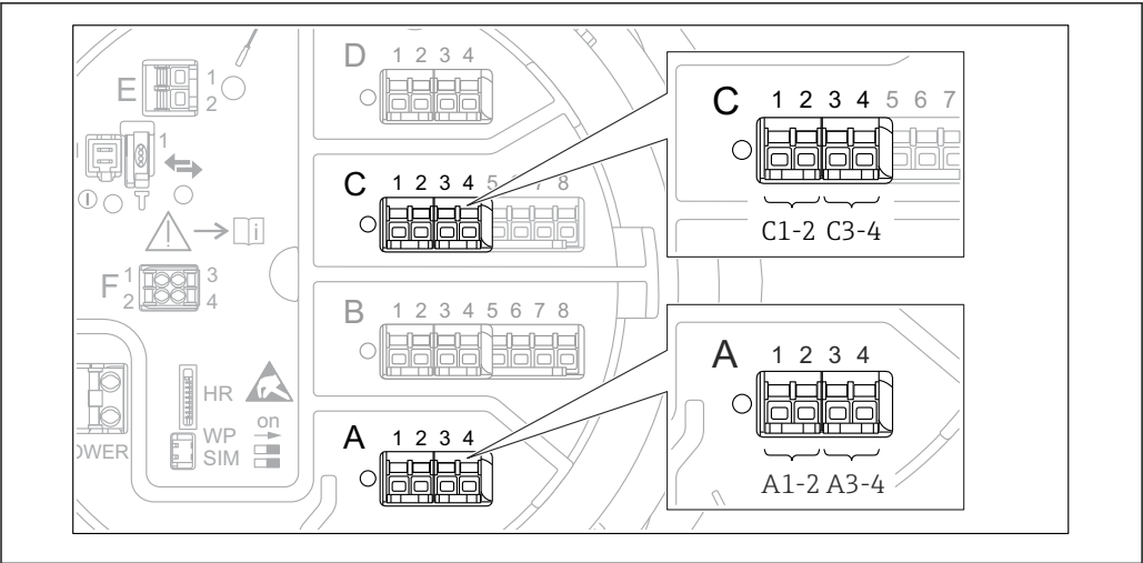
33 Emplacements possibles des modules Digital I/O (exemples) ; la référence de commande détermine le nombre et l'emplacement des modules d'entrée numériques → 21.
