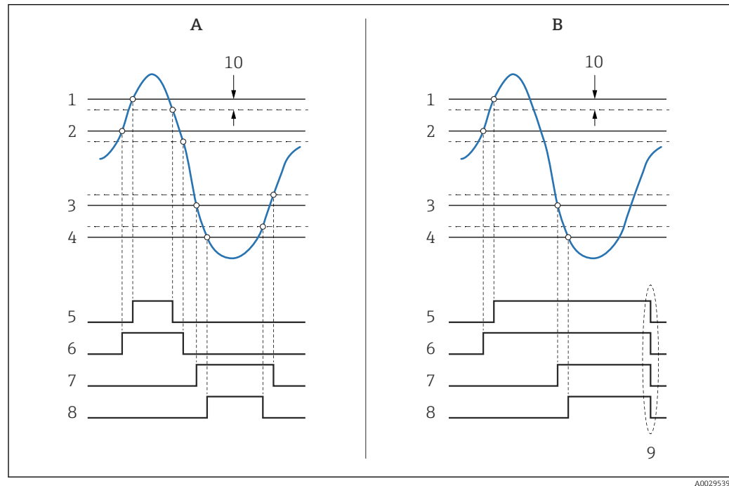
35 Principe de l'évaluation des limites
