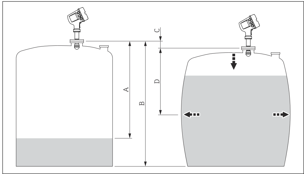
34 Correction de la déformation hydrostatique du réservoir (HyTD)
