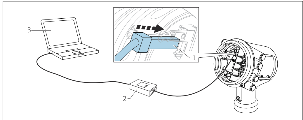
23 Configuration via l'interface service
