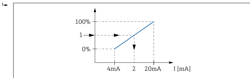
37 Mise à l'échelle de la variable de cuve en fonction du courant de sortie
