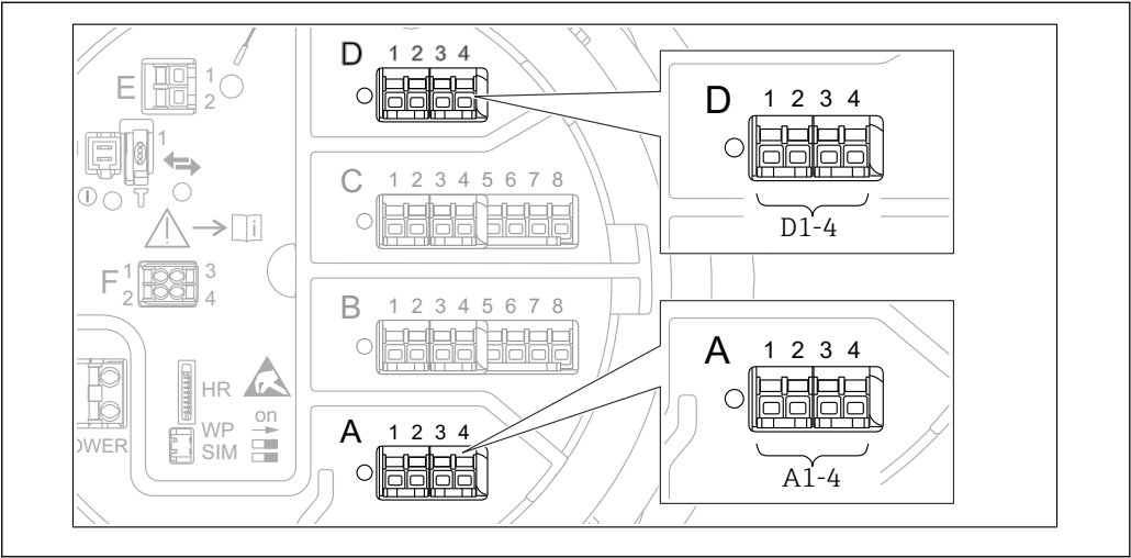
51 Désignation des modules "Modbus", "V1" ou "WM550" (exemples) ; selon la version d'appareil, ces modules peuvent également se trouver dans les slots B ou C.
