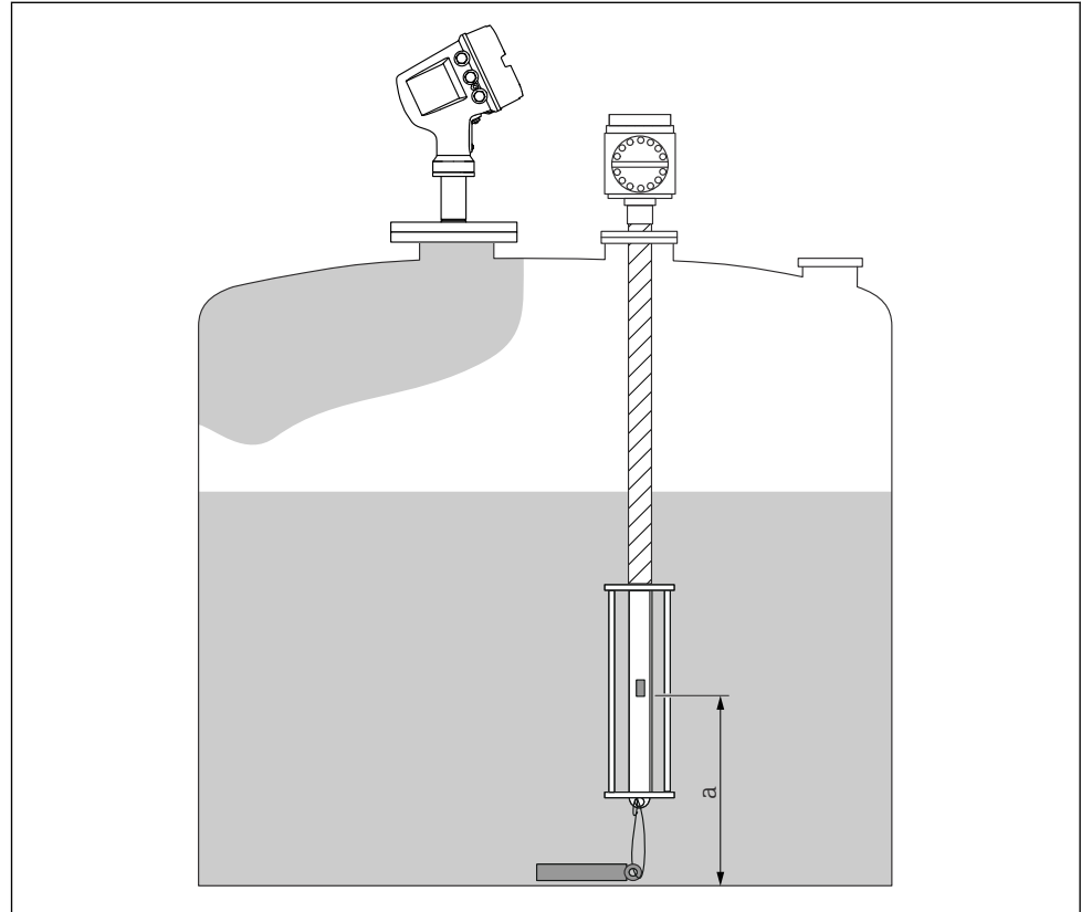
27 Prothermo NMT53x : position de l'élément de température du fond
