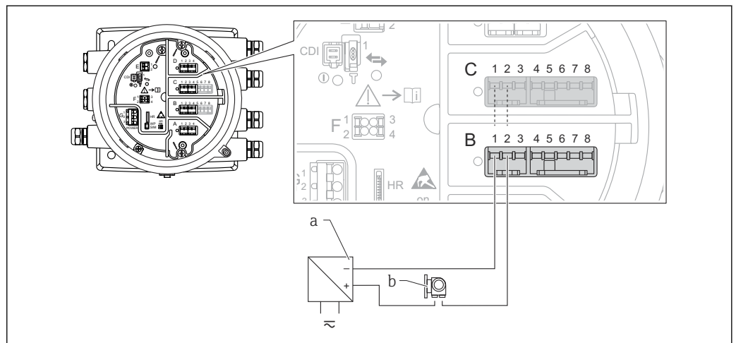
9 Utilisation passive du module Analog I/O en mode entrée
