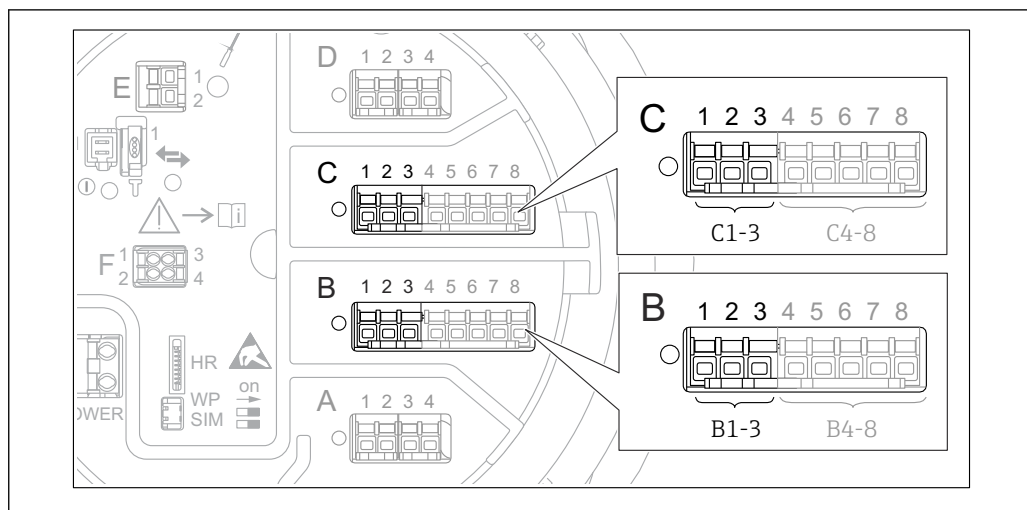
36 Emplacements possibles des modules Analog I/O, qui peuvent être utilisés comme sortie 4-20 mA. La référence de commande de l'appareil détermine le module réellement présent → 21.
