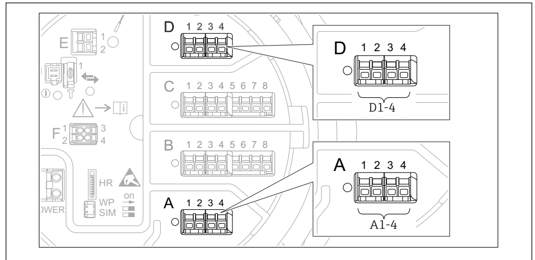
39 Emplacements possibles des modules Modbus (exemples) ; selon la version d'appareil, ces modules peuvent également se trouver dans le slot B ou C → 21 .
