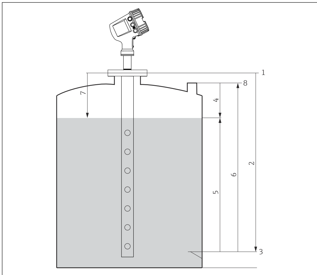
25 Termes relatifs à la mesure sur cuve par radar
