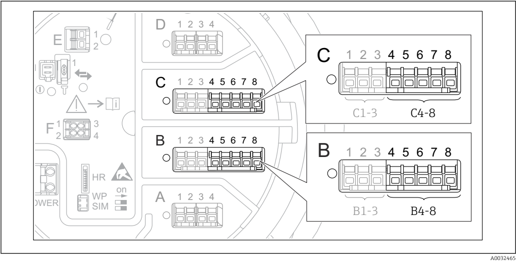
46 Bornes pour le sous-menu "Analog IP" ("B4-8" ou "C4-8", respectivement)
