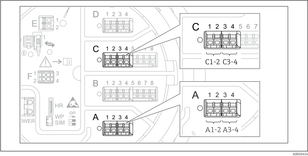
48 Désignation des entrées ou sorties numériques (exemples)
