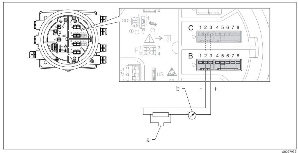
11 Utilisation active du module Analog I/O en mode sortie
