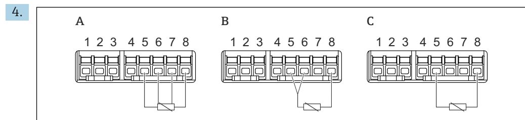
32 Types de raccordement de thermorésistances
