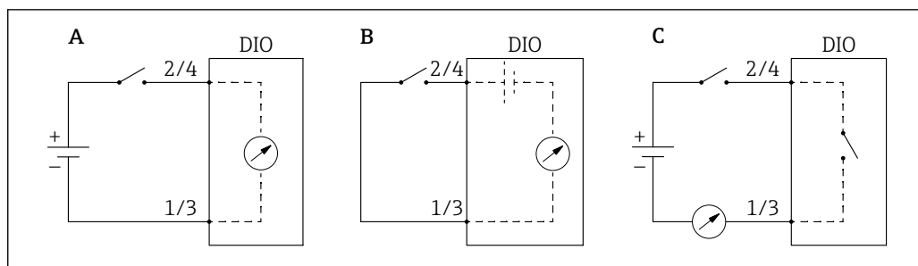
49 Режимы работы модуля цифрового ввода/вывода
