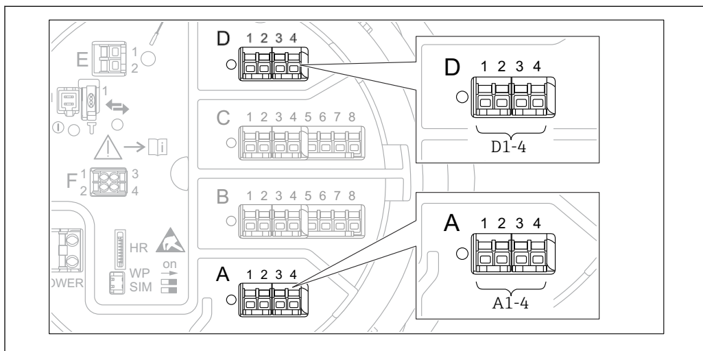
51 Обозначение модулей Modbus, V1 или WM550 (примеры). В зависимости от исполнения прибора эти модули могут находиться в гнезде B или C.
