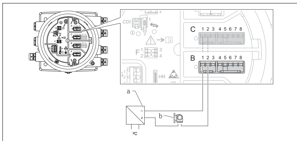
9 Использование модуля аналогового ввода/вывода в режиме пассивного входа
