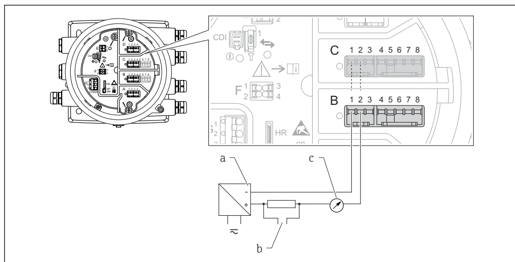
8 Использование модуля аналогового ввода/вывода в режиме пассивного выхода
