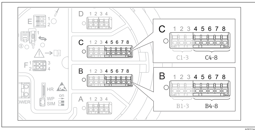
46 Контакты для подменю "Analog IP" (соответственно В4-8 или С4-8)
