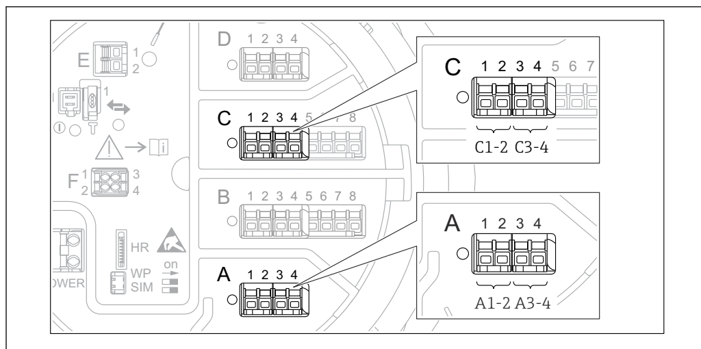
14 Обозначение цифровых входов и выходов (примеры)
