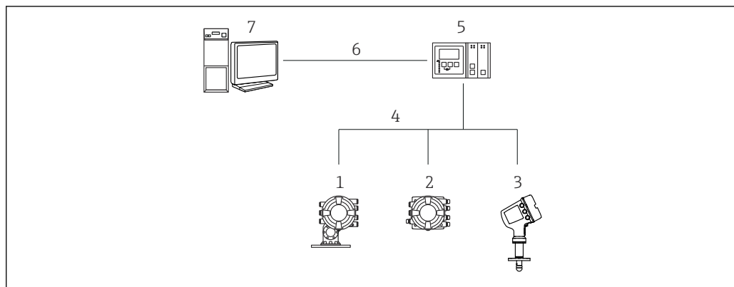
24 Подключение приборов для измерений в резервуарах к FieldCare посредством Tankvision Tank Scanner NXA820
