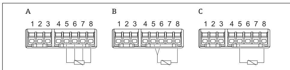
32 Типы подключений ТС
