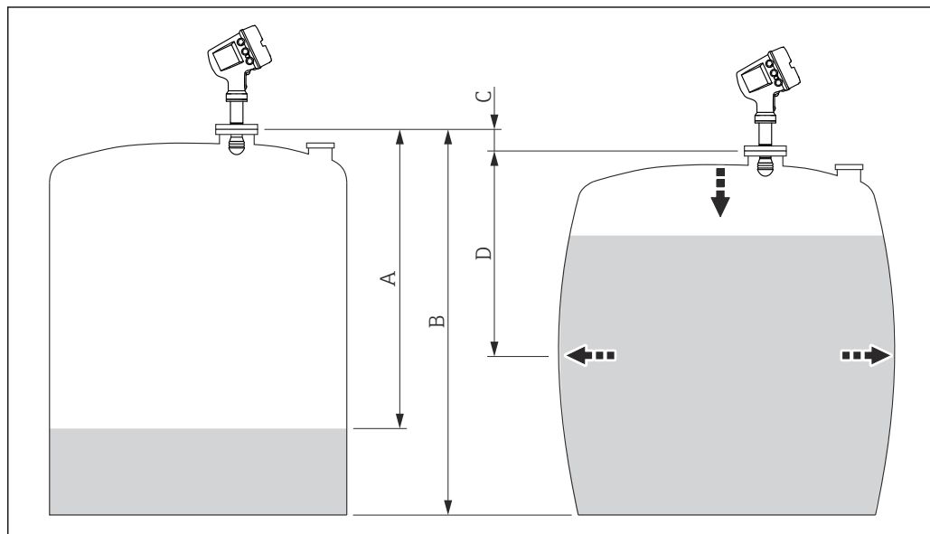
34 Корректировка гидростатической деформации резервуара (HyTD)
