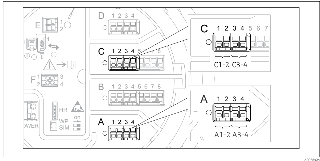
48 Обозначение цифровых входов и выходов (примеры)
