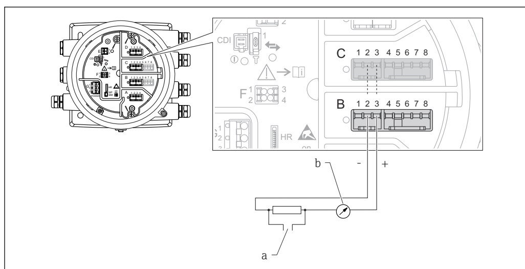
11 Использование модуля аналогового ввода/вывода в режиме активного выхода
