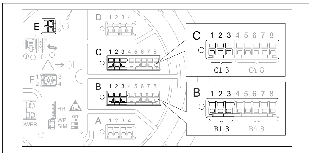
26 Доступные клеммы для цепей HART
