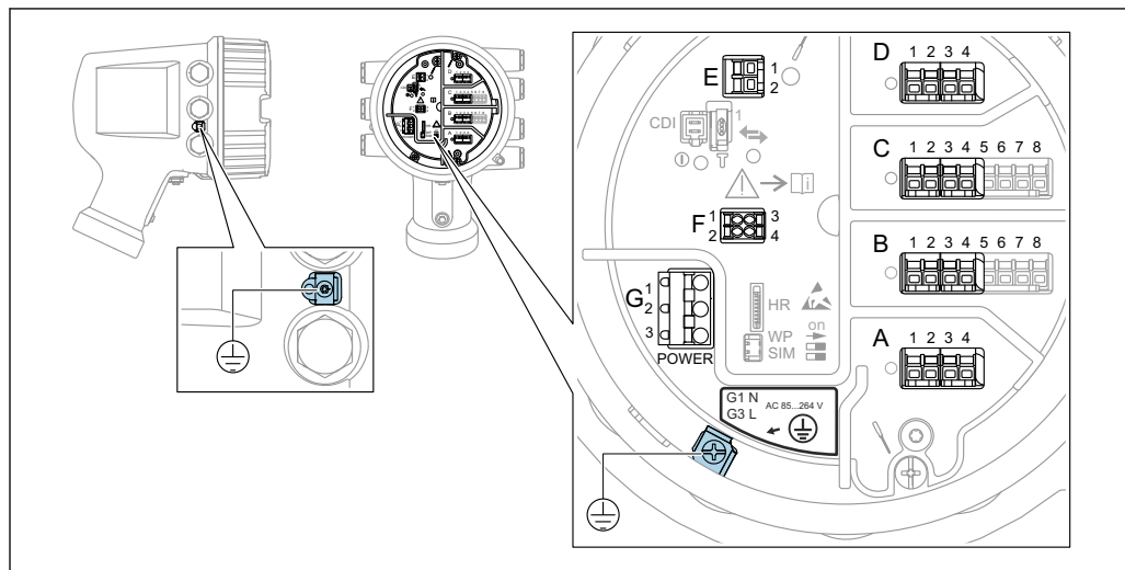
4 Клеммный отсек (типовой пример) и клеммы заземления
