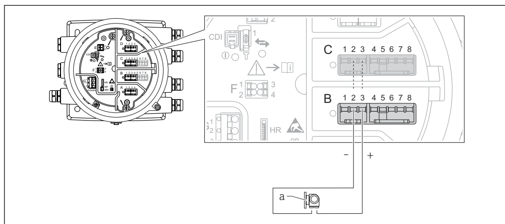
12 Использование модуля аналогового ввода/вывода в режиме активного входа
