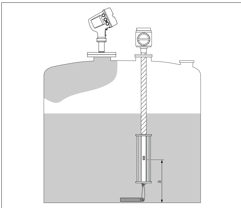
27 Prothermo NMT53x: позиция нижнего температурного элемента
