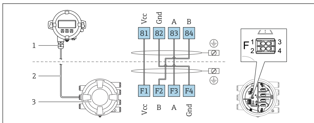
6 Подключение выносного модуля управления и дисплея DKX001 к прибору для измерения уровня в резервуарах (NMR8x, NMS8x или NRF8x)
