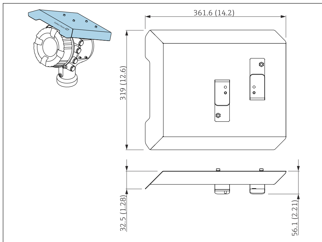
45 Защитный козырек от погодных явлений; размеры: мм (дюймы)
