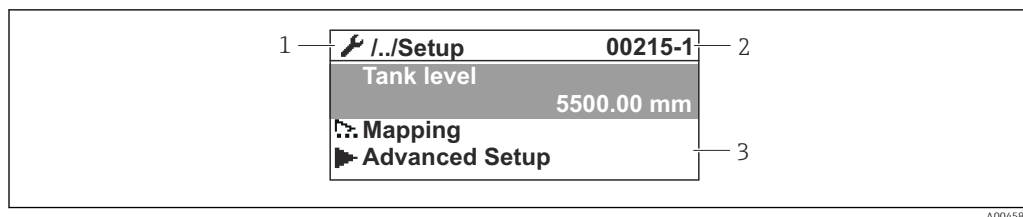
17 Окно навигации
