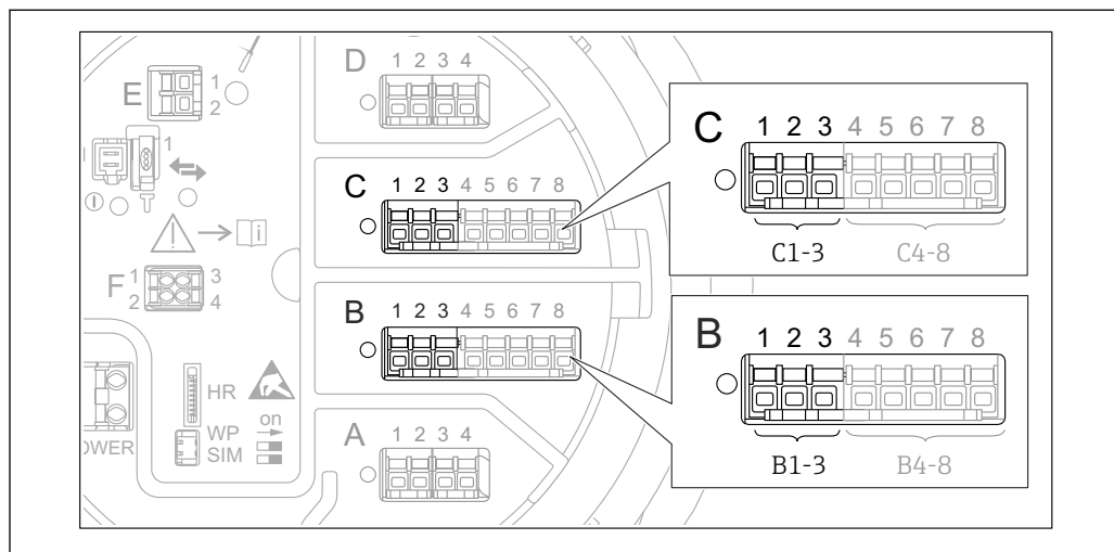
47 Контакты для подменю "Analog I/O" (соответственно B1-3 или C1-3)
