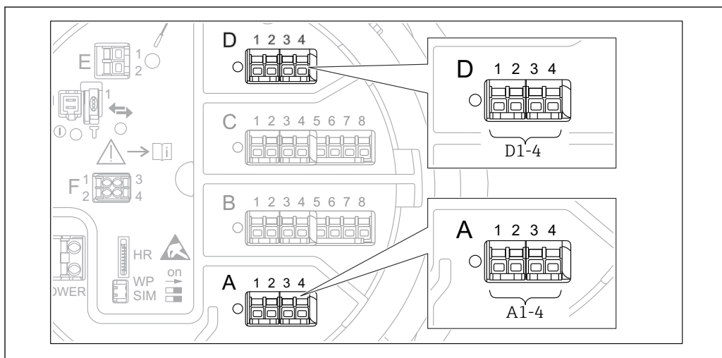
39 Возможное расположение модулей Modbus (примеры); в зависимости от исполнения прибора эти модули также могут находиться в гнезде B или C → 21.
