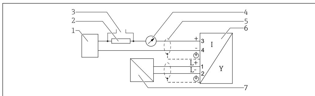
14 Schéma de principe 4 fils : 4-20 mA HART (10,4 ... 48 V DC )
