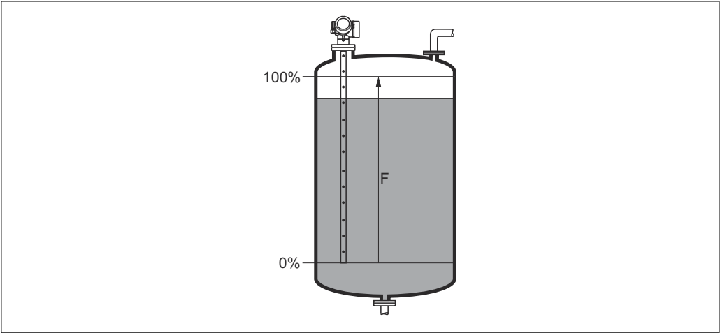
40 Plage de mesure (F) pour la mesure sur liquides
