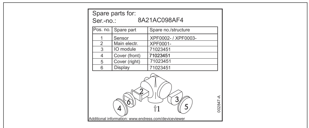
36 Exemple de plaque signalétique des pièces de rechange dans le couvercle du compartiment de raccordement
