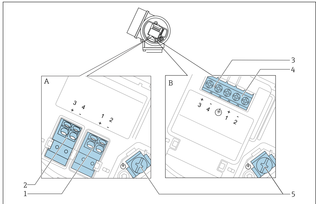
11 Occupation des bornes 2 fils : 4-20 mA HART, 4-20 mA
