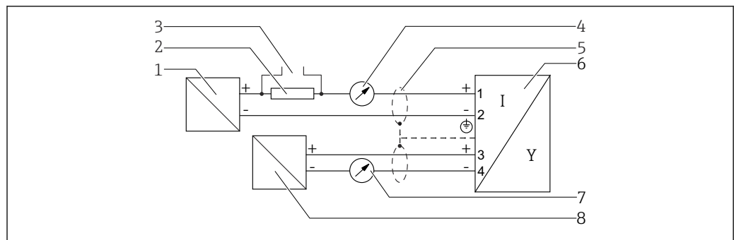
12 Schéma de principe 2 fils : 4-20 mA HART, 4-20 mA
