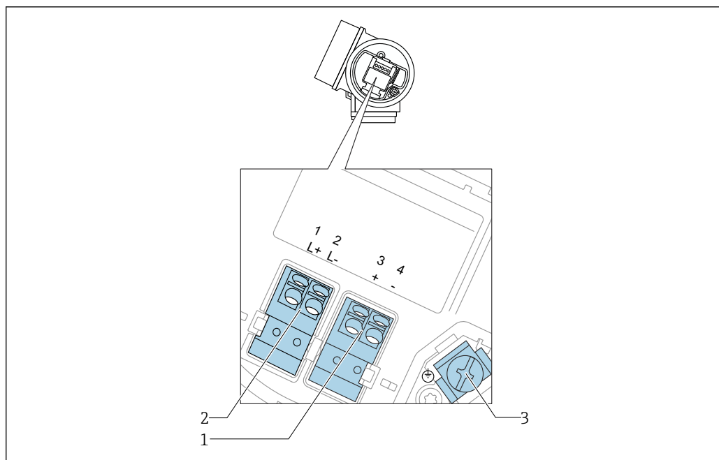
13 Occupation des bornes 4 fils : 4-20mA HART (10,4 ... 48 V DC )
