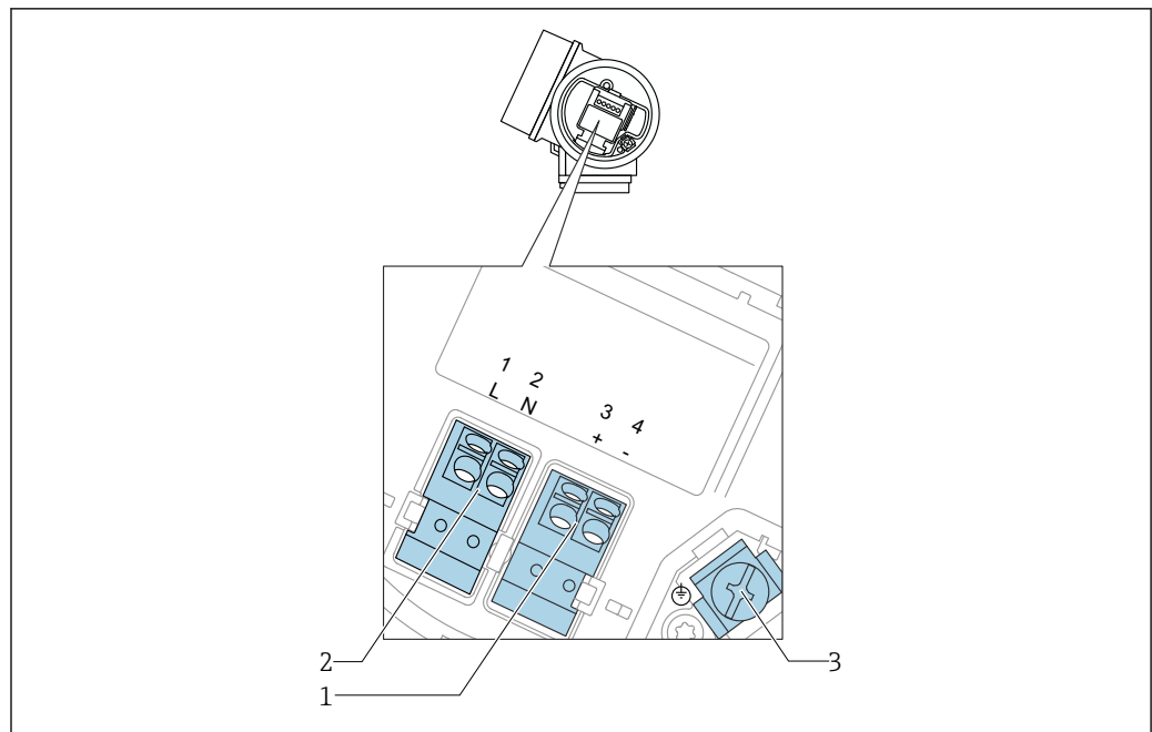
15 Occupation des bornes 4 fils : 4-20mA HART (90 ... 253 V AC )
