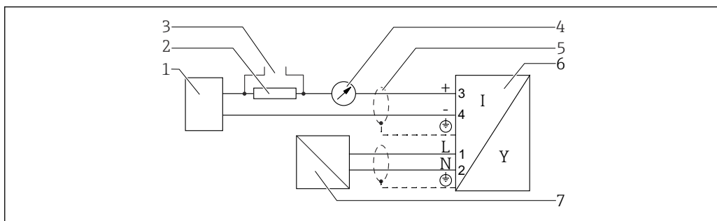
16 Schéma de principe 4 fils : 4-20 mA HART (90 ... 253 V AC )
