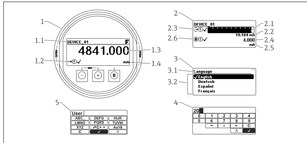
28 Apparence du module d'affichage et de configuration pour la configuration sur site
