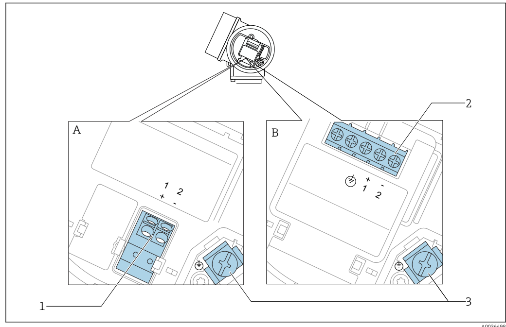
7 Occupation des bornes 2 fils : 4-20mA HART
