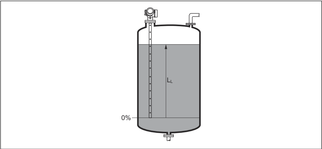
41 Niveau pour la mesure sur liquides
