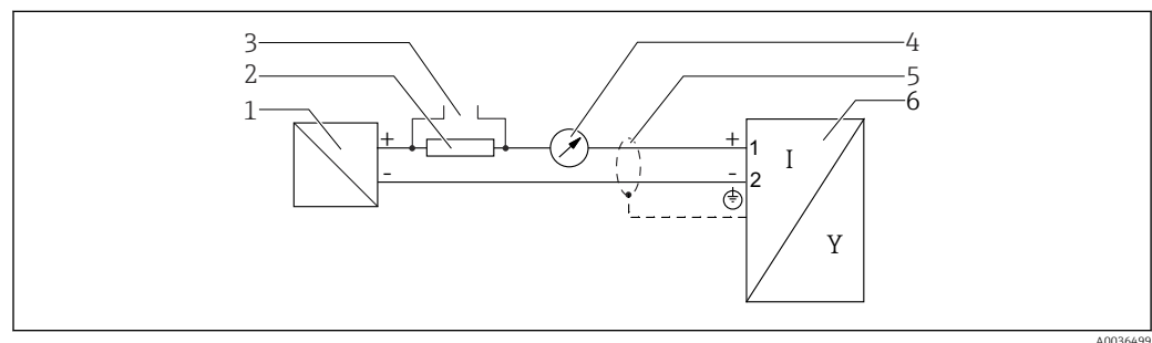
8 Schéma de principe 2 fils : 4-20 mA HART
