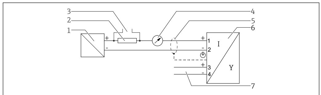
10 Schéma de principe 2 fils : 4-20 mA HART, sortie tout ou rien
