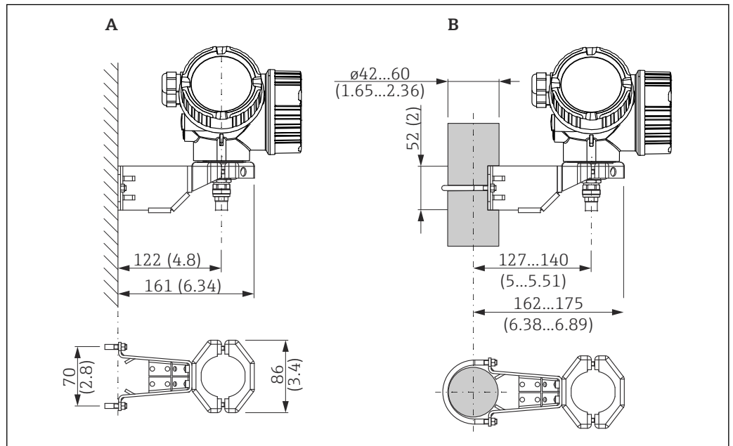
6 Montage du boîtier de l'électronique avec le support de montage. Unité de mesure mm (in)
