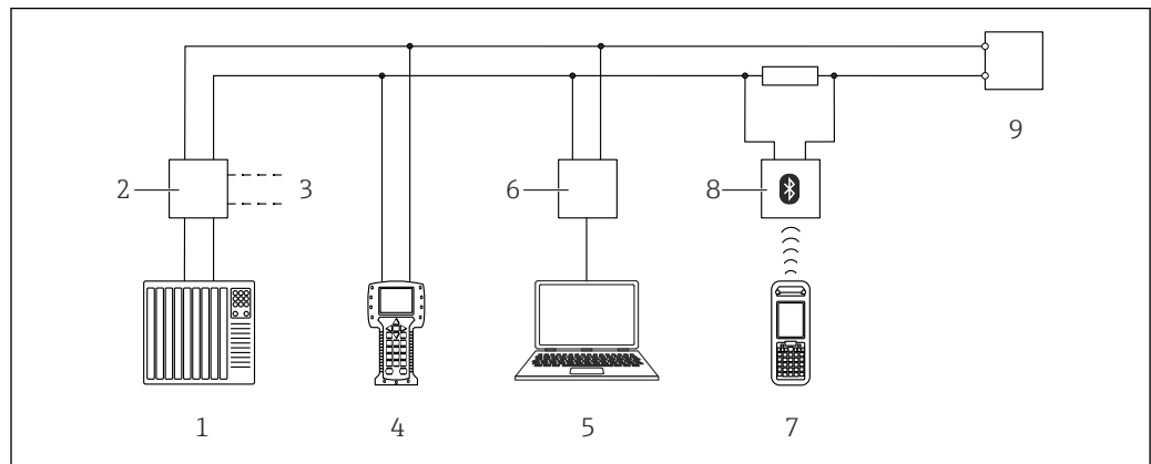
26 Options de configuration à distance via protocole HART
