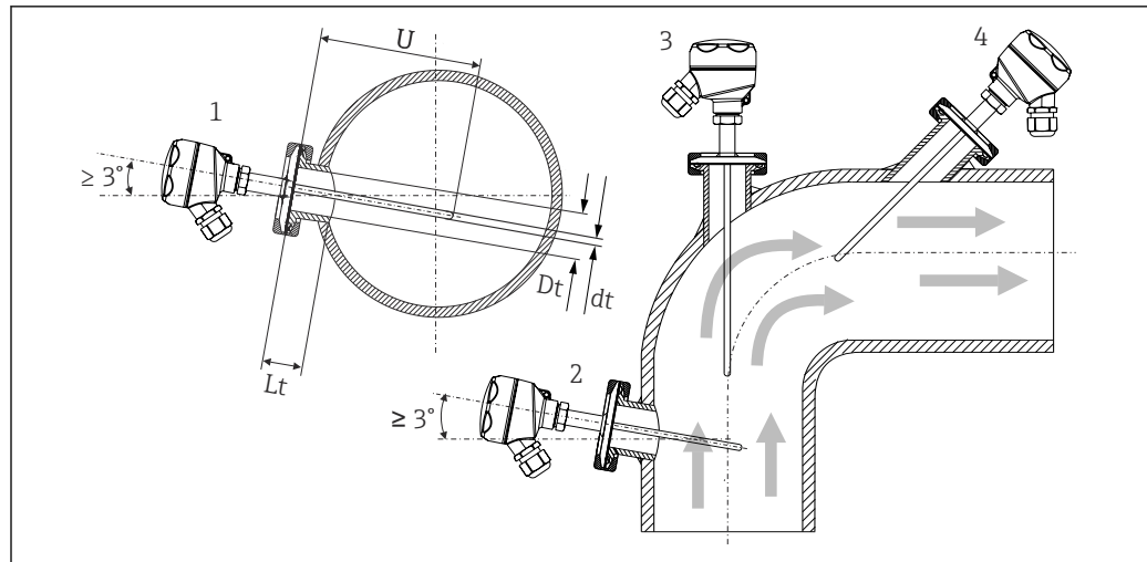
图 6 安装实例
