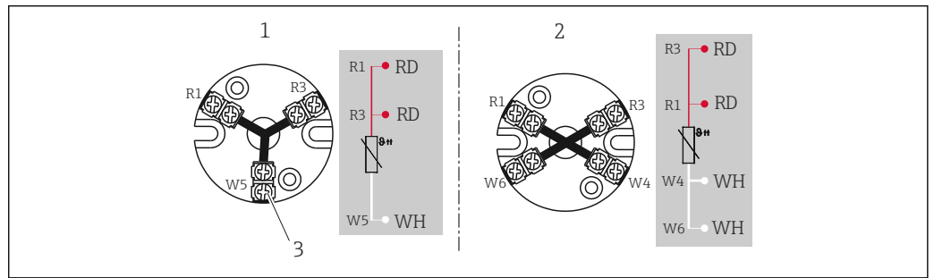
图 5 安装有接线端子块
