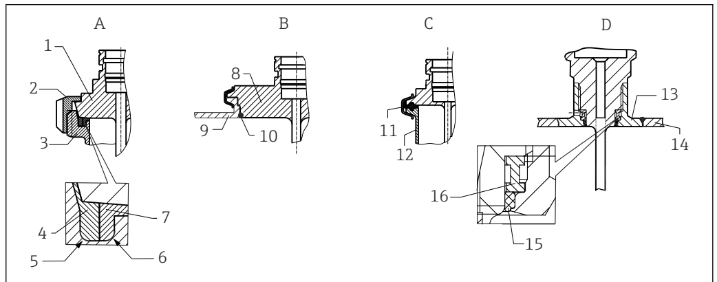
图 8 符合卫生要求安装の詳細安装说明 (取决于订购的型号)
