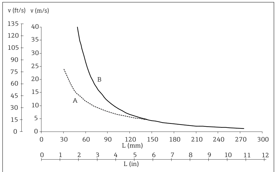
图 9 允许流速: 6 mm (1/4 in) 管径的保护套管
