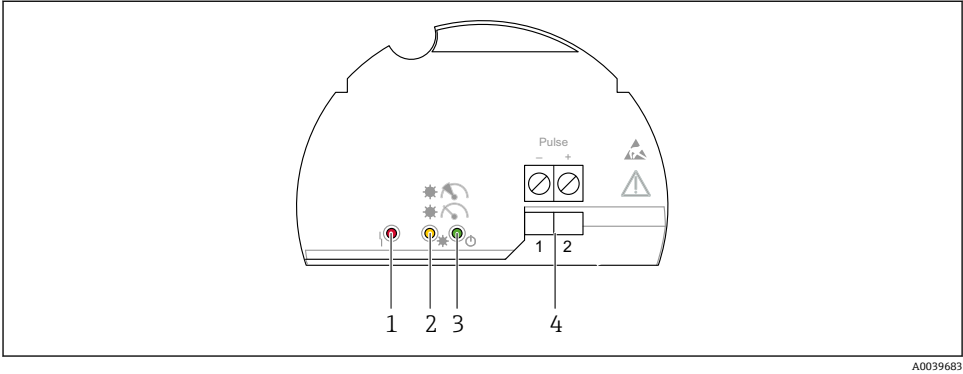
图 17 电子插件 FEL60D
