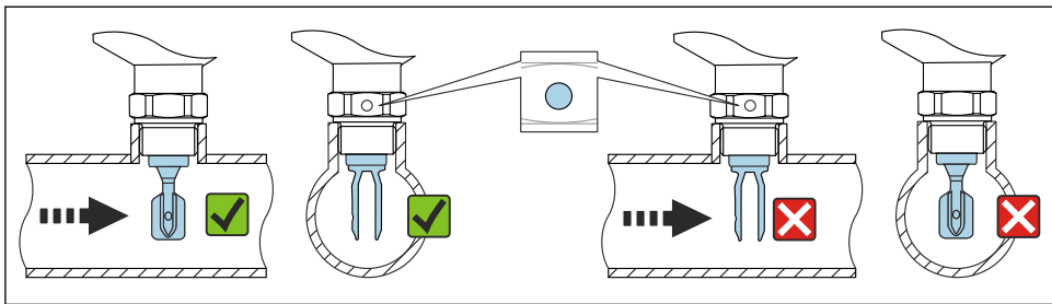
图 10 管道内安装（注意叉体安装位置和标记）
