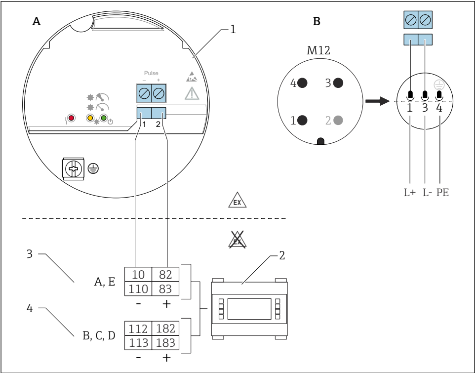
图 14 电子插件 FEL60D 和密度计算仪 FML621 的接线图
