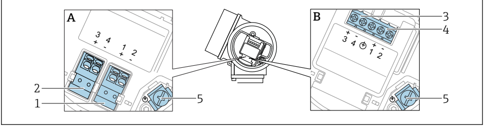
6 Terminal ataması, 2 telli: 4 ... 20 mA HART, 4 ... 20 mA
