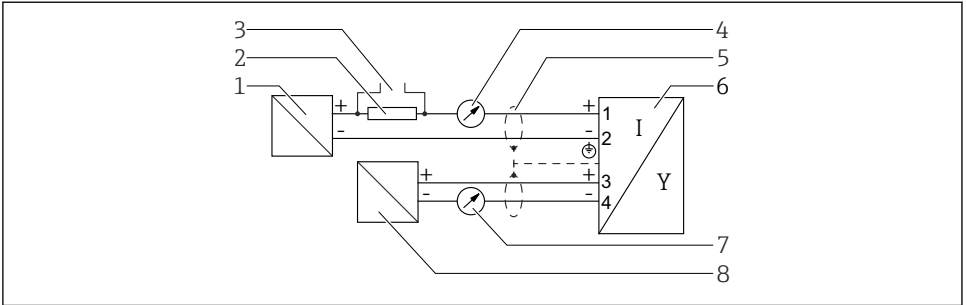
7 Blok şeması, 2 telli: 4 ... 20 mA HART, 4 ... 20 mA
