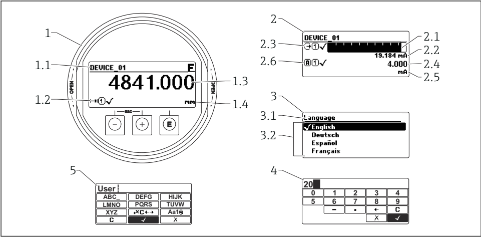
图 8 显示与操作单元的显示格式
