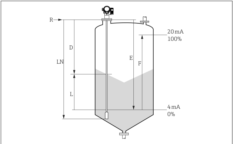
图 11 固体散料料位测量设置参数
