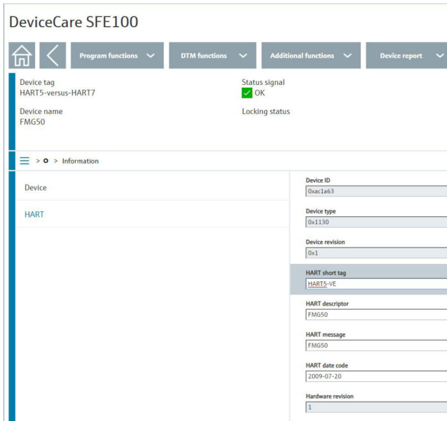
11 Darstellung des Device Tag und HART short tag in DeviceCare
