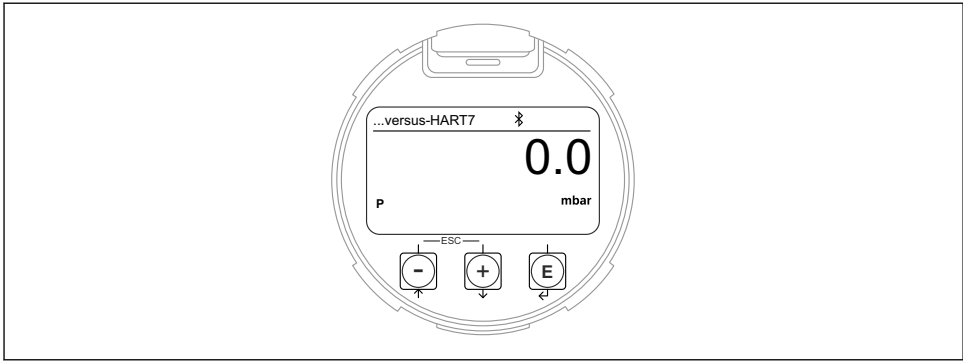
13 Darstellung des Device Tag in der Anzeige mit Produktstruktur, Merkmal "Anzeige; Bedienung", Option E "Grafische Anzeige mit Tasten", Option F "Grafische Anzeige mit Tasten + Bluetooth"
