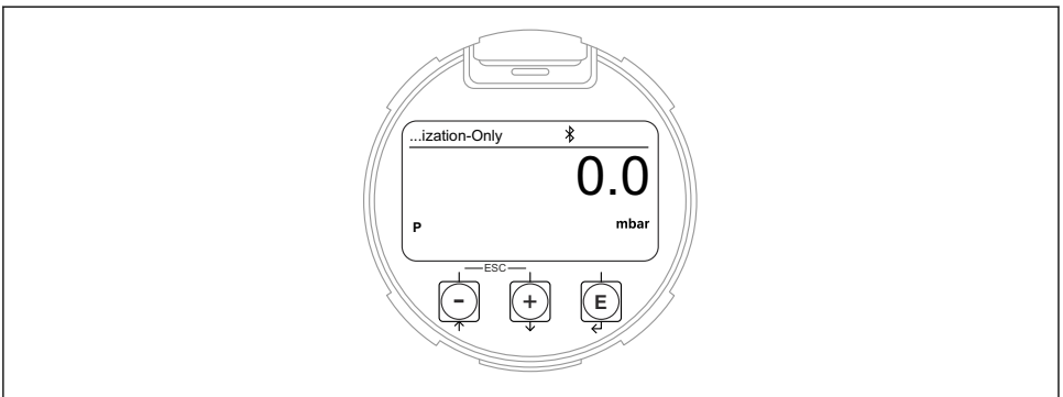
8 Darstellung des Device Tag in der Anzeige mit Produktstruktur, Merkmal "Anzeige; Bedienung", Option E "Grafische Anzeige mit Tasten", Option F "Grafische Anzeige mit Tasten + Bluetooth"
