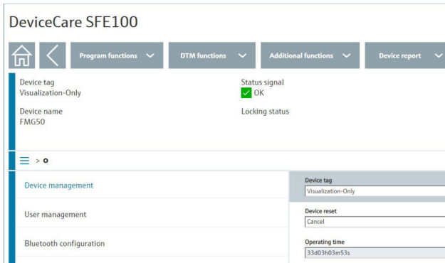
7 Darstellung des Device Tag in DeviceCare
