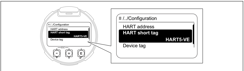
12 HART short tag im Bedienmenü der Anzeige mit Produktstruktur, Merkmal "Anzeige; Bedienung", Option E "Grafische Anzeige mit Tasten", Option F "Grafische Anzeige mit Tasten + Bluetooth"
