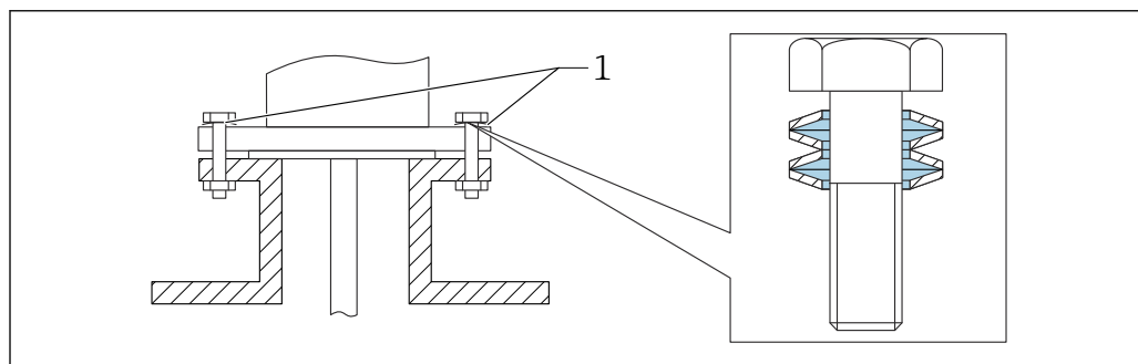
1 弹簧垫圈
