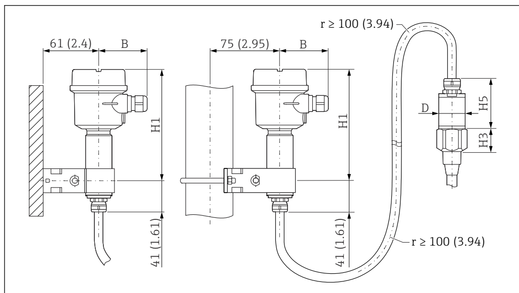
图 6 外壳端（墙装、管装）和传感器端。测量单位 mm (in)
