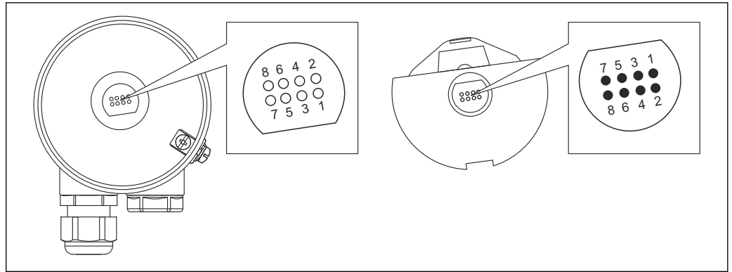
图 8 电子插件触点
