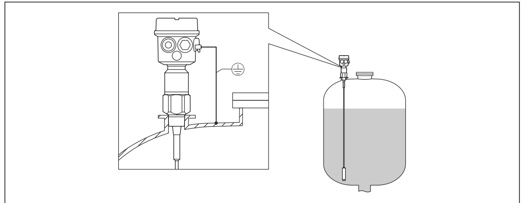
图 2 缆式探头
