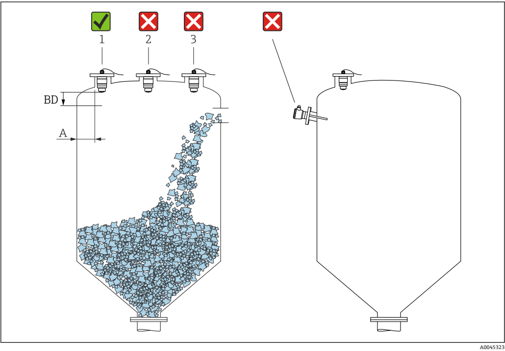
11 罐体上的安装位置
