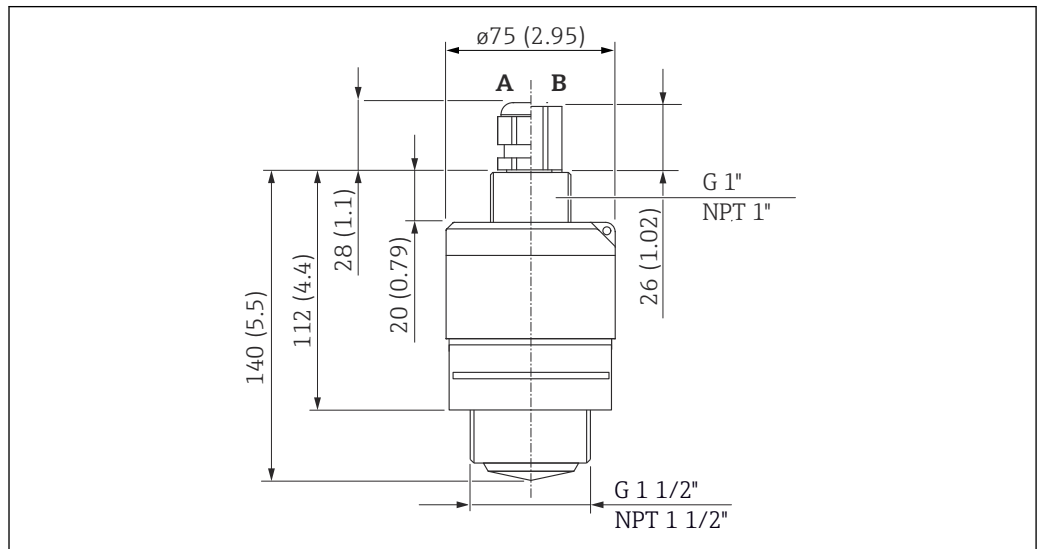
图 26 G 1-½" 或 MNPT 1-½" 螺纹过程连接的外形尺寸；单位：mm (in)
