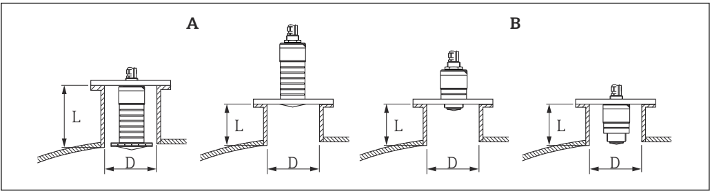
12 安装在安装短管中
