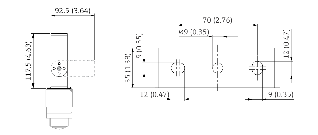
图 43 墙装架的外形尺寸；单位：mm (in)
