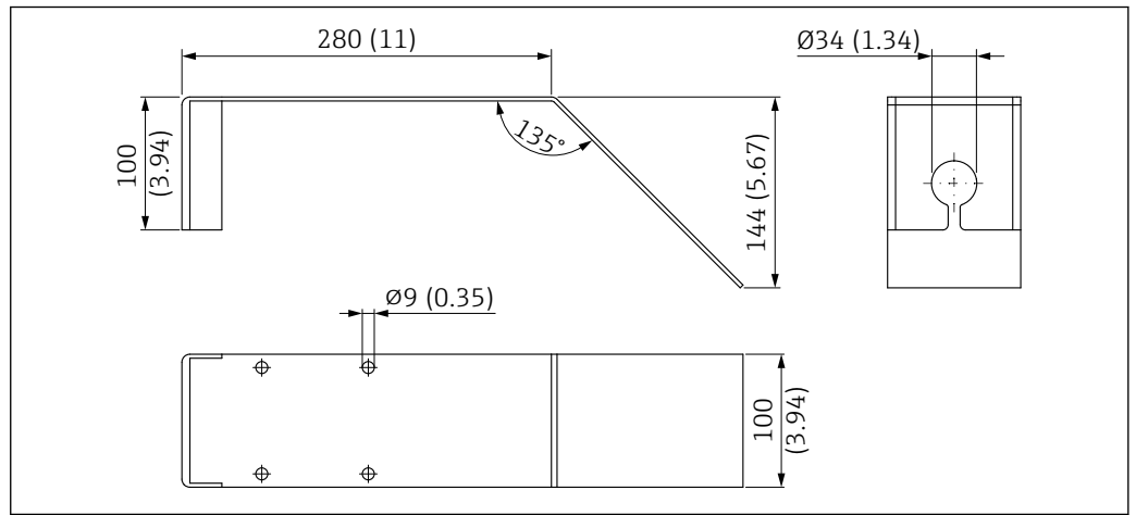
图 61 水平安装架的外形尺寸。测量单位 mm (in)
