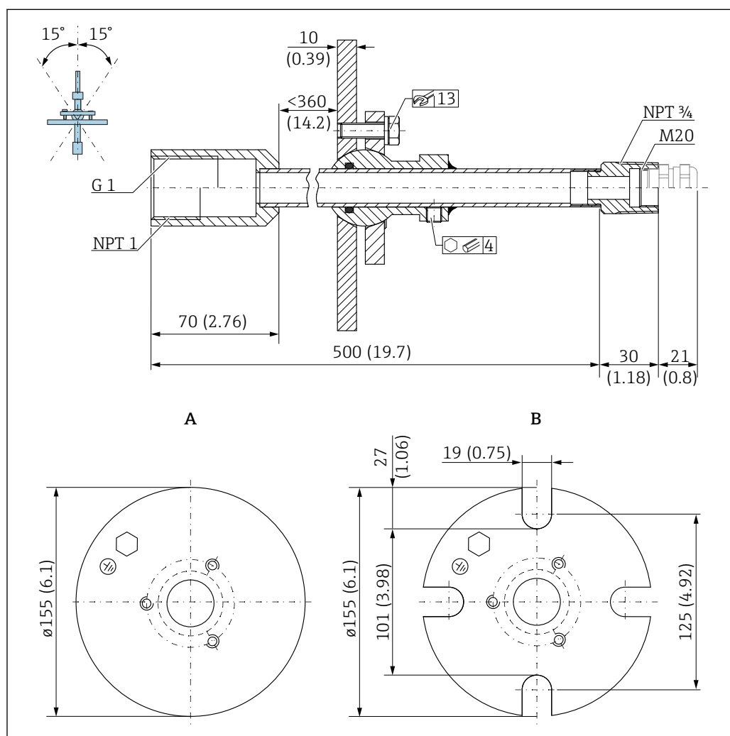
图 62 外形尺寸。测量单位 mm (in)
