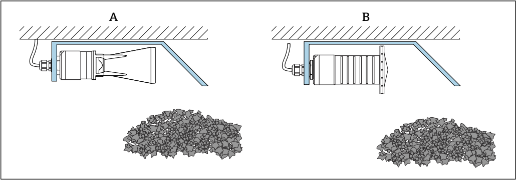
21 使用水平安装支架安装 A 40 mm (1.5 in) 口径天线，安装有防溢管（附件） B 80 mm (3 in) 口径天线，未安装防溢管
