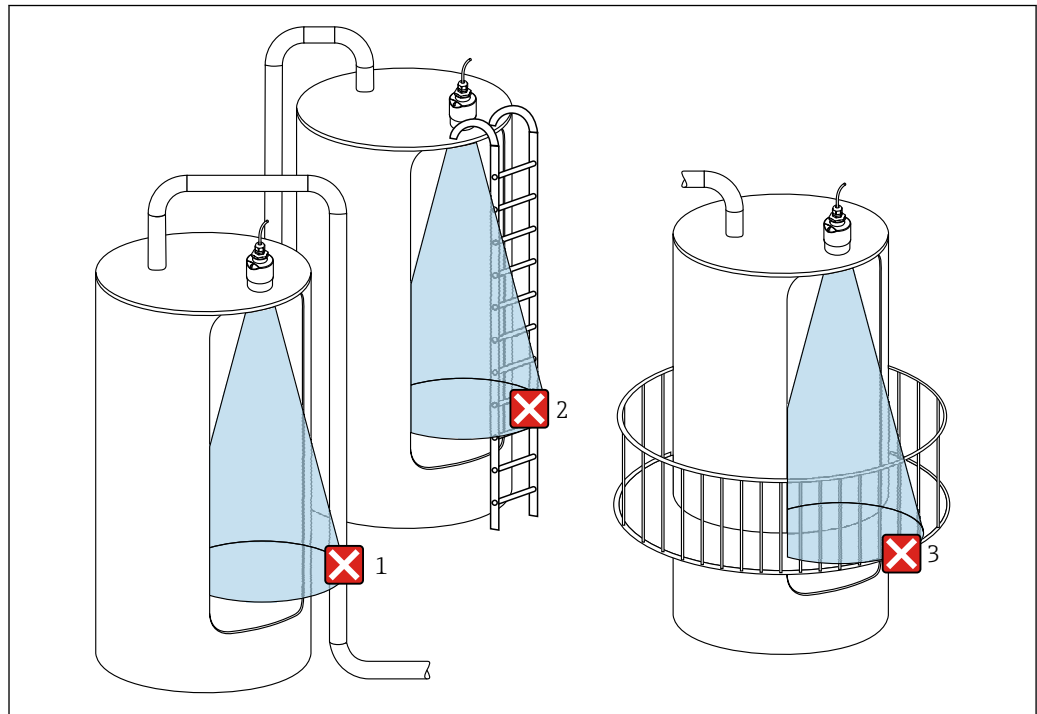
图 16 在外部装有金属干扰物的塑料罐中测量
