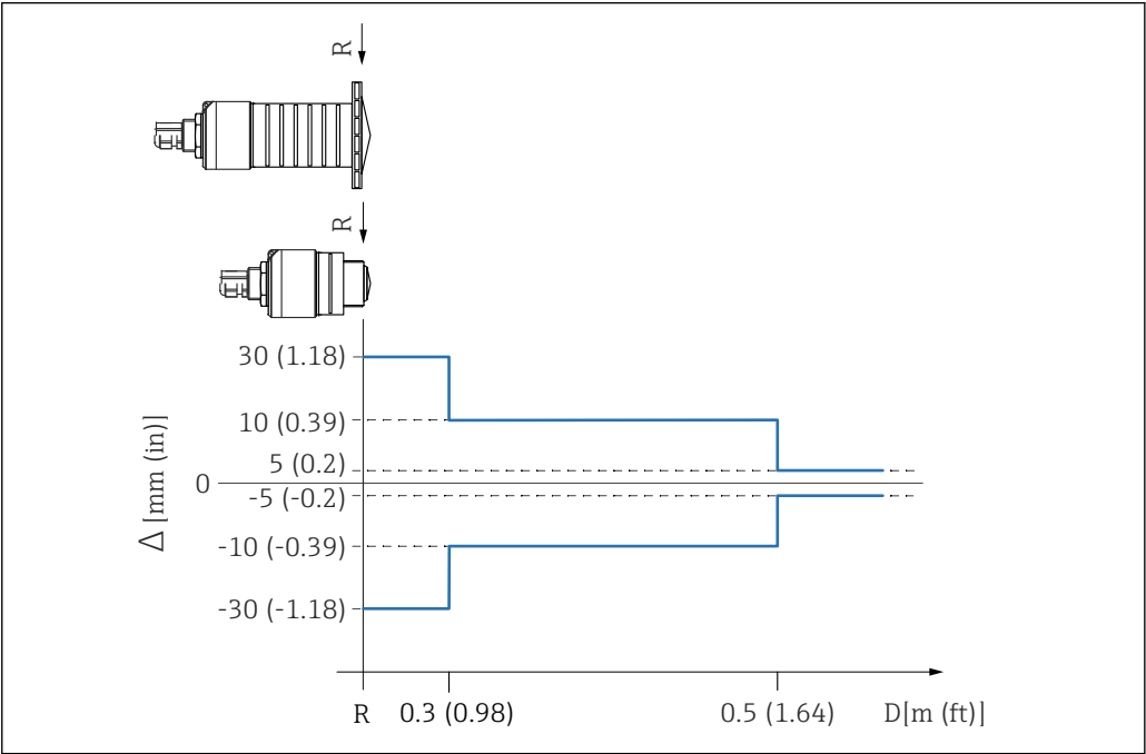
9 近距离测量时的最大测量误差 (以标准型仪表为例) Δ 最大测量误差 R 距离测量的参考点 D 距离天线参考点的间距
