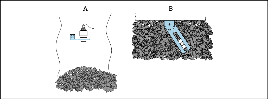
22 安装，可旋转和可调节 A 使用悬臂和安装架安装 B 可旋转和可调节悬臂（将设备对准待测介质）
