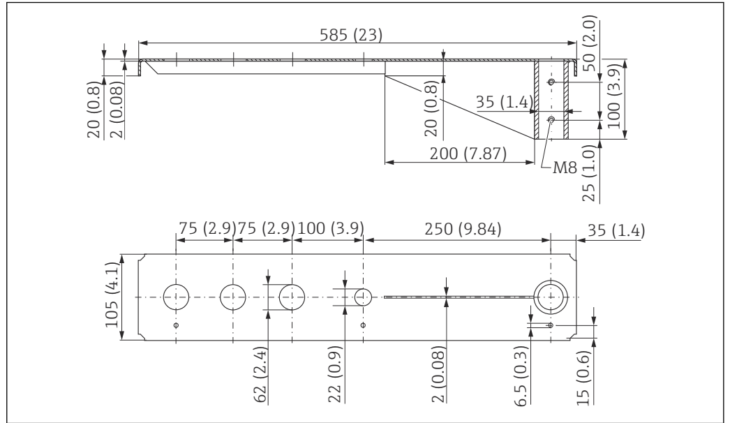
54 外形尺寸。测量单位 mm (in)
