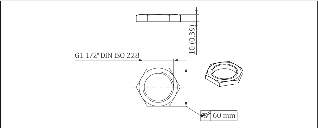
39 锁紧螺母的外形尺寸；单位：mm (in)
