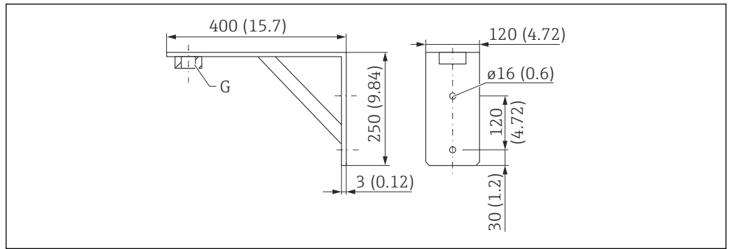
图 47 角撑架的外形尺寸。测量单位 mm (in)
