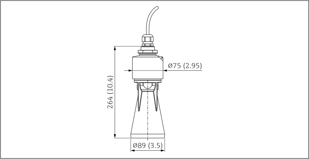
28 40 mm (1.5 in)口径天线的外形尺寸，安装有防溢管；单位：mm (in)
