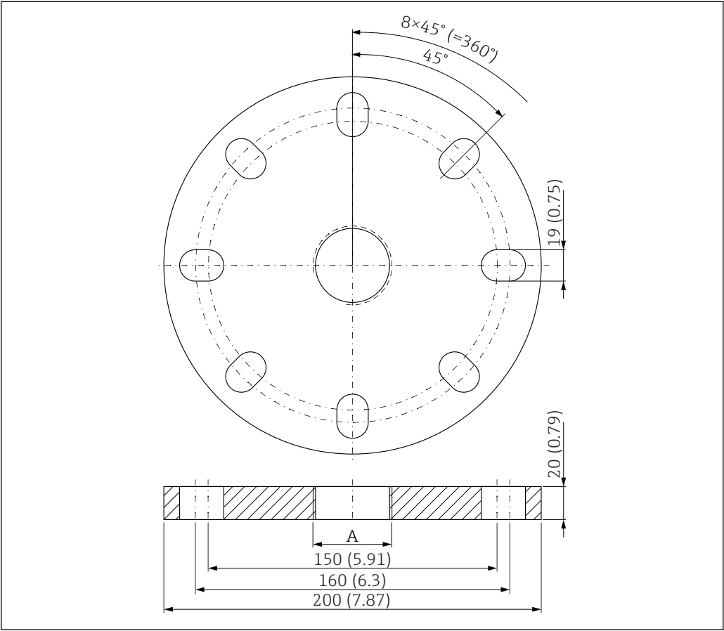
45 UNI 3"/DN80/80 法兰的外形尺寸; 单位: mm (in)
