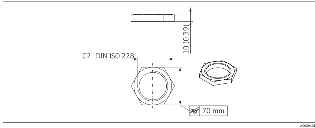
40 锁紧螺母的外形尺寸；单位：mm (in)
