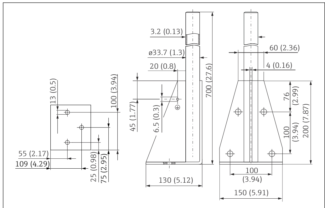
图 56 外形尺寸。测量单位 mm (in)
