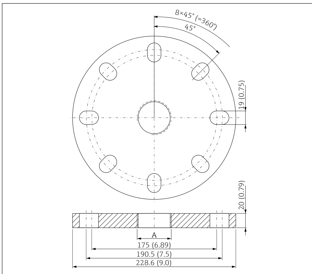
图 46 UNI 4"/DN100/100 法兰的外形尺寸; 单位: mm (in)
