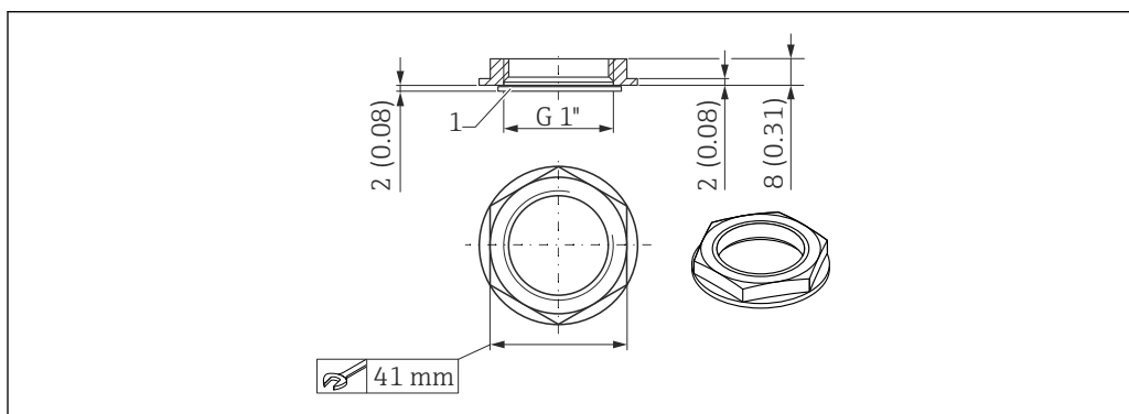
图 34 底部过程连接锁紧螺母的外形尺寸；单位：mm (in)
