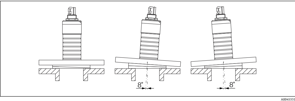
图 24 Micropilot FMR20，带可变角度法兰密封圈
