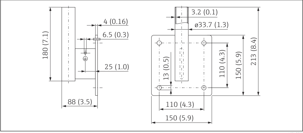
图 58 墙装架的外形尺寸。测量单位 mm (in)
