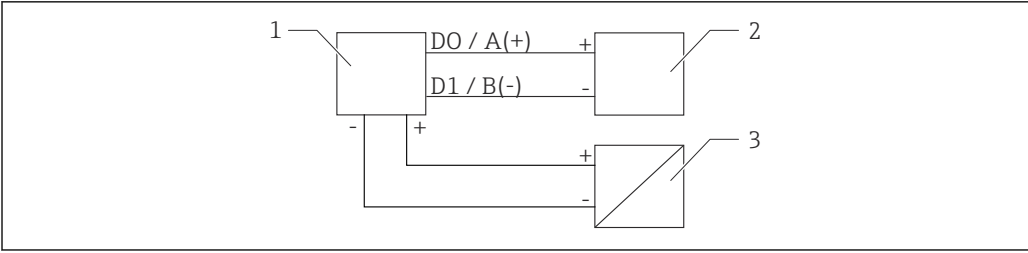
6 Modbus RS485 信号回路连接
