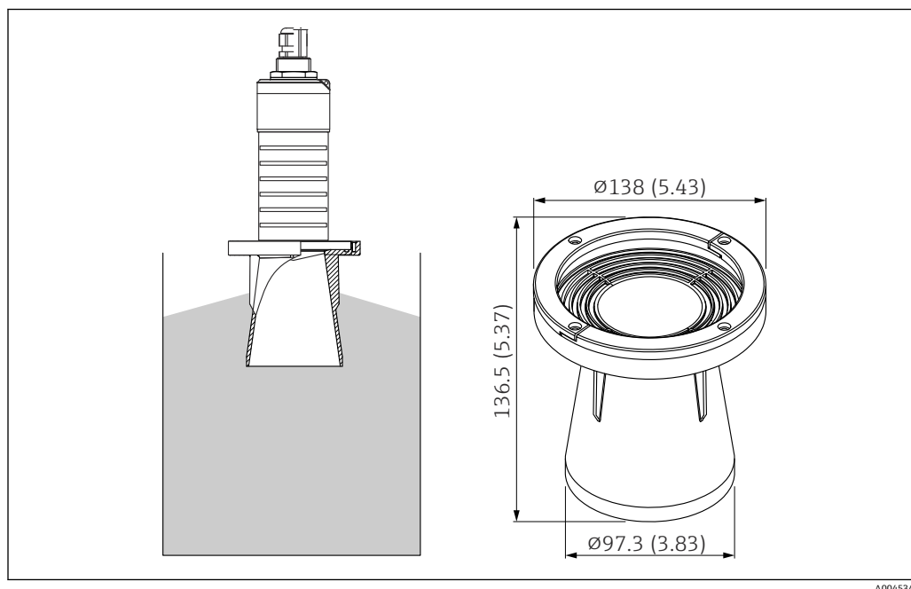
图 42 80 mm (3 in)防溢管的外形尺寸；单位：mm (in)
