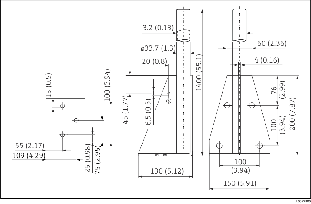
图 57 外形尺寸。测量单位 mm (in)
