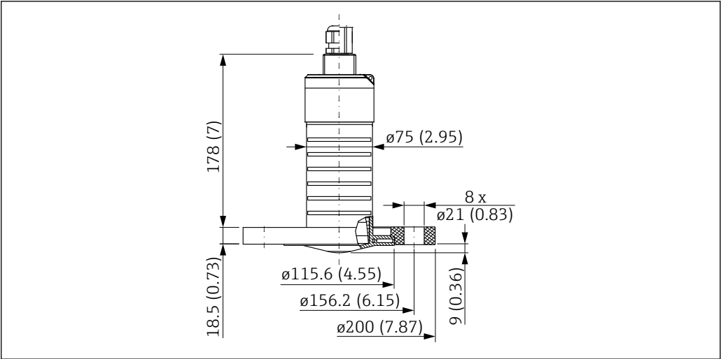
31 80 mm (3 in)口径天线的外形尺寸，安装有 3"/DN80 松套法兰；单位：mm (in)
