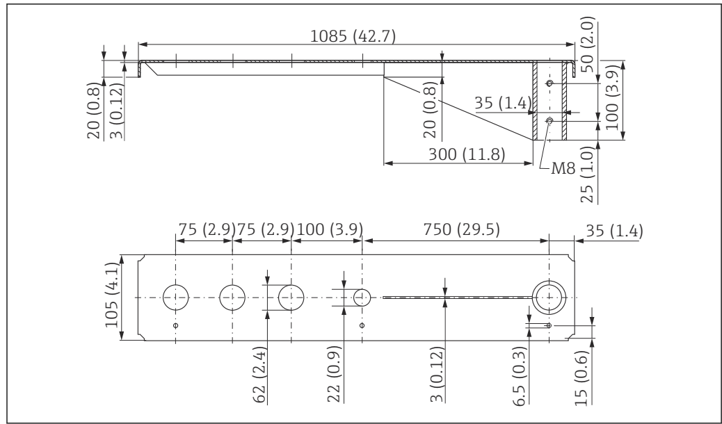
图 55 外形尺寸。测量单位 mm (in)
