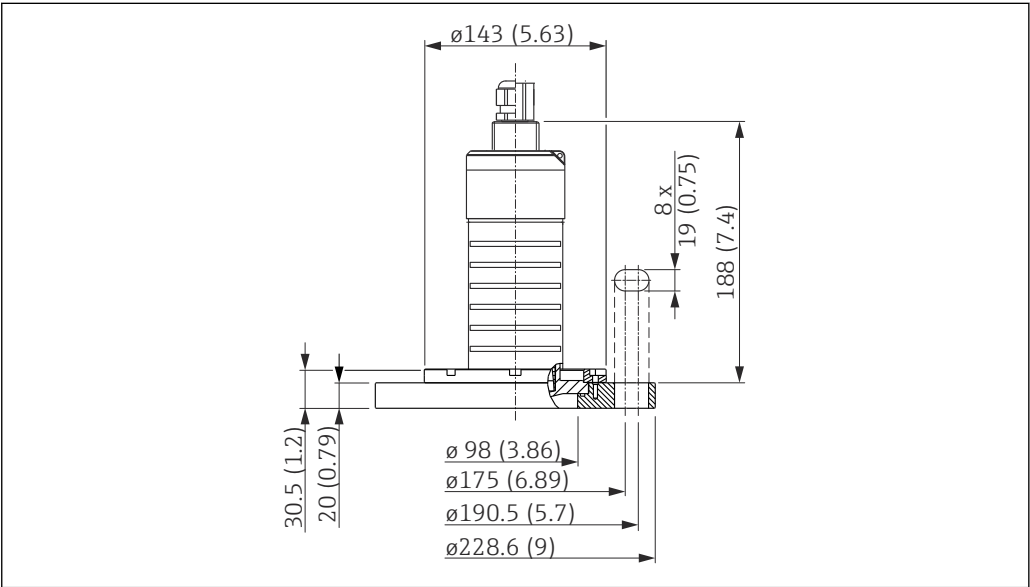
32 80 mm (3 in)口径天线的外形尺寸，安装有 4"/DN100 松套法兰；单位：mm (in)
