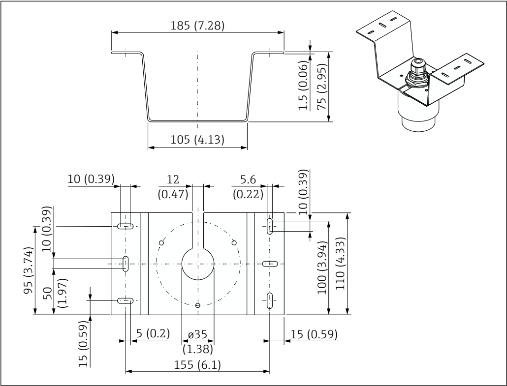
59 罐顶安装架的外形尺寸。测量单位 mm (in)
