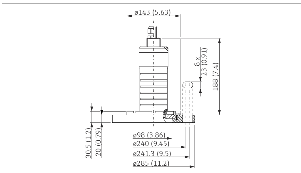
图 33 80 mm (3 in) 口径天线的外形尺寸，安装有 6"/DN150 松套法兰；单位：mm (in)
