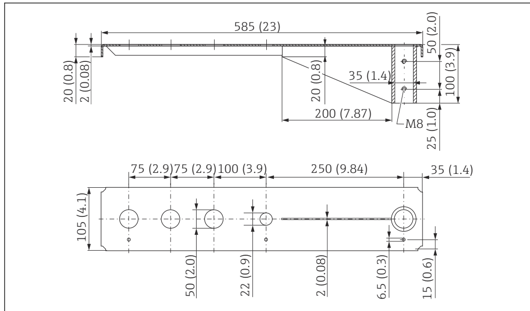
图 52 外形尺寸。测量单位 mm (in)
