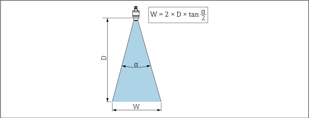
图 15 波束角 \alpha 、距离 D 和波束宽度 W 的相互关系
