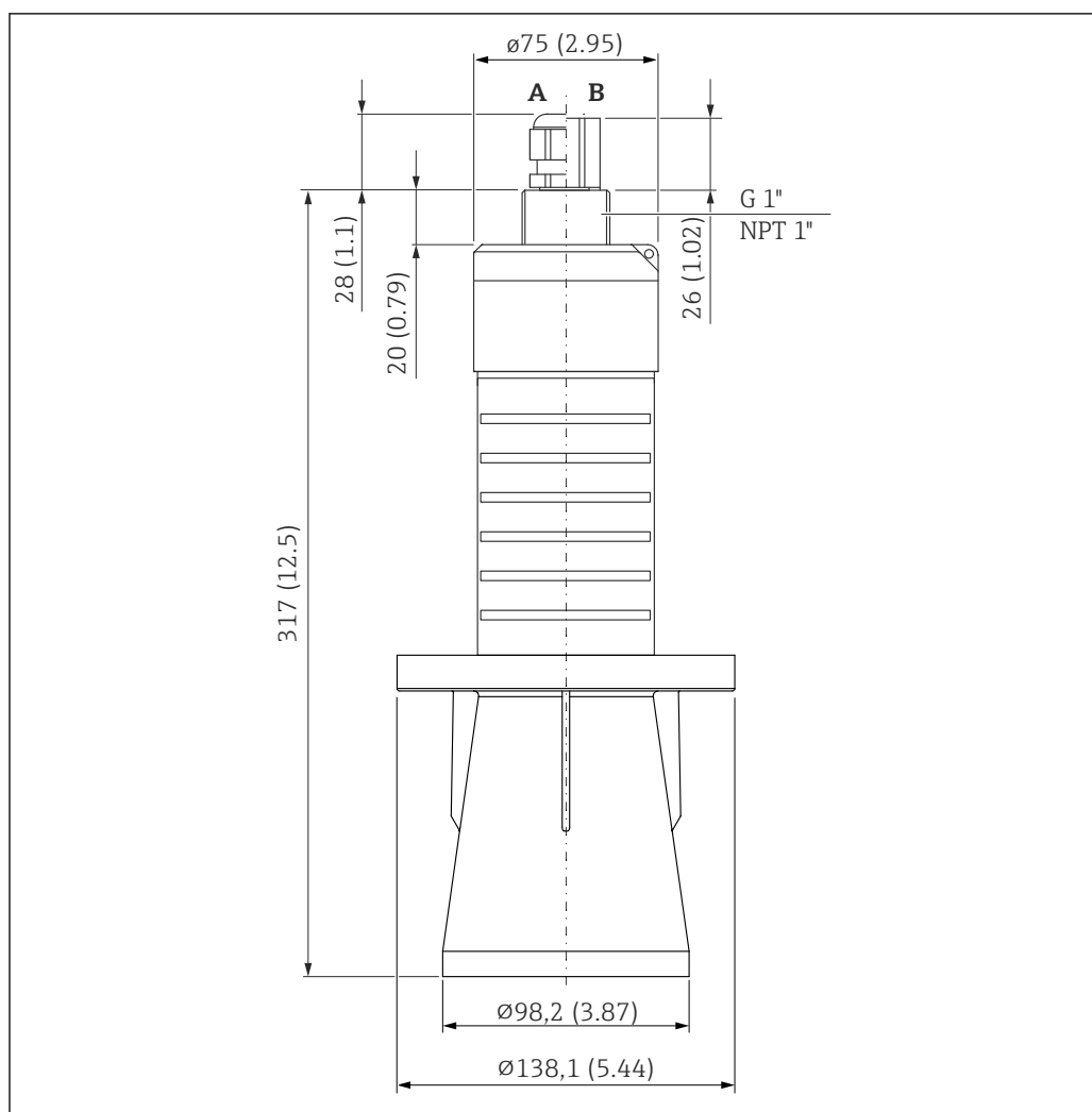
图 30 80 mm (3 in) 口径天线的外形尺寸，安装有防溢管；单位：mm (in)
