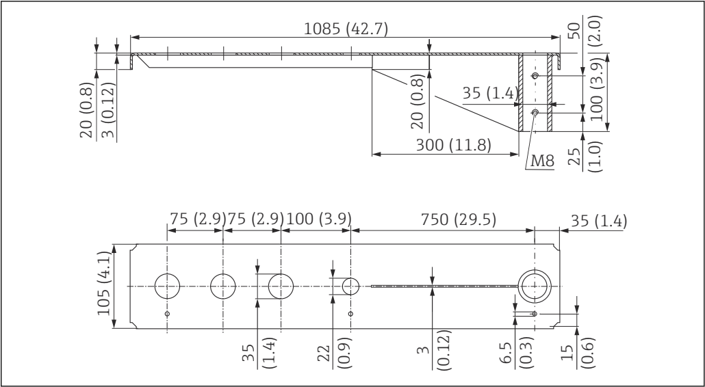
50 外形尺寸。测量单位 mm (in)
