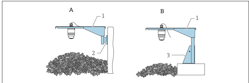
图 48 传感器过程连接（背面）的安装方式
