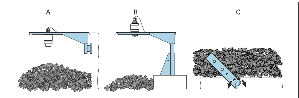
图 20 使用悬臂安装（可旋转）
