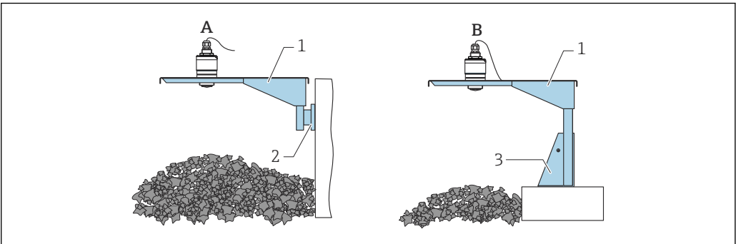
51 传感器过程连接（正面）的安装方式
