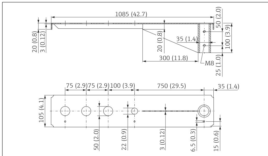
图 53 外形尺寸。测量单位 mm (in)
