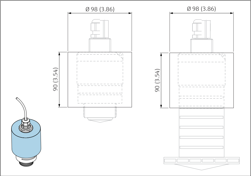
38 防护罩的外形尺寸；单位：mm (in)
