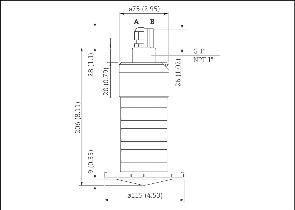
29 80 mm (3 in)口径天线的外形尺寸；单位：mm (in)
