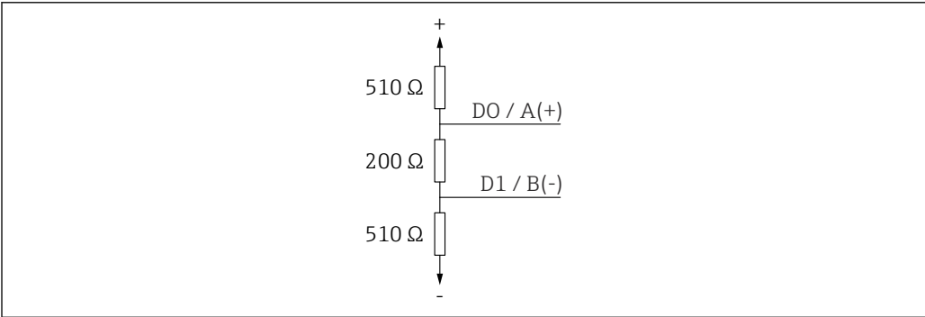
8 总线终端电阻连接，符合 RS485-IS 规范
