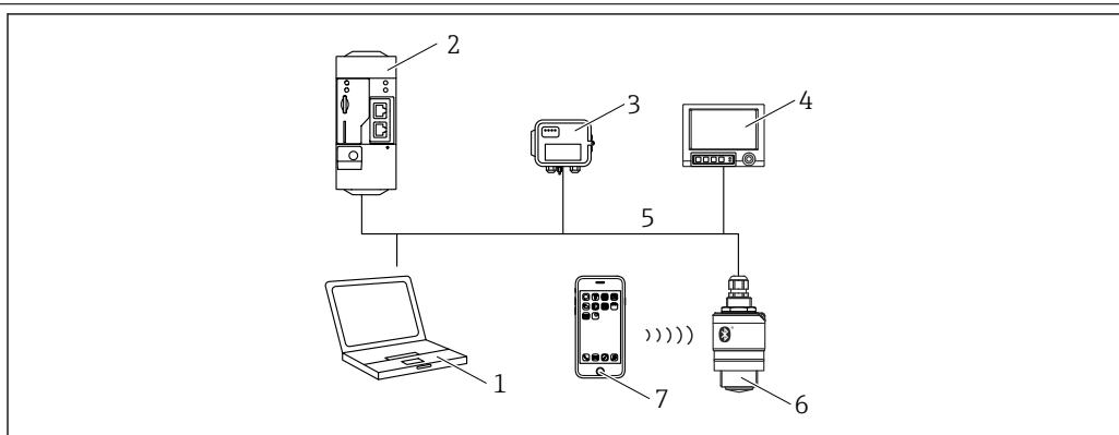
图 37 通过 Modbus 通信实现远程操作
