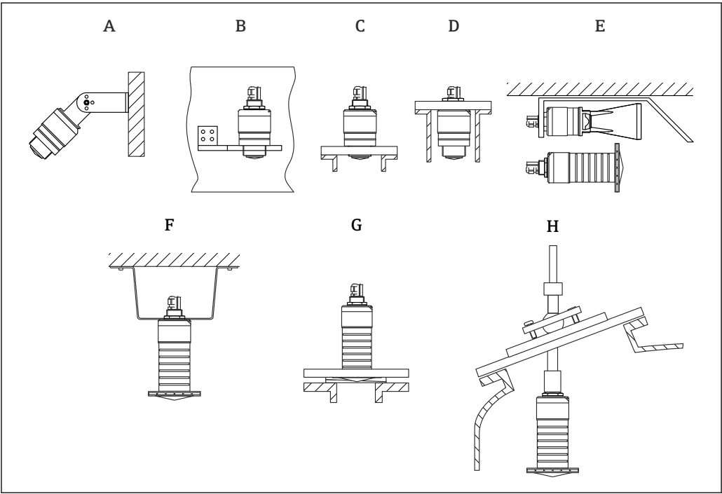
图 10 安装在墙壁上、罐顶上或安装短管中
