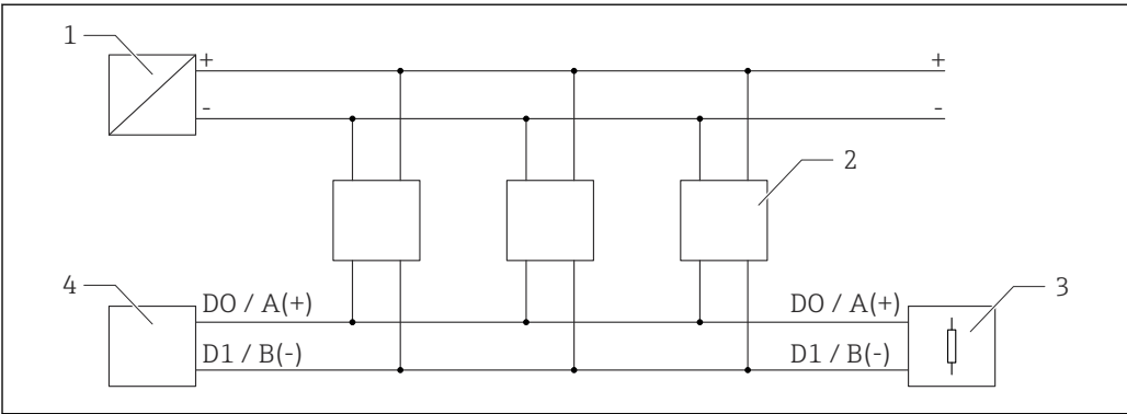
7 Modbus RS485 信号回路连接（多用户）
