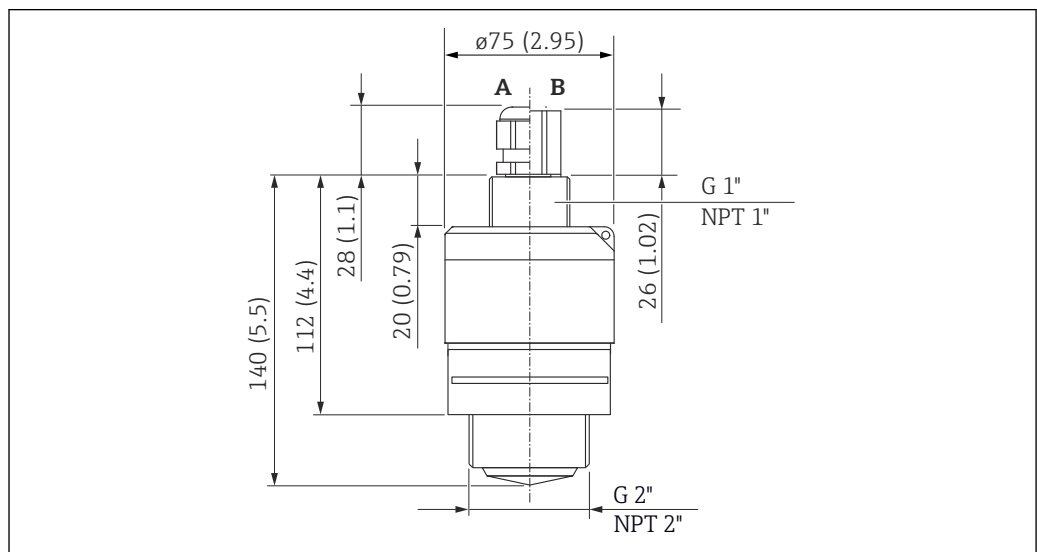
图 27 G 2" 或 MNPT 2" 过程连接螺纹的外形尺寸；单位：mm (in)
