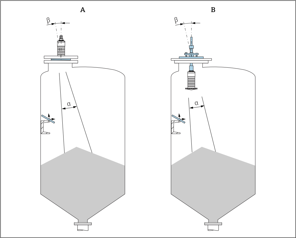
图 14 传感器垂直于介质仓底
