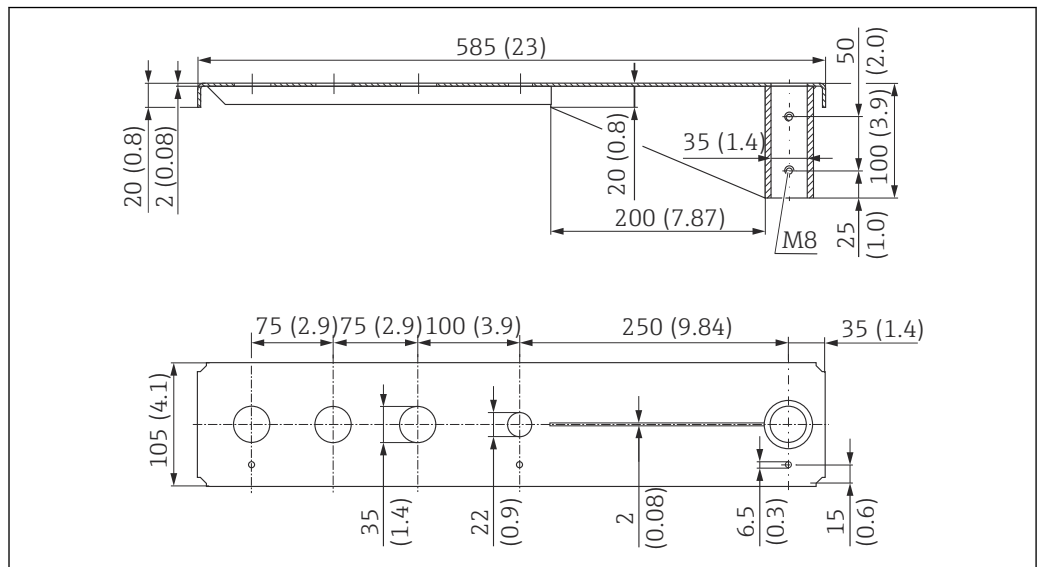
图 49 外形尺寸。测量单位 mm (in)
