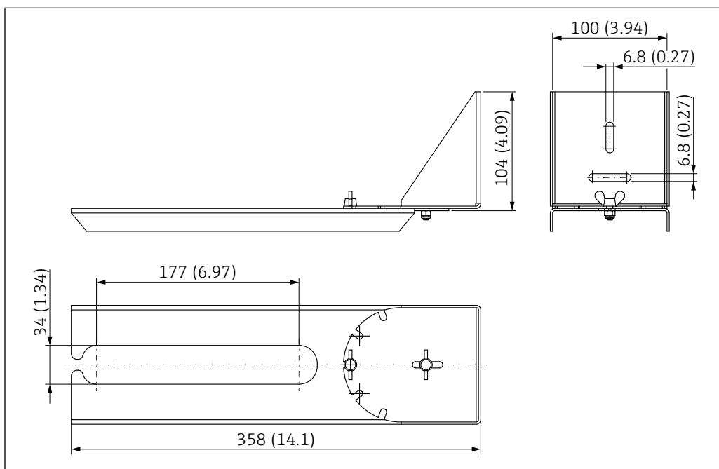
图 60 旋转安装架的外形尺寸。测量单位 mm (in)
