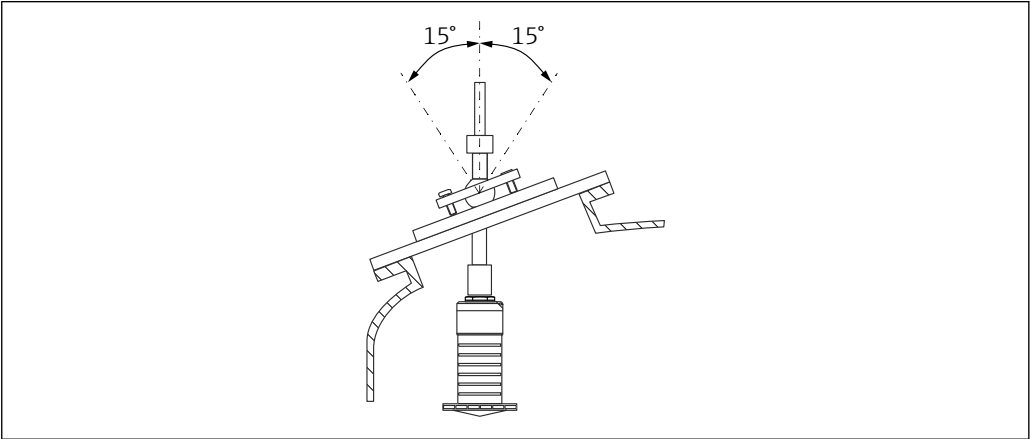
23 带天线角度调节装置的 Micropilot FMR20
