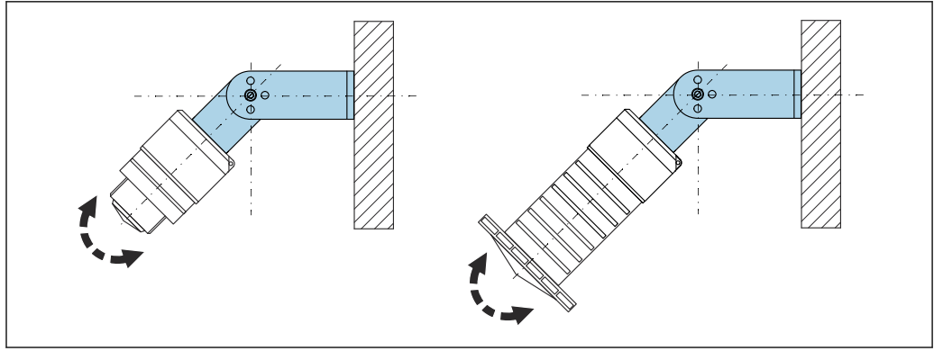
图 19 使用墙装架安装（可调节）
