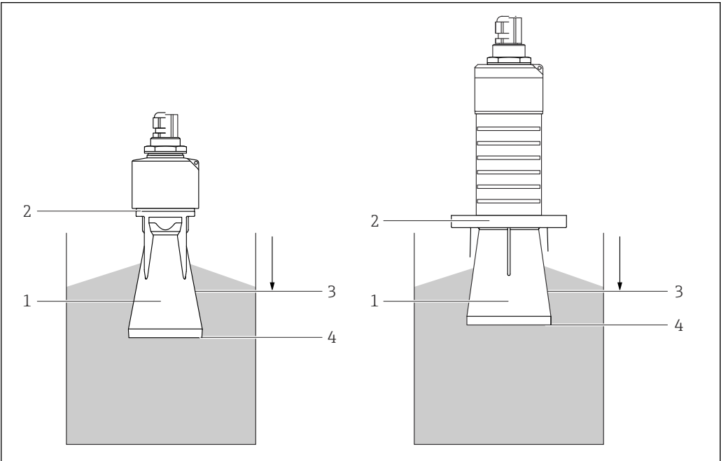
18 防溢管的功能
