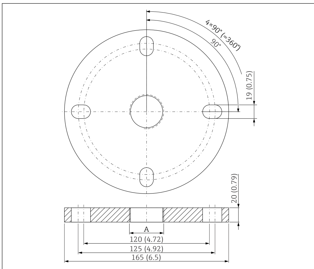
图 44 UNI 2"/DN50/50 法兰的外形尺寸；单位：mm (in)
