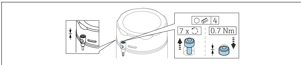
2 Крышка с крепежным винтом; гигиенический корпус (только для взрывозащиты от пыли)
