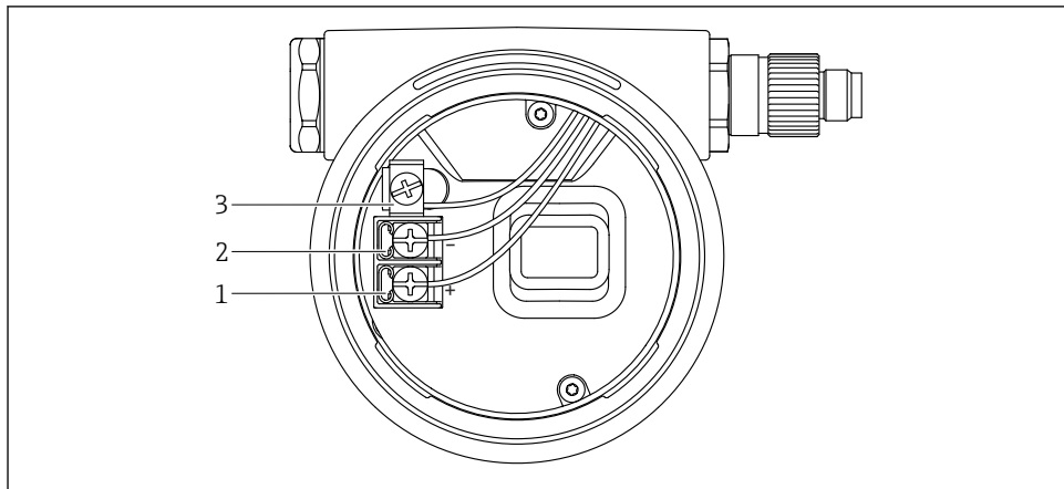
図 4 端子部の接続端子と接地端子
