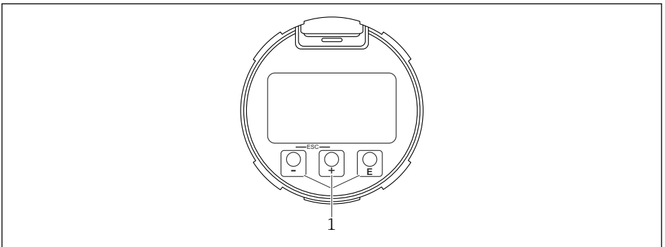
図 8 光学式操作キー (1) 付きグラフィックディスプレイ
