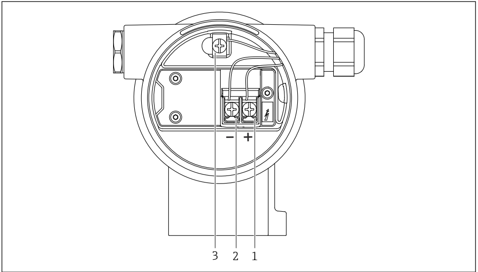
図 5 端子部の接続端子と接地端子
