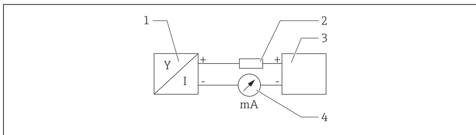
6 Blokdiagram van HART-aansluiting
