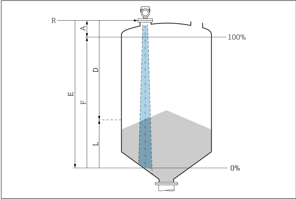
图 13 固体散料料位测量的设置参数
