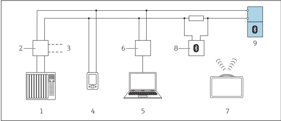
图 12 通过 HART 通信实现远程操作
