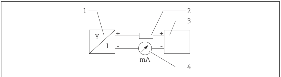
图 6 HART 信号回路连接框图
