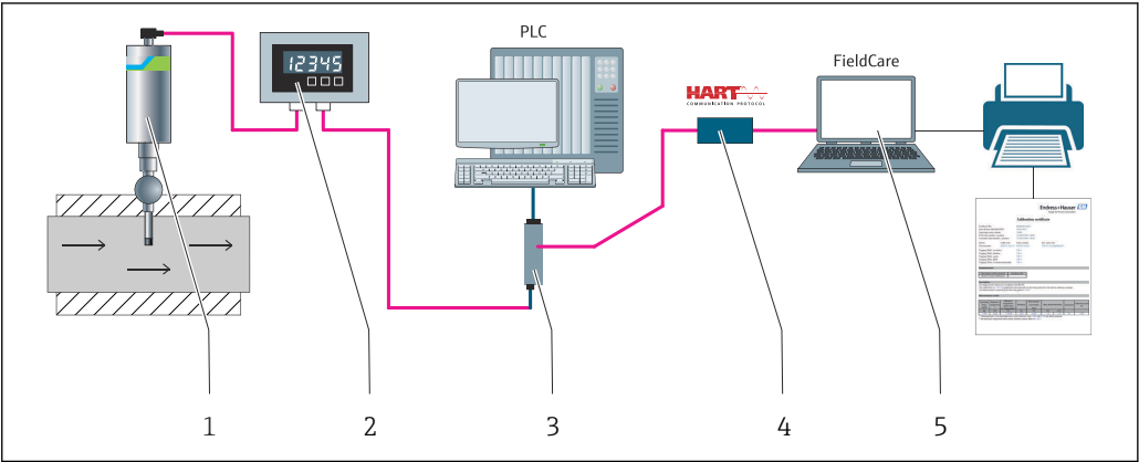
图 7 设备的操作方式
