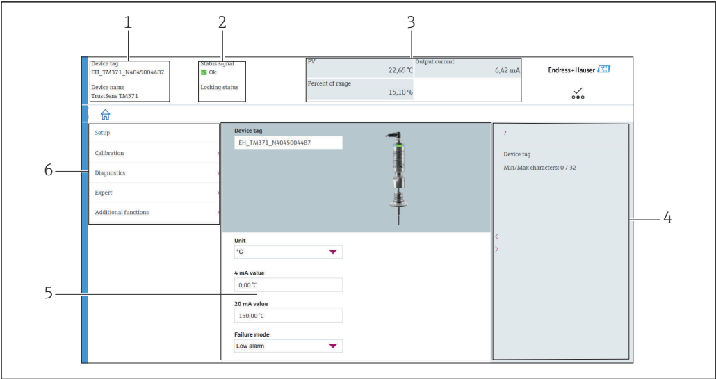
图 8 用户界面，通过 HART®通信显示设备信息
