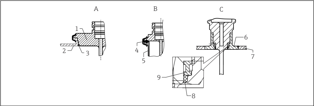
图 5 保证卫生合规的安装指南（取决于仪表选型）
