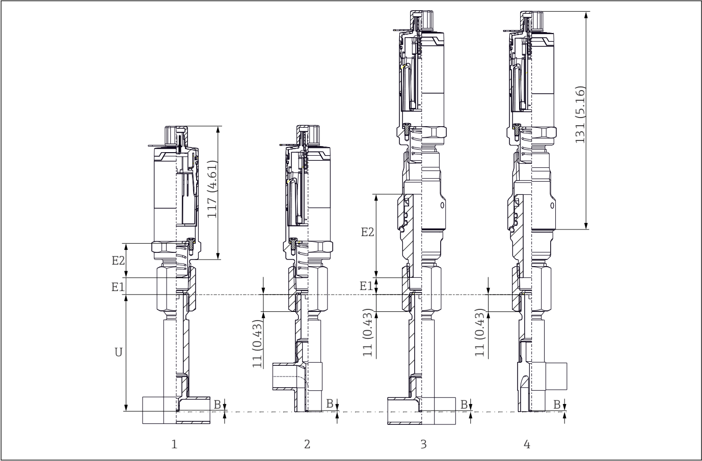
温度计，带 T-piece 或直角弯头保护套管
