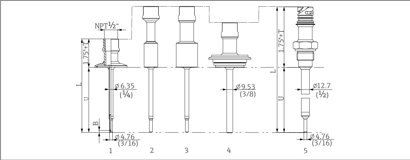
图 11 保护套管，带 NPT 1/2"螺纹延长颈和各类过程连接:
