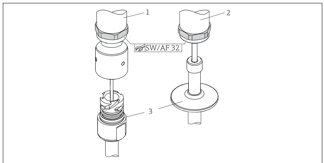
2 紧凑型温度计的安装过程
