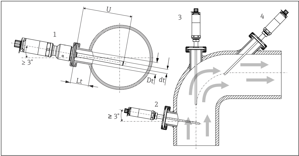
图 3 在过程中的允许安装位置 1、2 安装方向与介质流向垂直，为了确保自排空，倾斜安装角度不得小于 3° 3 安装在管道弯头位置处 4 倾斜安装在小标称口径管道中 U 插深
