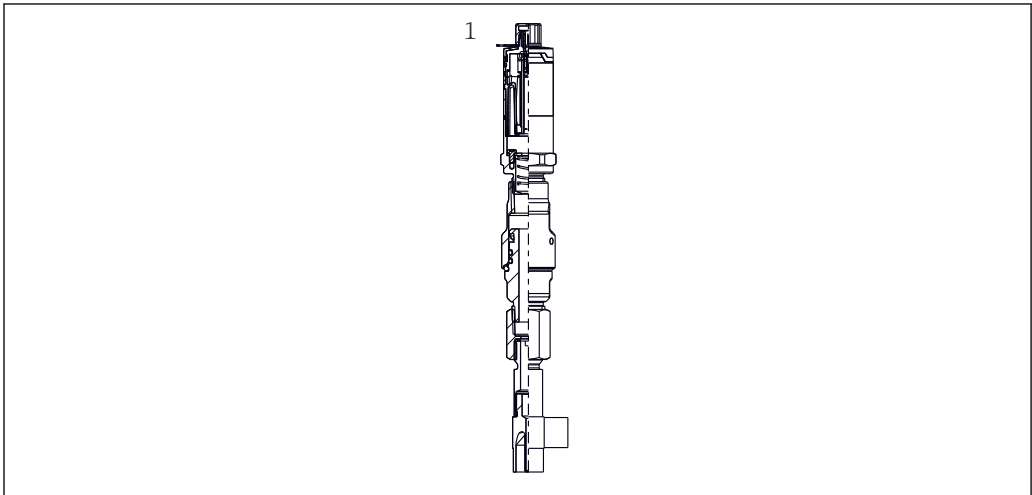
图 4 在小标称口径管道中安装的温度计的过程连接 1 弯头保护套管，焊接安装，符合 DIN 11865 / ASME BPE 2012 标准
