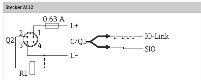
IO-Link: 2 x PNP-Schaltausgang R1 und R2
