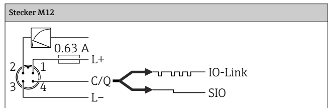
IO-Link: 1 x PNP Schaltausgang R1 mit zusätzlichem Analogausgang 4...20 mA (aktiv)
