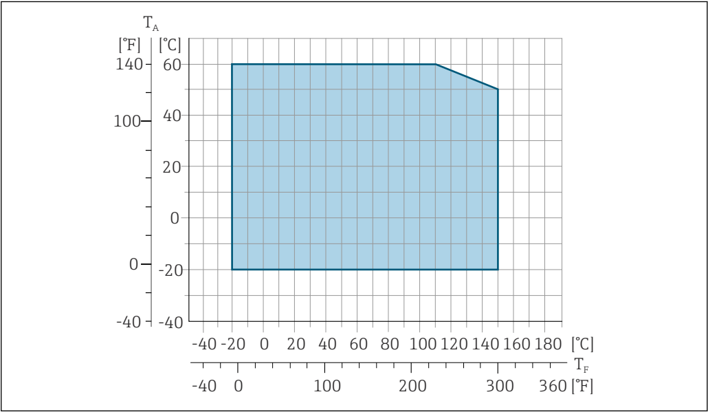
33 Promag 500 (数字)
