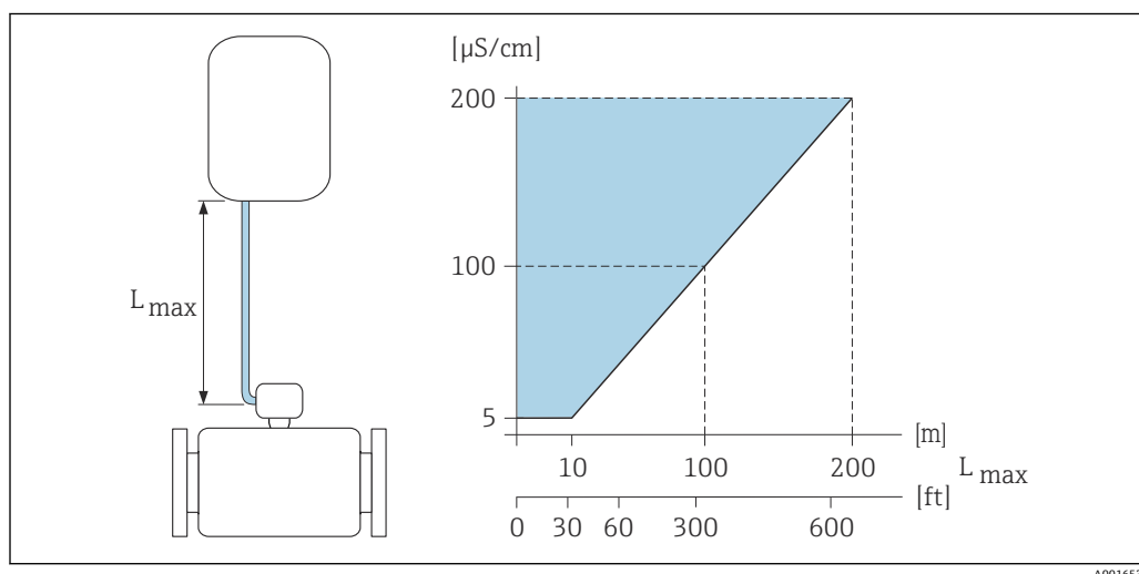
图 26 允许连接电缆长度
