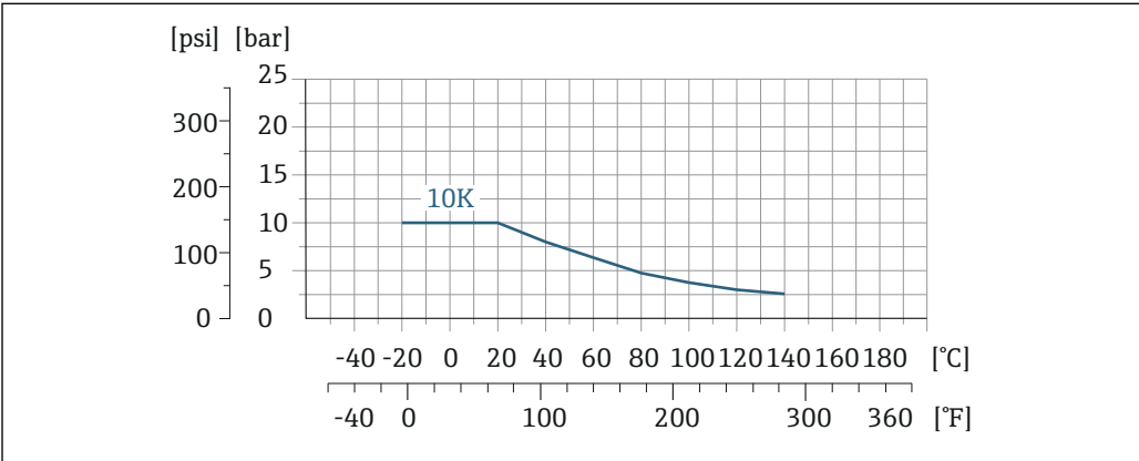
42 过程连接材质: PVDF
