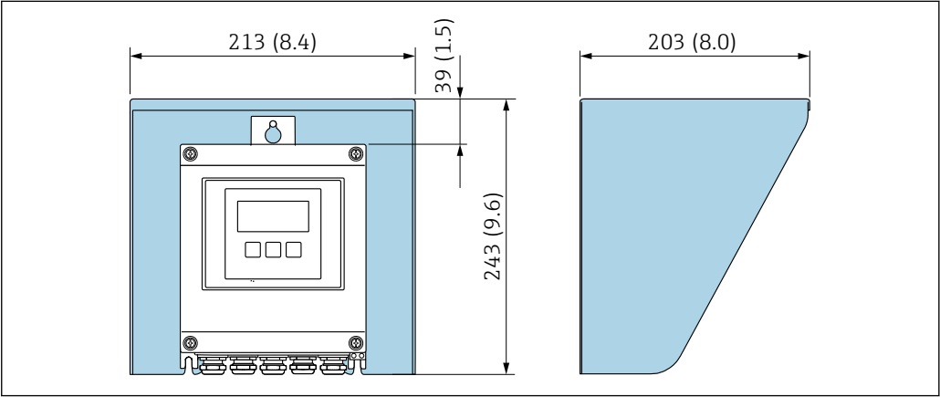
63 Proline 500 (数字) 变送器的防护罩的外形尺寸图; 单位: mm (in)
