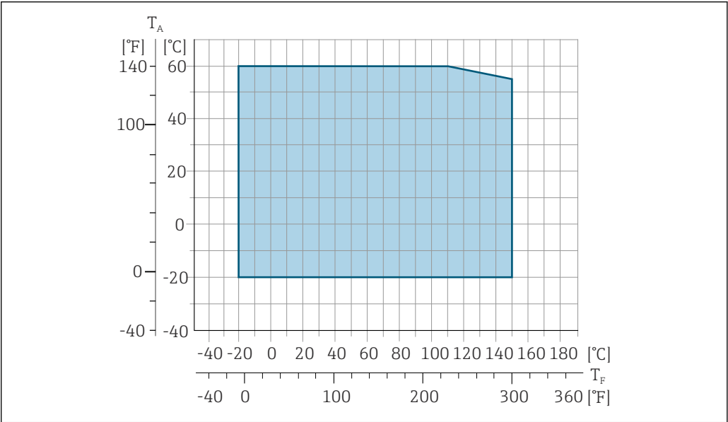
34 Promag 500 (模拟)
