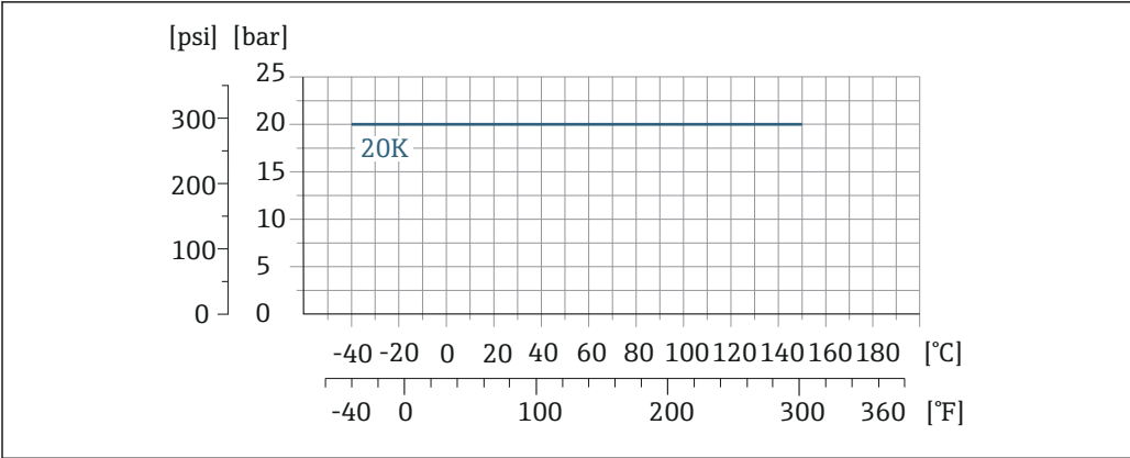
41 过程连接材质: 不锈钢 1.4404 (F316L)
