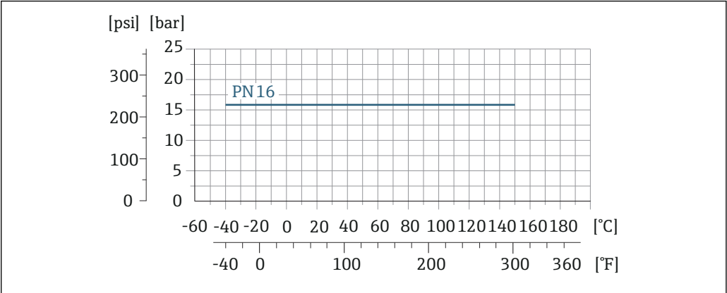
44 过程连接材质：不锈钢 1.4404 (F316L)
