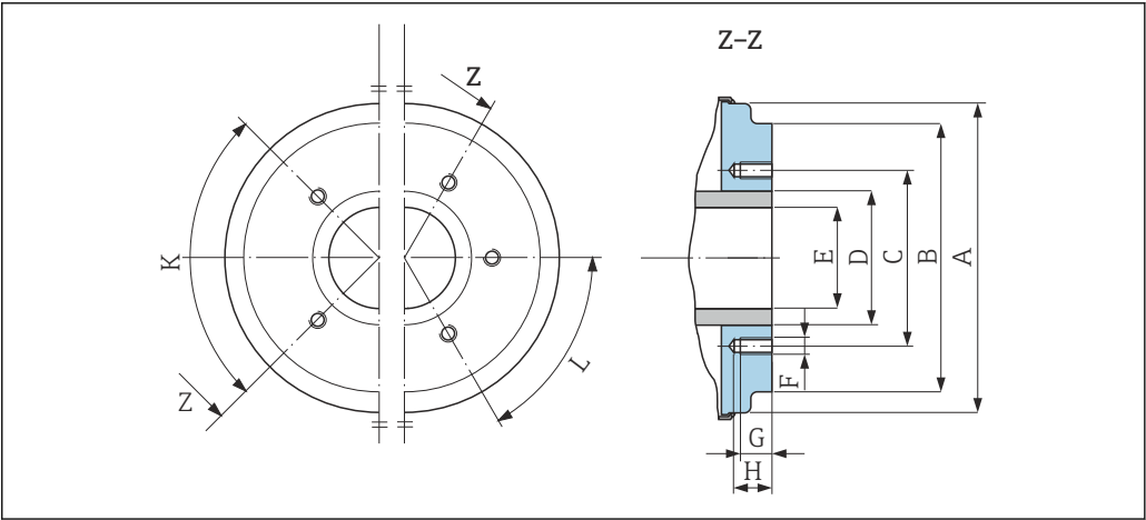
52 正视图，未安装过程连接
