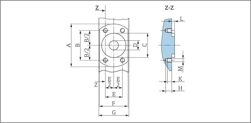
51 正视图，未安装过程连接
