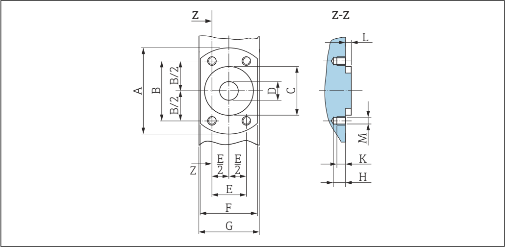
图 61 正视图，未安装过程连接
