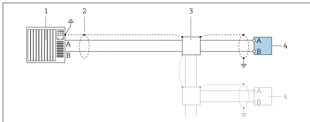
图 12 接线实例：Modbus RS485，非危险区和 Zone 2/Div. 2 防爆场合
