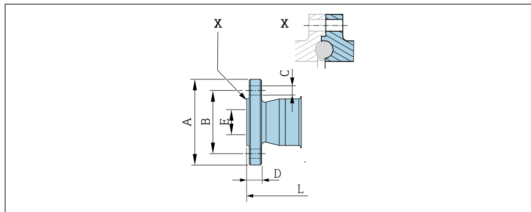
图 53 视图 X: 非对称过程连接; 蓝色部分由供应商提供。
