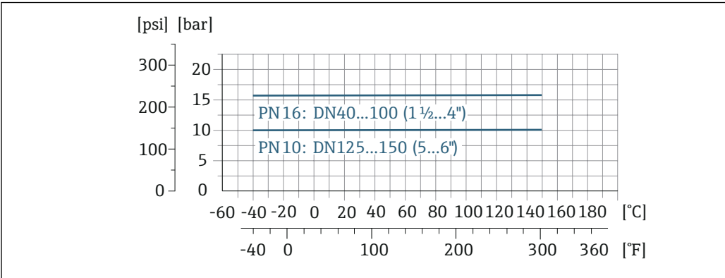
图 47 过程连接材质：不锈钢 1.4404 (F316L)
