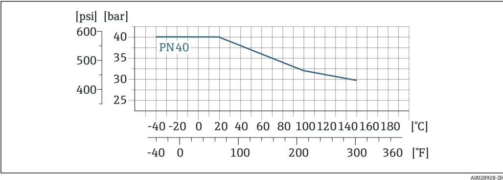
图 36 过程连接材质：不锈钢 1.4404 (F316L)
