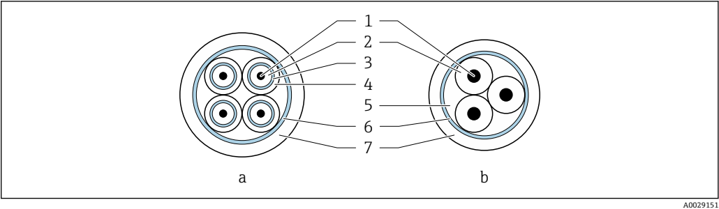
图 22 电缆截面图
