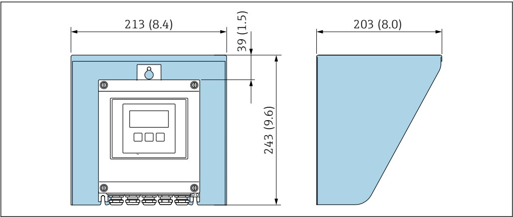
图 31 Proline 500（数字）变送器的防护罩的外形尺寸图；单位：mm (in)
