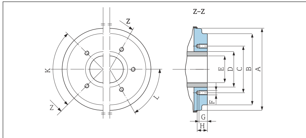
图 62 正视图，未安装过程连接
