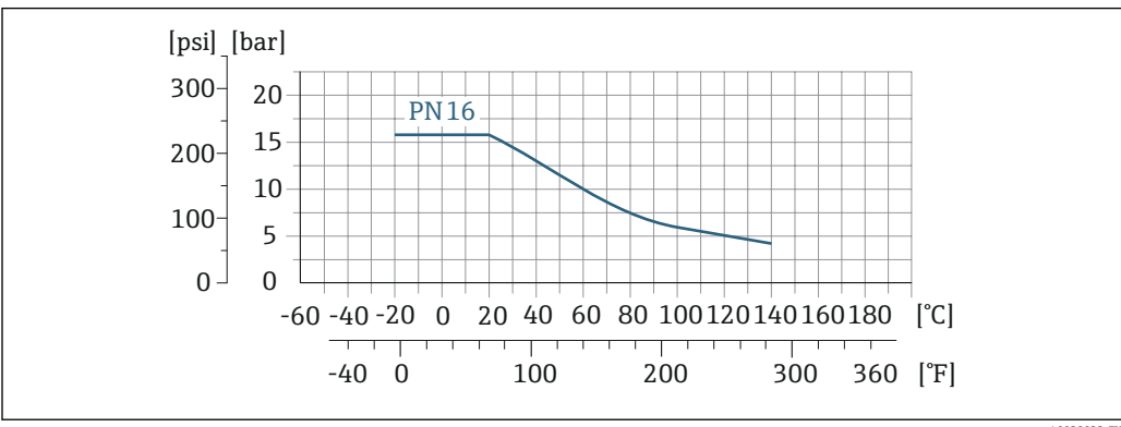
图 37 过程连接材质：PVDF
