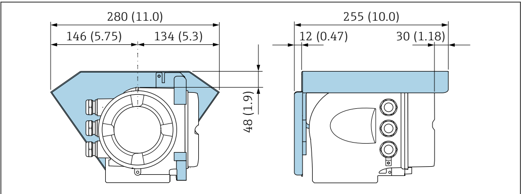
图 32 Proline 500（模拟）变送器的防护罩的外形尺寸图；单位：mm (in)
