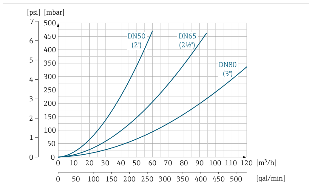
48 Perda de pressão DN 50 a 80 (2 a 3") para o código de pedido para "Projeto", opção C "Flange fixa, tubo de medição comprimido", 0 x DN trechos retos a montante e a jusante"
