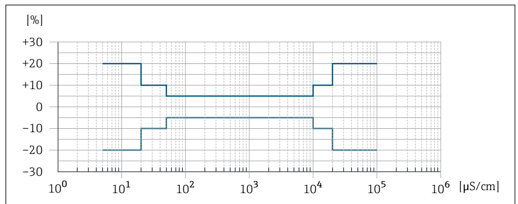
47 Erro medido (opcional: código de pedido para "Medição de condutividade calibrada", opção CW)
