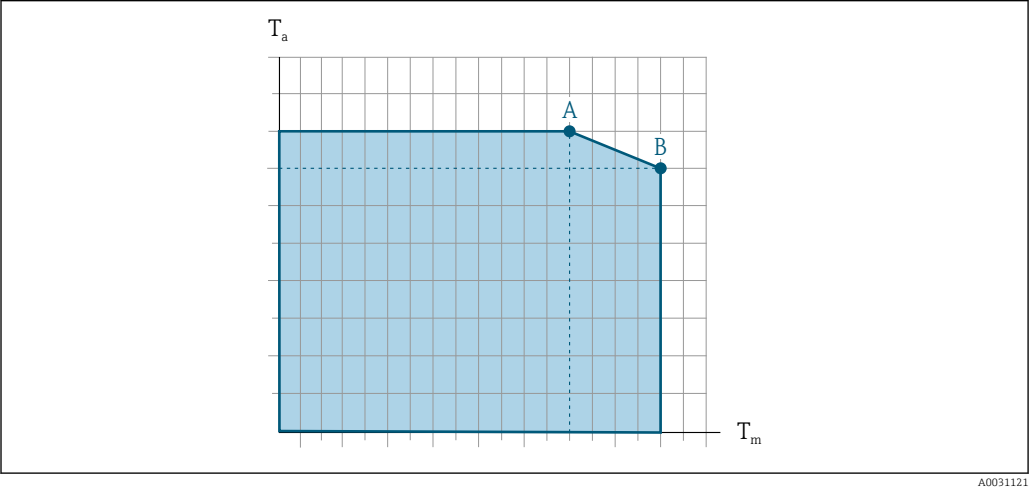
48 Exemple, valeurs dans le tableau ci-dessous. T_a Température ambiante T_m Température du produit A Température de produit maximale admissible T_m à T_{a\ max} = 60\ ^\circ\text{C}\ (140\ ^\circ\text{F}) ; des températures de produit T_m plus élevées requièrent une réduction de la température ambiante T_a B Température ambiante maximale admissible T_a pour la température de produit maximale T_m spécifiée pour le capteur
