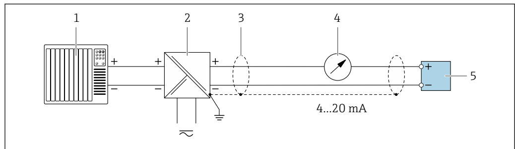
20 Exemple de raccordement de la sortie courant 4...20 mA HART (passive)
