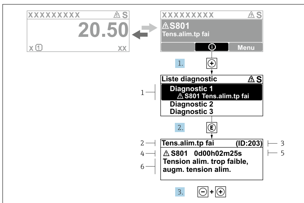
43 Message relatif aux mesures correctives
