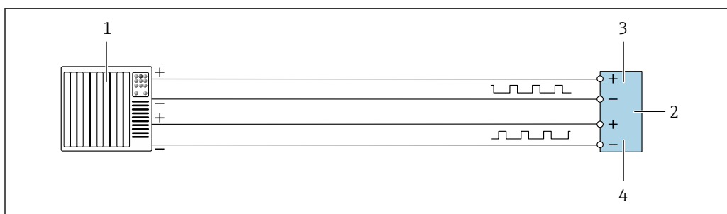
26 Exemple de raccordement pour la double sortie impulsion (active)
