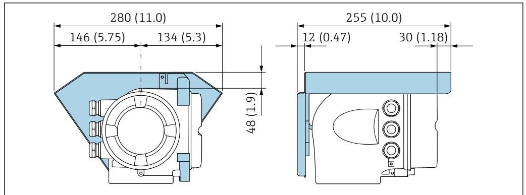
图 11 Proline 500 (模拟) 变送器的防护罩的外形尺寸图; 单位: mm (in)
