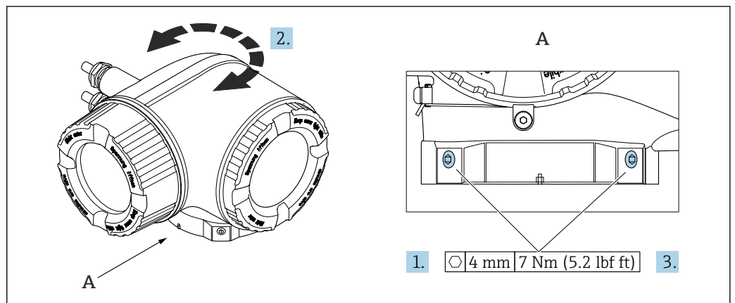
图 16 防爆型外壳
