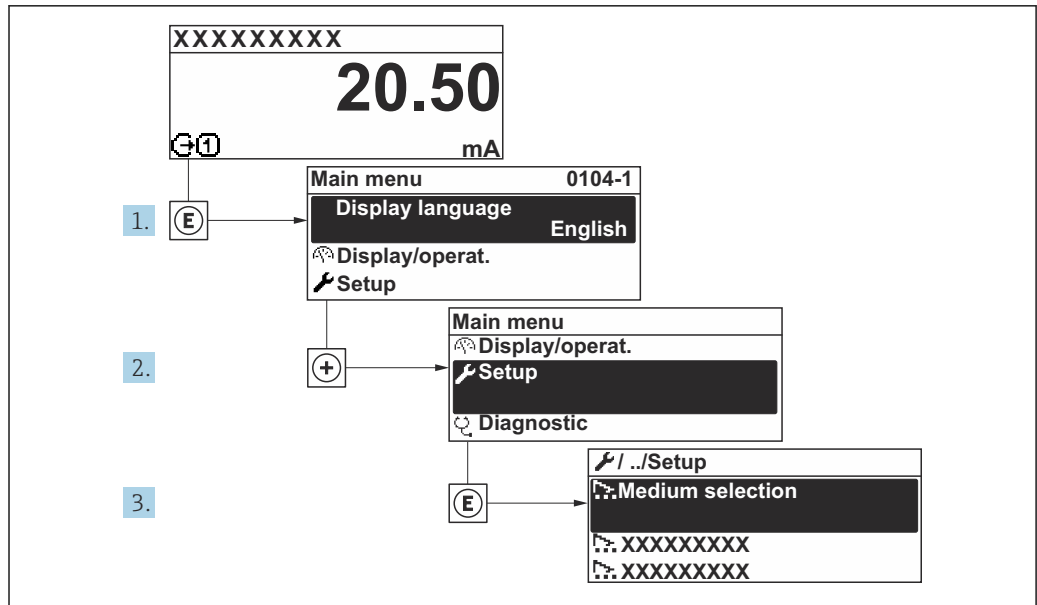
图 39 现场显示单元示例
