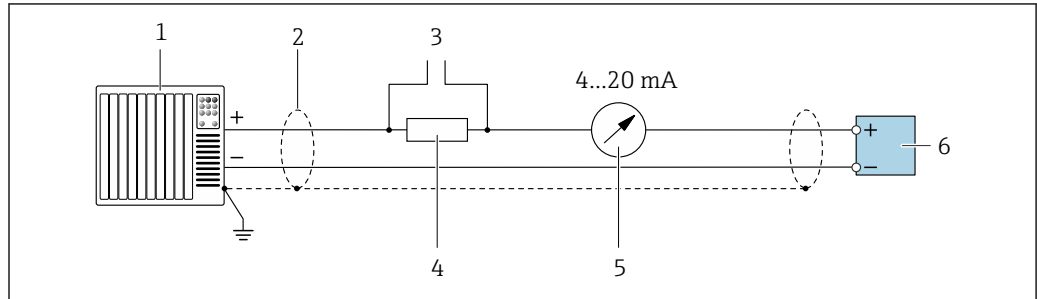
图 18 接线实例：4...20 mA HART 电流输出（有源信号）
