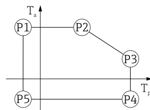
25 Invólucro plástico; temperatura do processo -40 para +80 °C (-40 para +176 °F)
