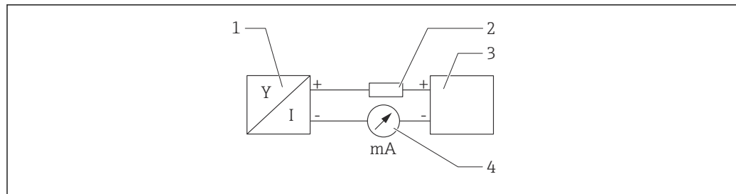
4 Diagrama do bloco da conexão HART
