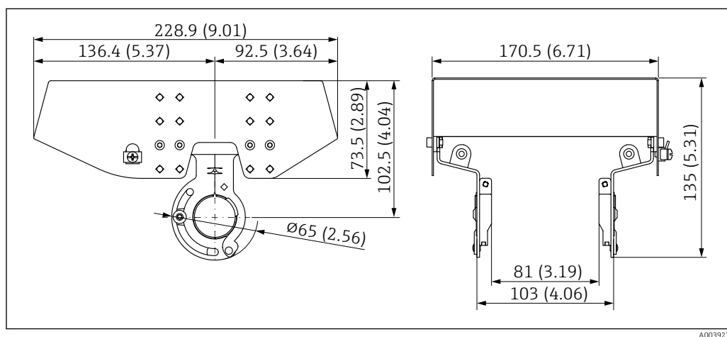
Fig. 17 Dimensões. Unidade de medida mm (in)
