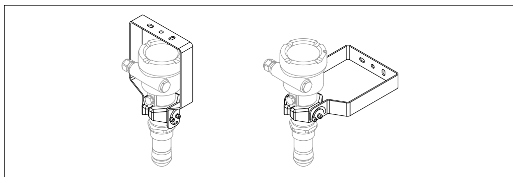
19 Монтаж на потолке или стене
