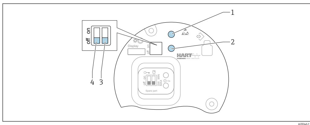
8 Кнопки управления и DIP-переключатели на электронной вставке HART
