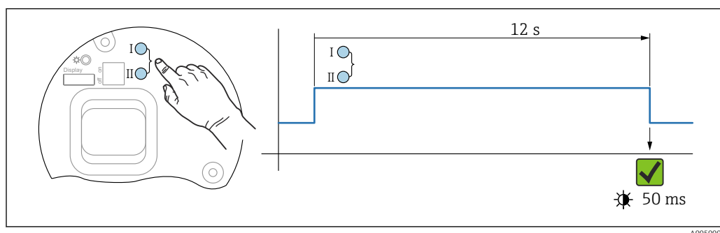
16 Кнопки управления на электронной вставке
