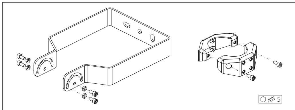
21 Комплект поставки регулируемого монтажного кронштейна
