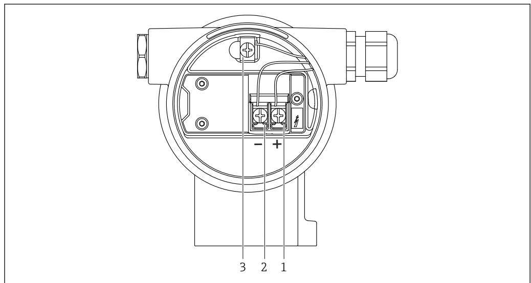
6 Соединительные клеммы и клемма заземления в клеммном отсеке
