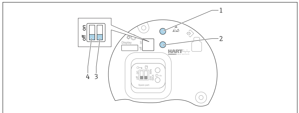
67 Teclas de operação e minisseletoras na unidade eletrônica HART
