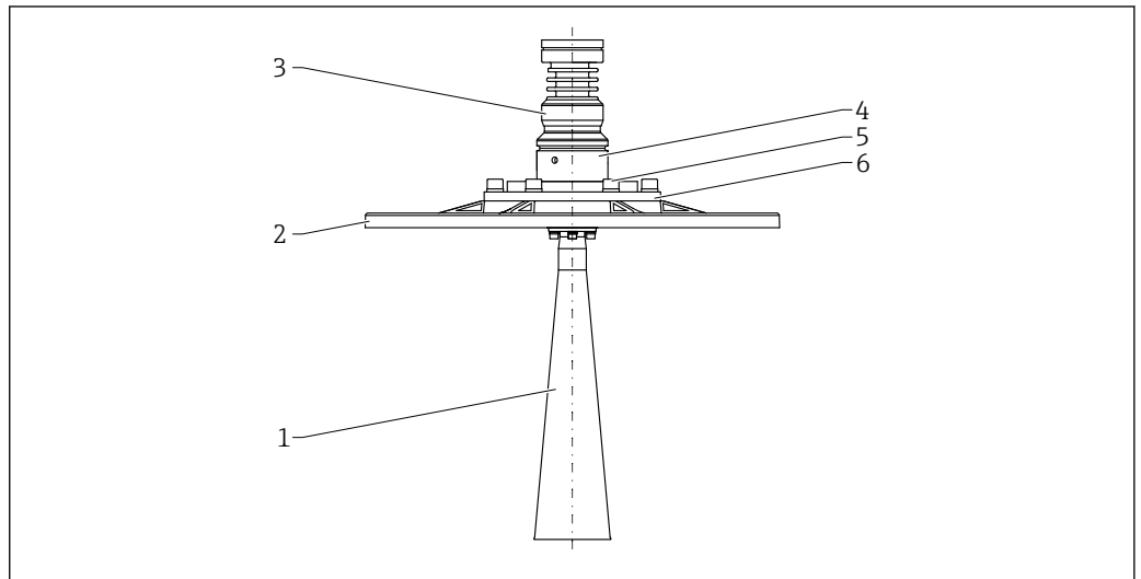
62 Material; antena piramidal DN65, com flange UNI e unidade de alinhamento. Unidade de medida mm (in)
