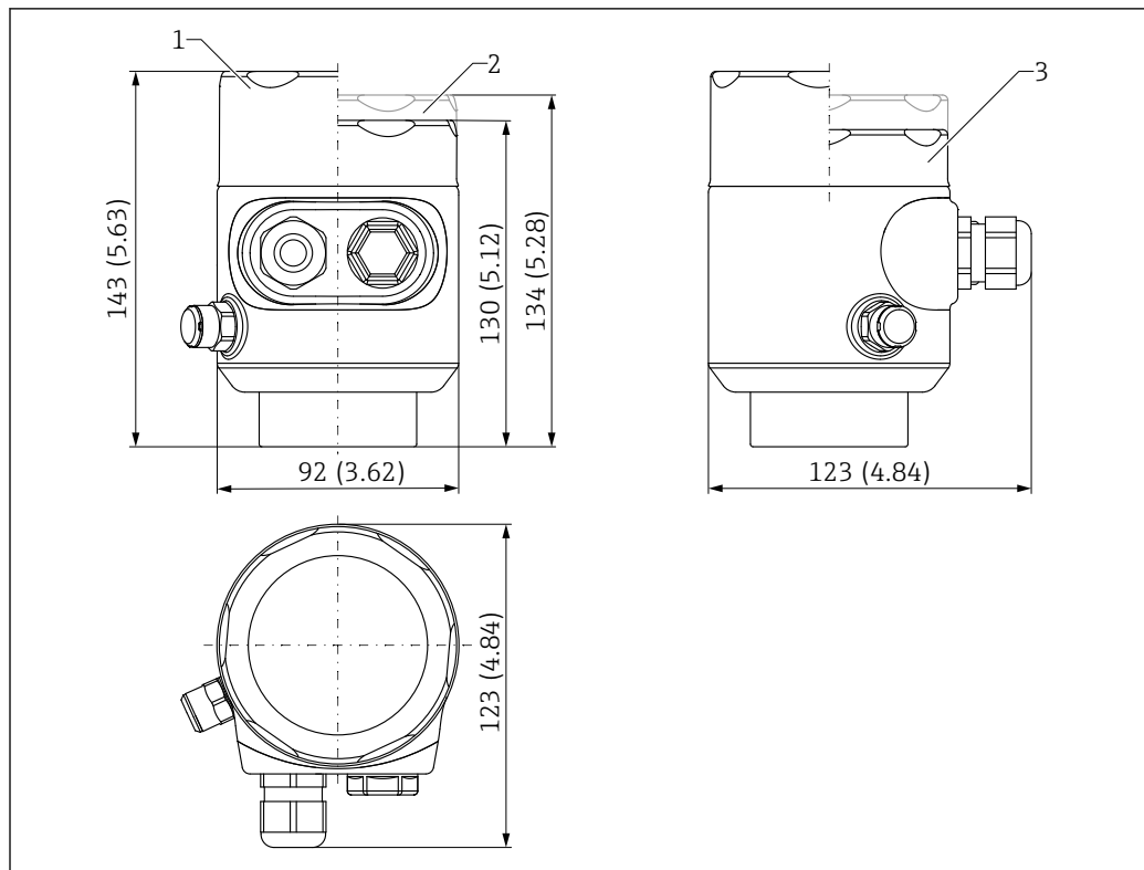
▣ 39 Dimensões do invólucro de compartimento único, 316L, higiene. Unidade de medida mm (in)
