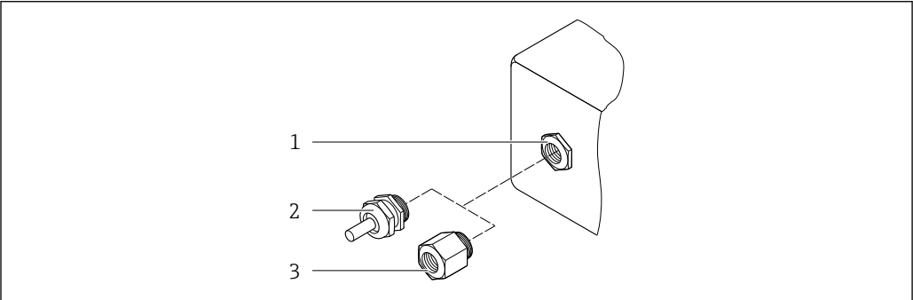
47 允许的电缆入口/缆塞 1 内螺纹 M20 × 1.5 2 缆塞 M20 × 1.5 3 转接头，适用 G ½"或 NPT ½"内螺纹电缆入口
