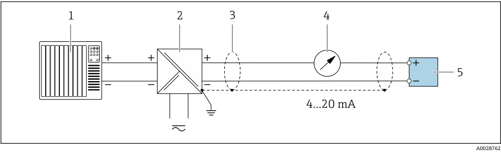
图 19 接线实例：4...20 mA HART 电流输出（无源信号）
