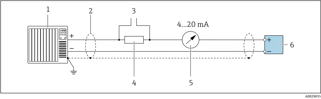
图 18 接线实例：4...20 mA HART 电流输出（有源信号）
