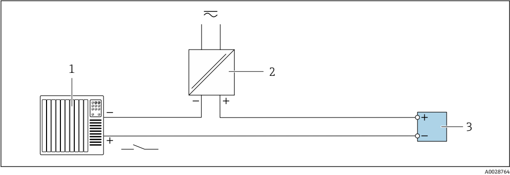
图 29 接线实例：状态输入 1 自动化系统，带状态输出（例如 PLC） 2 电源 3 变送器
