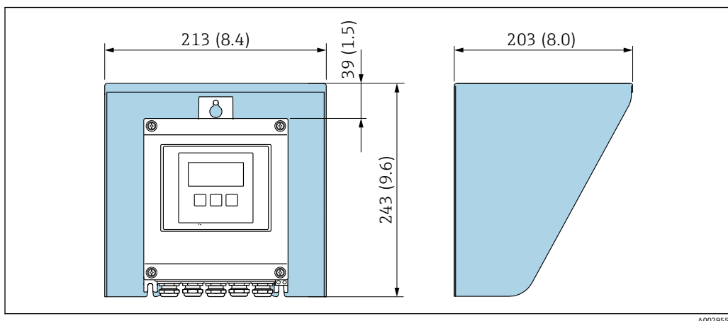
图 9 Proline 500 (数字) 变送器的防护罩的外形尺寸图; 单位: mm (in)
