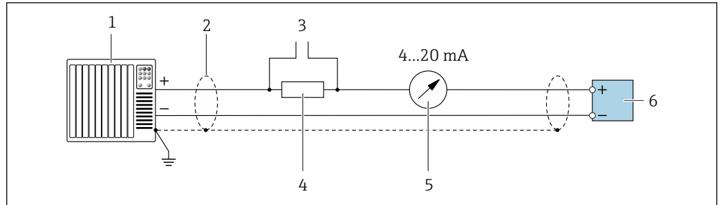
图 10 接线实例：4...20 mA HART 电流输出（有源信号）
