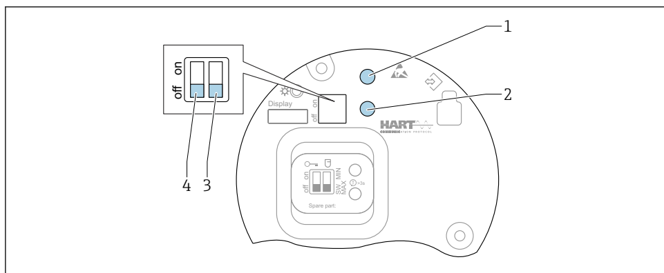
7 Ovládací tlačítka a DIP přepínače na modulu s elektronikou HART
