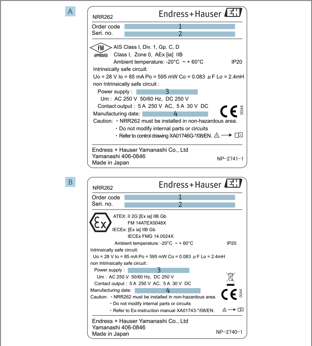
4 Plaque signalétique pour NRR262
