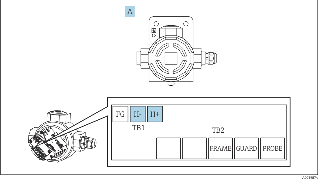
20 Boîtier de raccordement à sécurité intrinsèque
