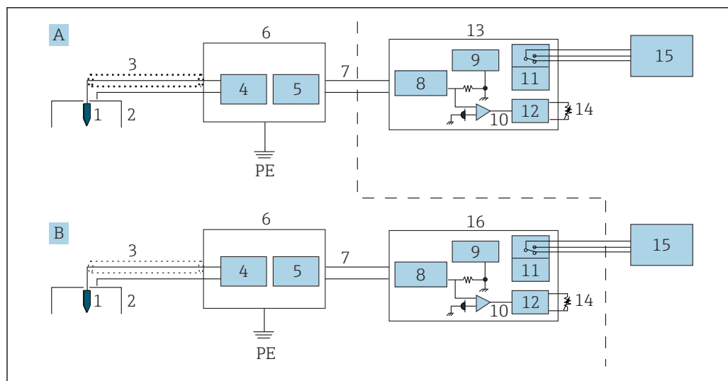
19 Schéma de raccordement
