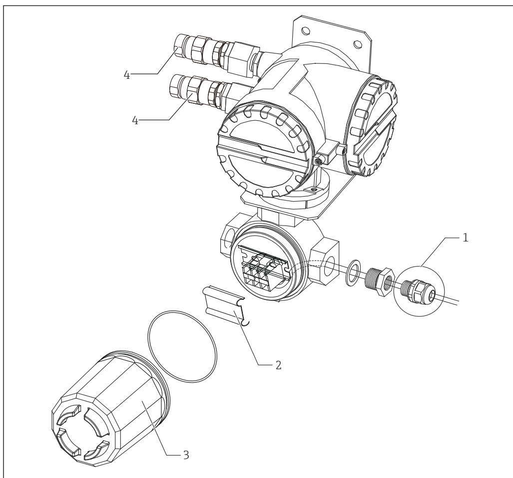
15 Montage du câble pour NRR261-5xx
