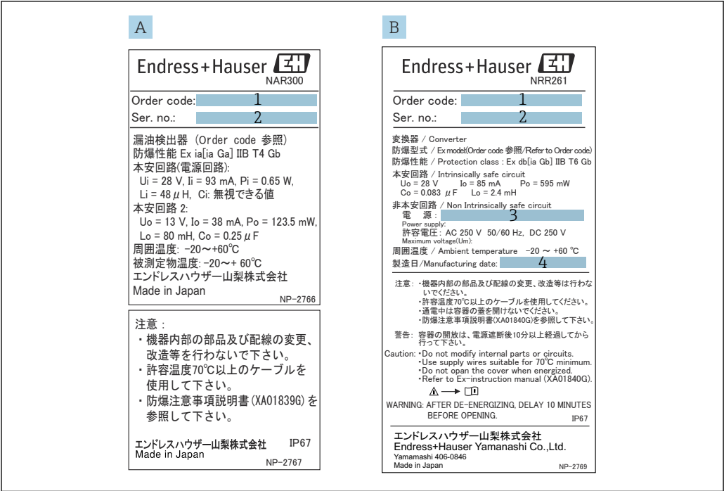
5 Plaque signalétique pour JPN Ex
