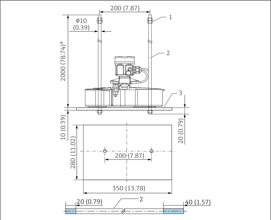
22 Guide de flotteur
