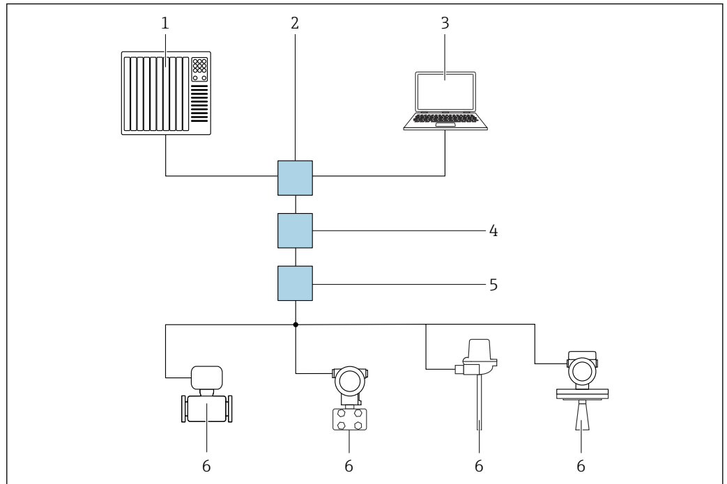
图 3 通过 PROFINET + Ethernet-APL 网络实现远程操作：星形拓扑结构
