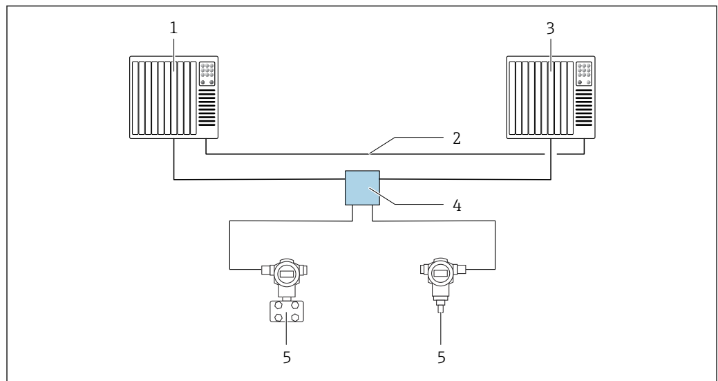
图 5 S2 系统冗余布局实例：星形拓扑结构
