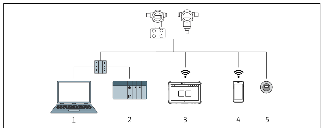
图 6 通过 PROFINET 通信实现远程操作
