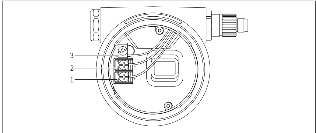
图 1 接线腔内的接线端子和接地端子
