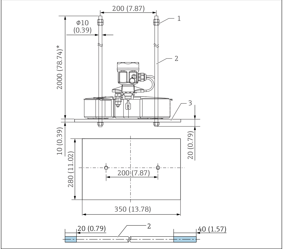
☐ 9 NAR300/플로트 가이드. 측정 단위 mm (in)
