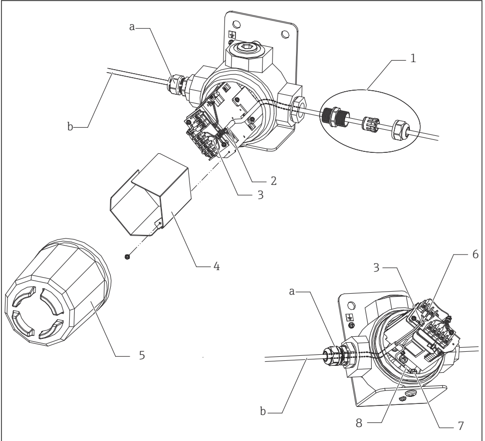
☐ 11 NAR300-x5xxxx 및 센서 I/F Ex 박스 케이블 설치
