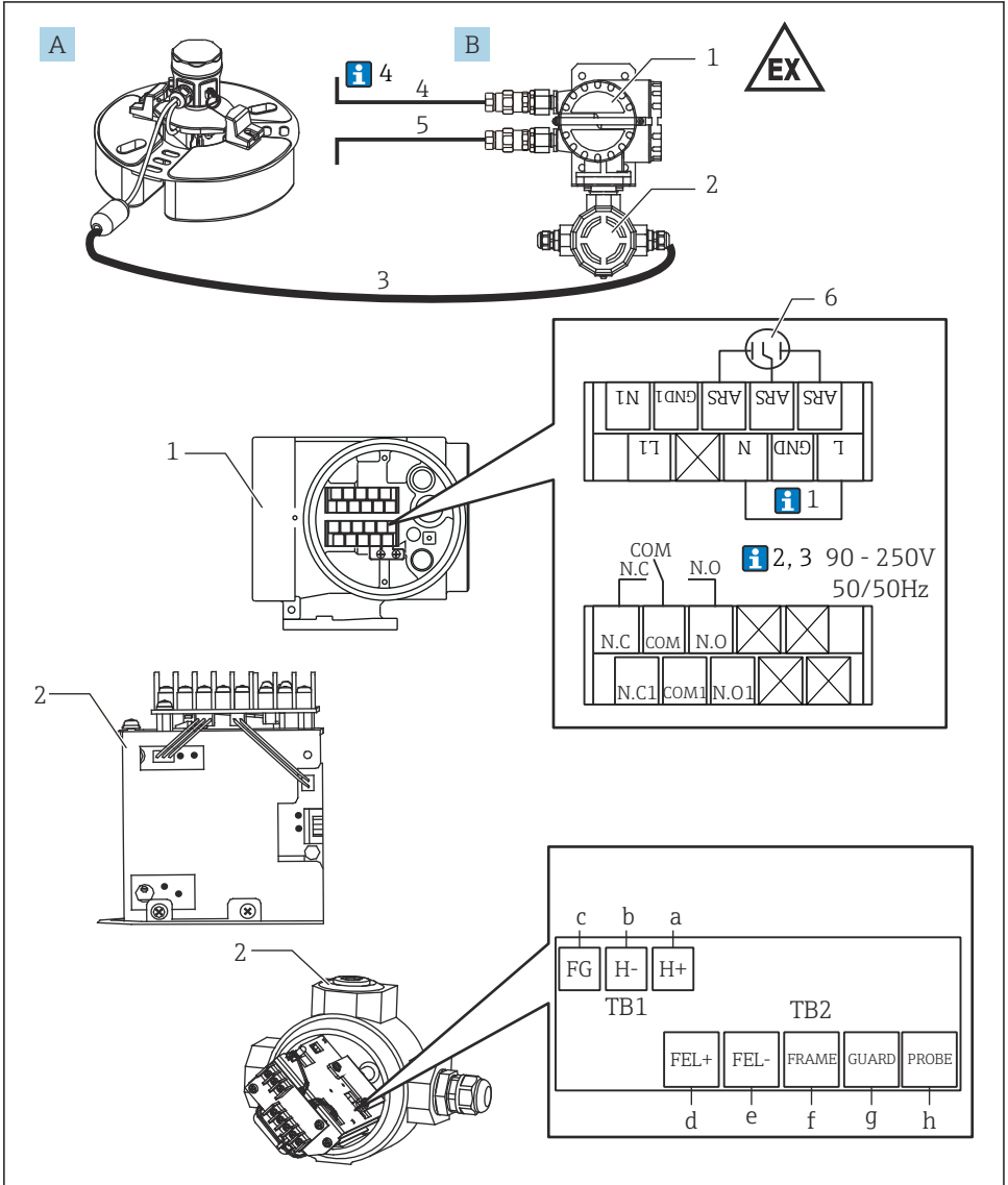
14 Ex d [ia] 컨버터 NRR261-4/A/B/C 결선
