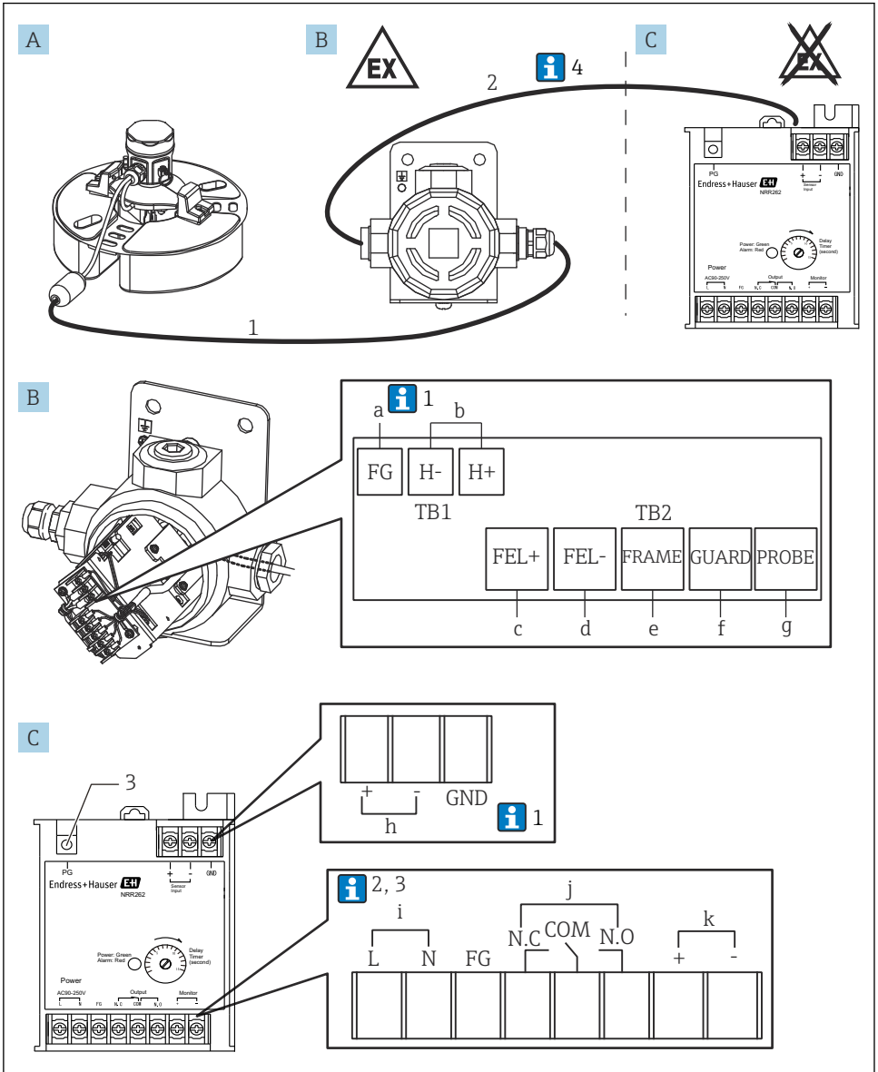
15 Ex [ia] 컨버터 NRR262-4/A/B/C 결선
