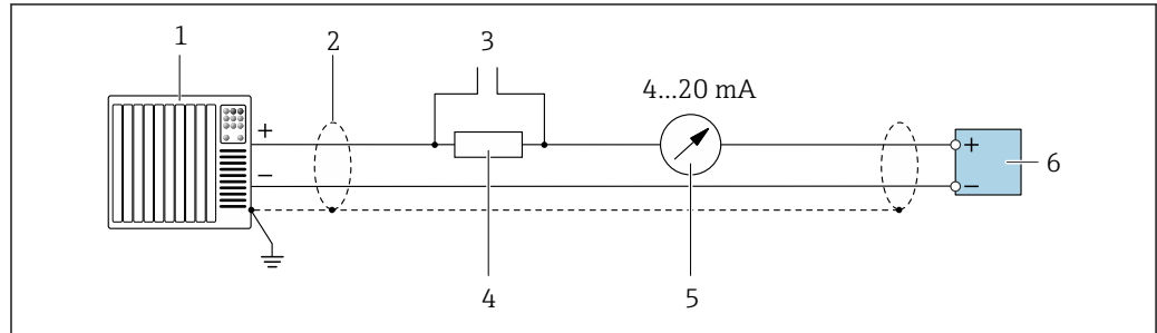
图 11 接线实例：4...20 mA HART 电流输出（有源信号）
