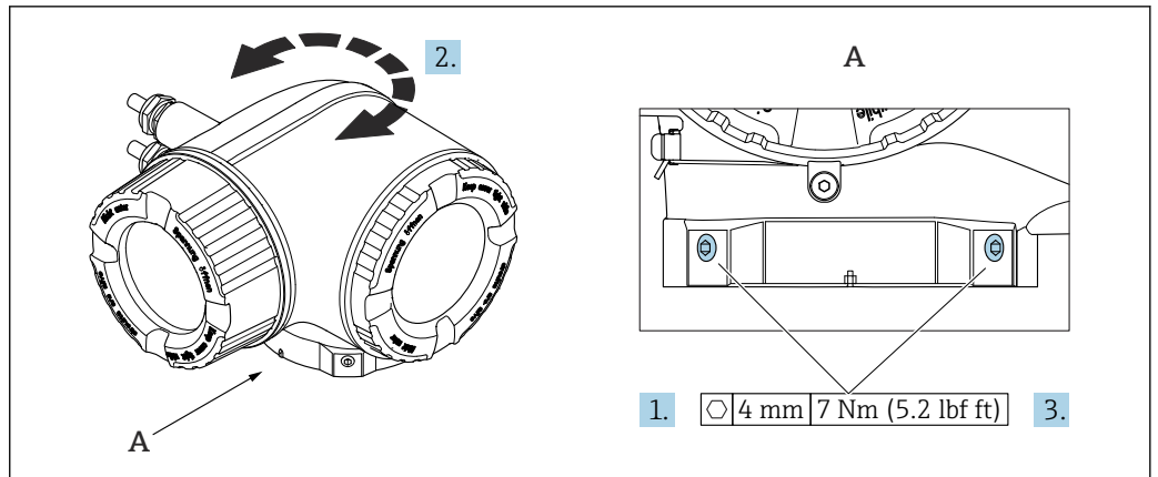
图 9 防爆型外壳
