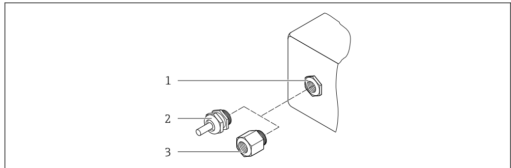
图 39 允许的电缆入口/缆塞
