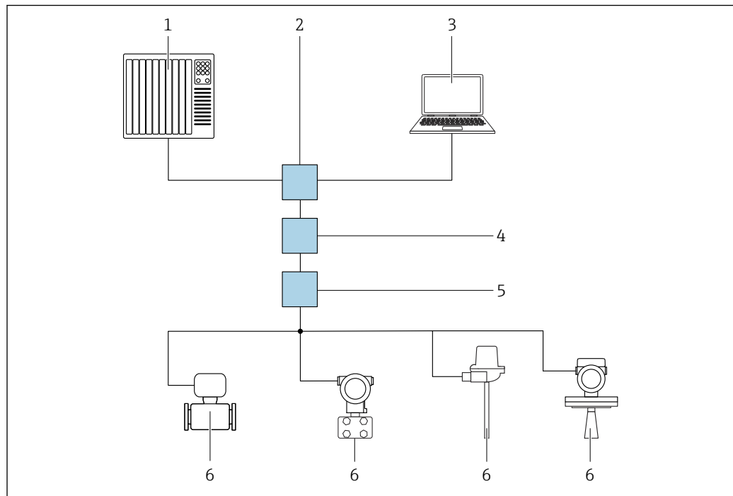
7 Opzioni per controllo a distanza mediante PROFINET con rete Ethernet-APL: topologia a stella
