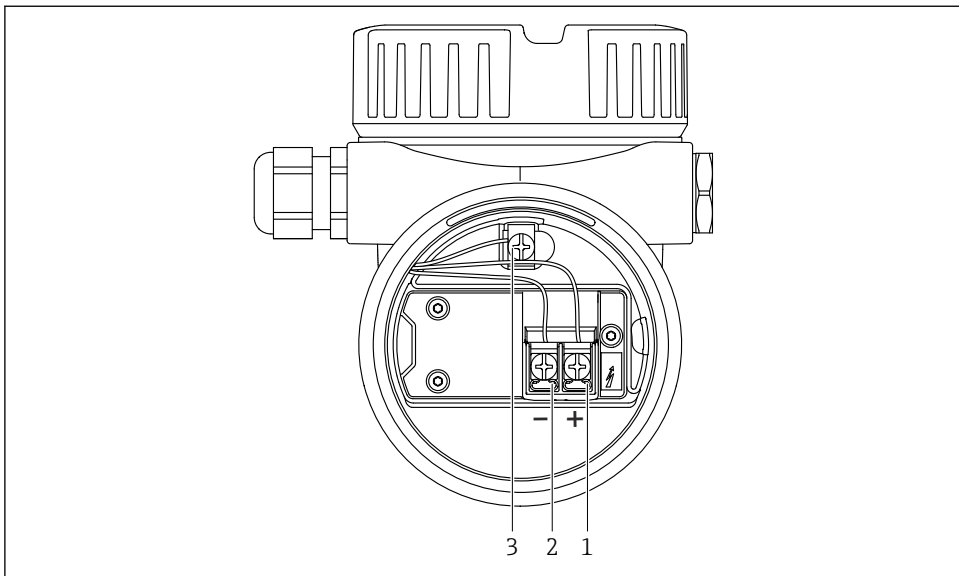
▣ 6 Соединительные клеммы и клемма заземления в клеммном отсеке
