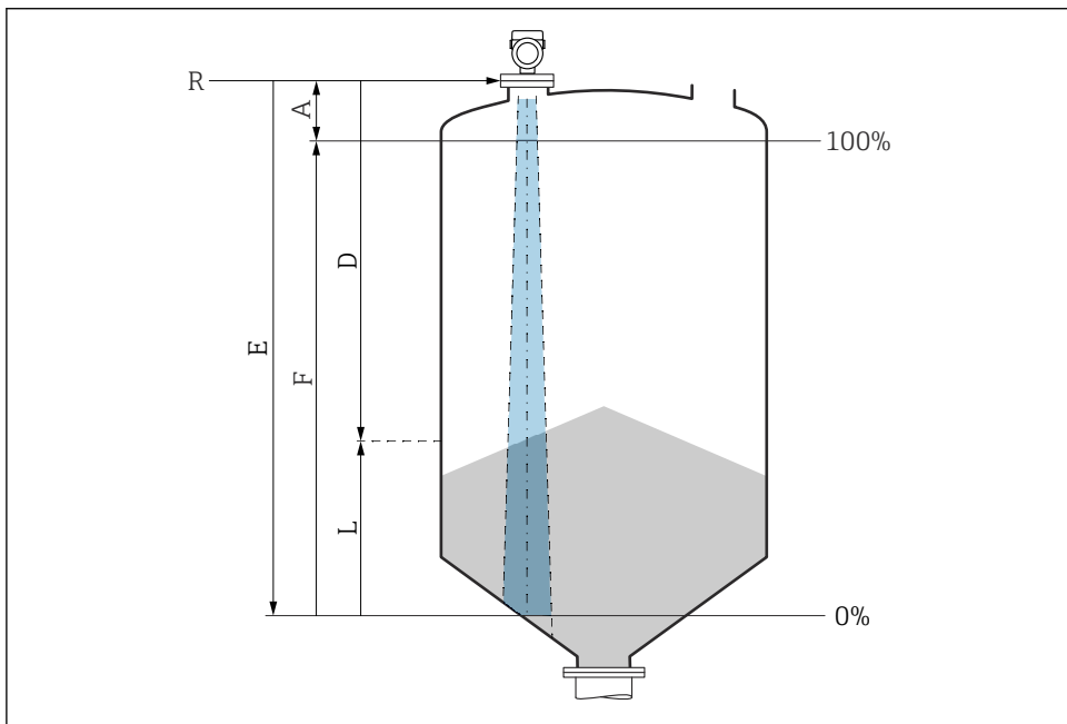
10 Параметры конфигурации для измерения уровня сыпучих сред
