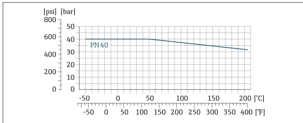
图 31 法兰材质: 1.4404 (F316/F316L)
