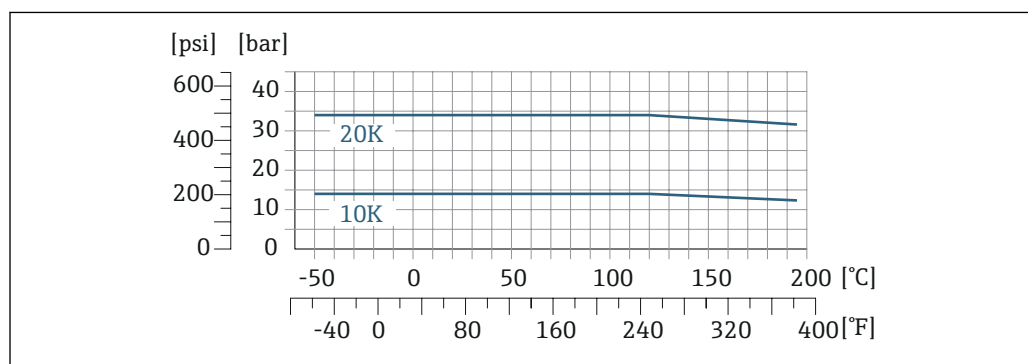
图 33 法兰材质: 1.4404 (F316/F316L)
