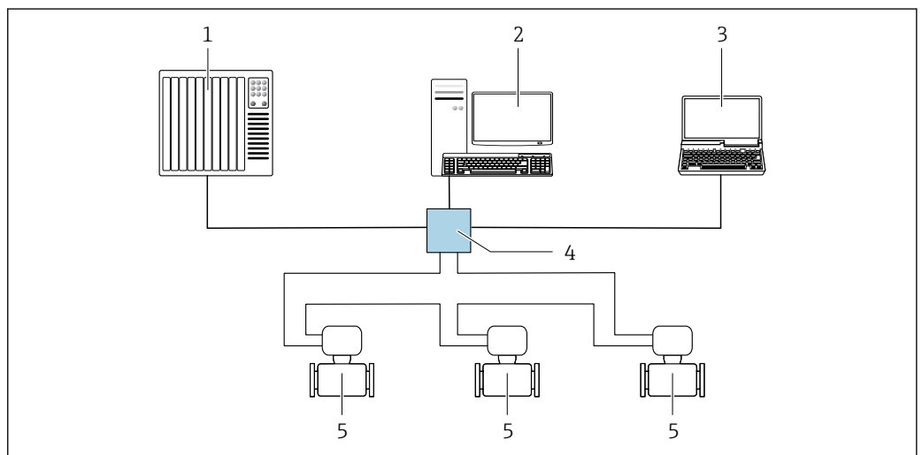
图 79 通过 EtherNet/IP 网络进行远程操作：环形拓扑结构
