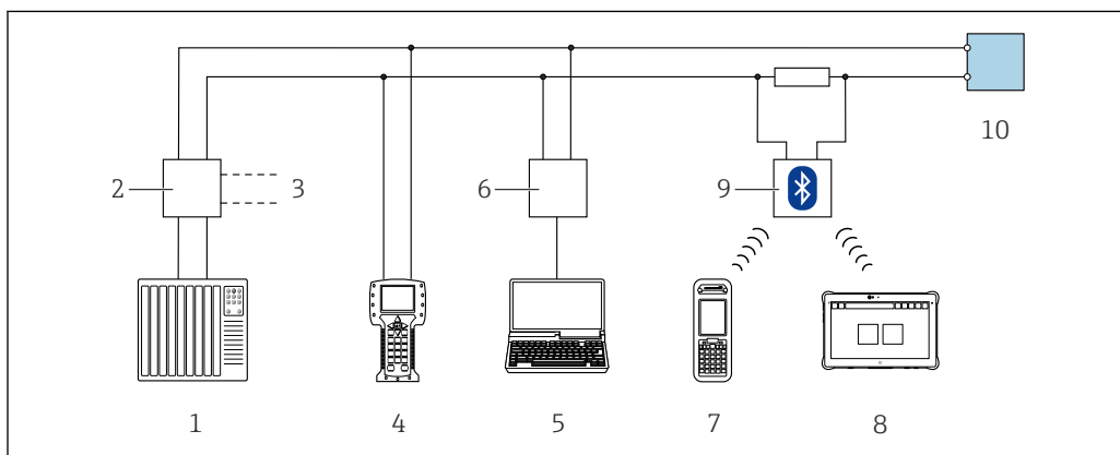
图 73 通过 HART 通信进行远程操作（无源信号）
