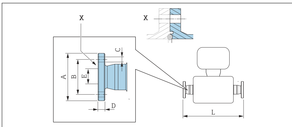
图 43 部件 X: 非对称过程连接; 蓝色部分由供应商提供。
