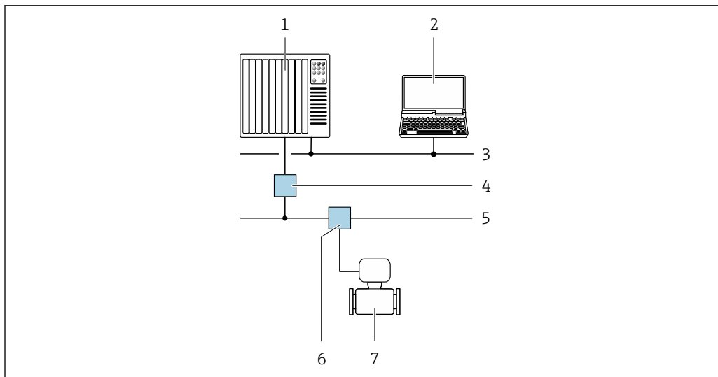
图 76 通过 PROFIBUS PA 网络进行远程操作
