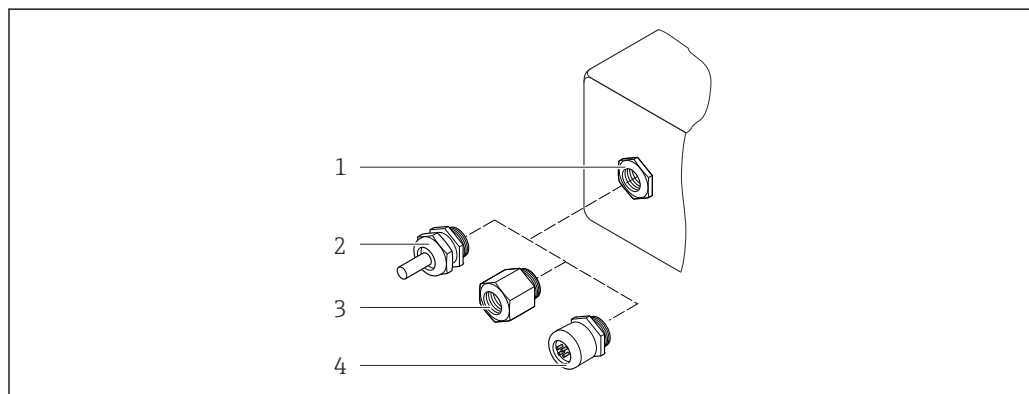
图 70 允许的电缆入口/缆塞
