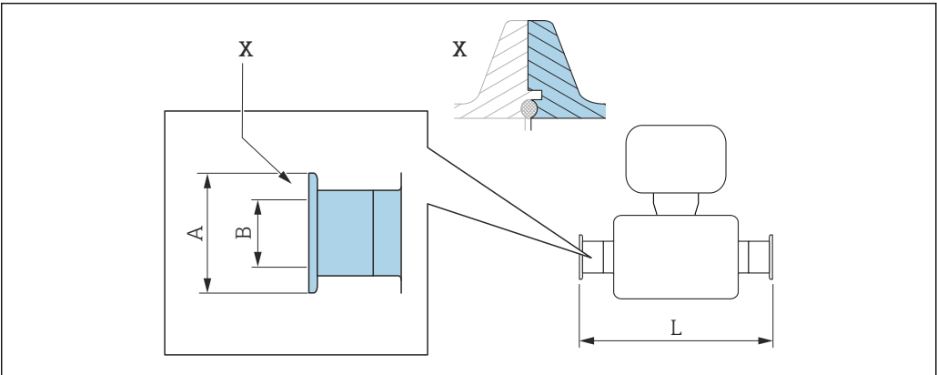
47 部件 X: 非对称过程连接; 蓝色部分由供应商提供。
