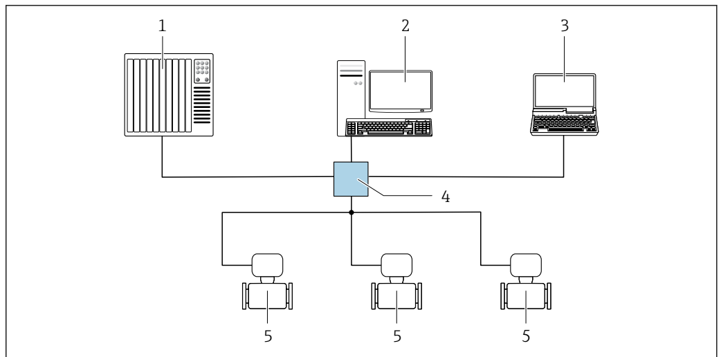
图 78 通过 EtherNet/IP 网络进行远程操作：星形拓扑结构
