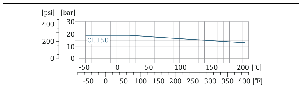
图 32 法兰材质: 1.4404 (F316/F316L)
