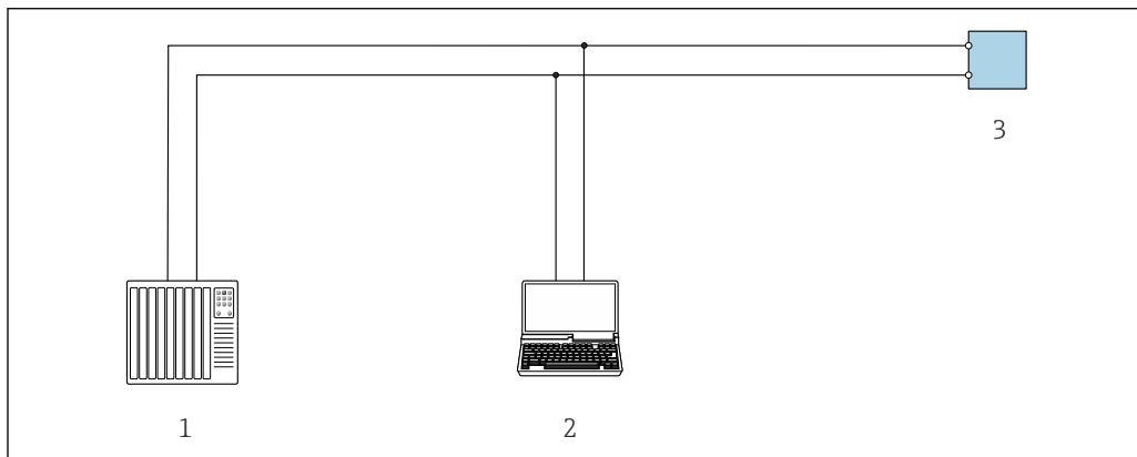
图 77 通过 Modbus-RS485 通信进行远程操作（有源信号）
