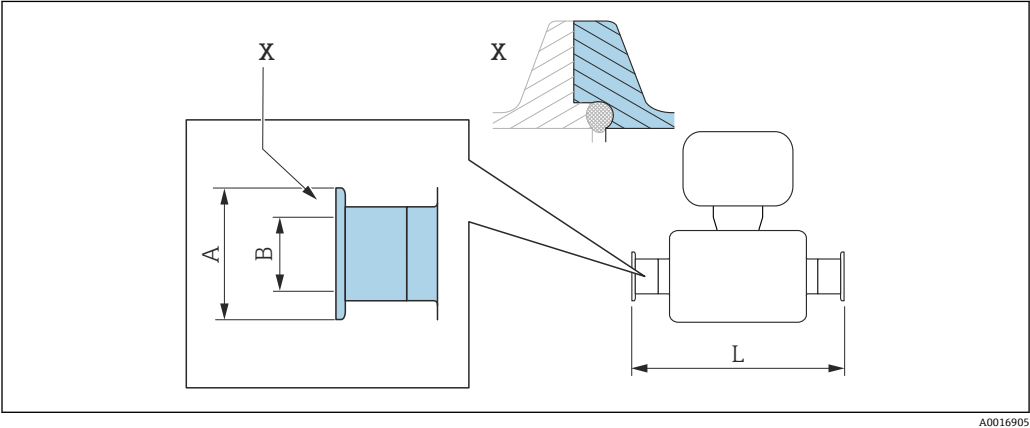
图 48 部件 X: 非对称过程连接; 蓝色部分由供应商提供。
