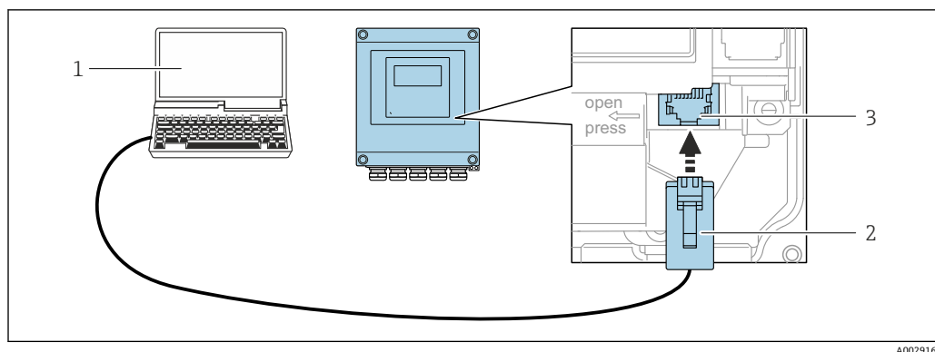
图 83 通过服务接口 (CDI-RJ45) 连接
