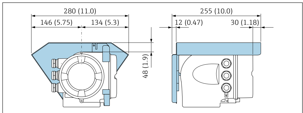
图 54 Proline 500（模拟）变送器的防护罩的外形尺寸图；单位：mm (in)
