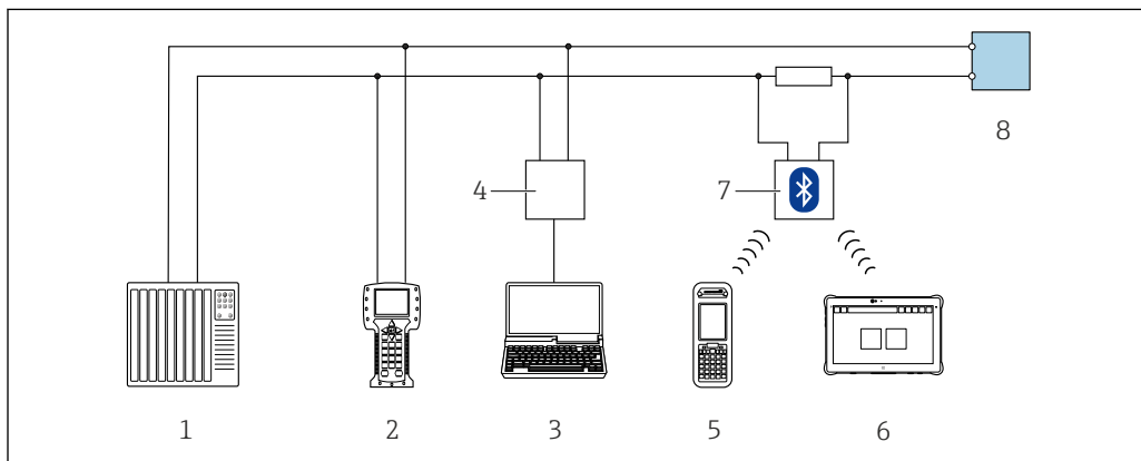
图 72 通过 HART 通信进行远程操作（有源信号）
