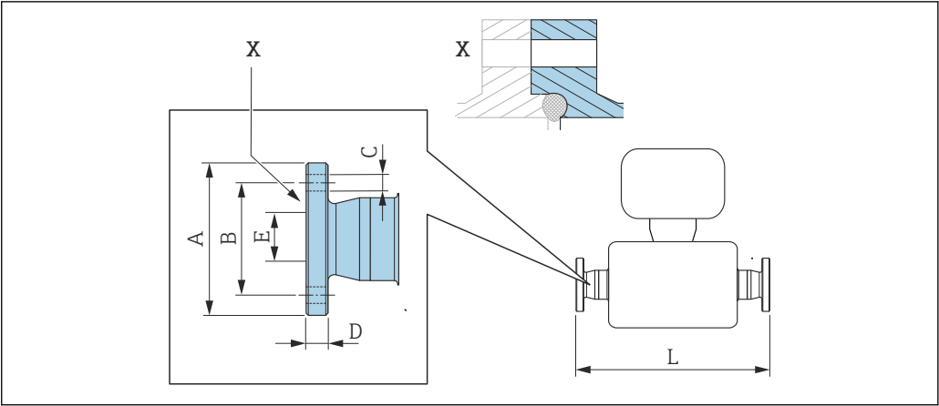
44 部件 X: 非对称过程连接; 蓝色部分由供应商提供。
