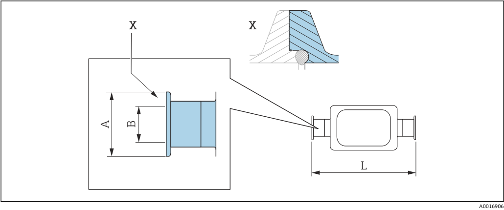
图 51 部件 X: 非对称过程连接; 蓝色部分由供应商提供。
