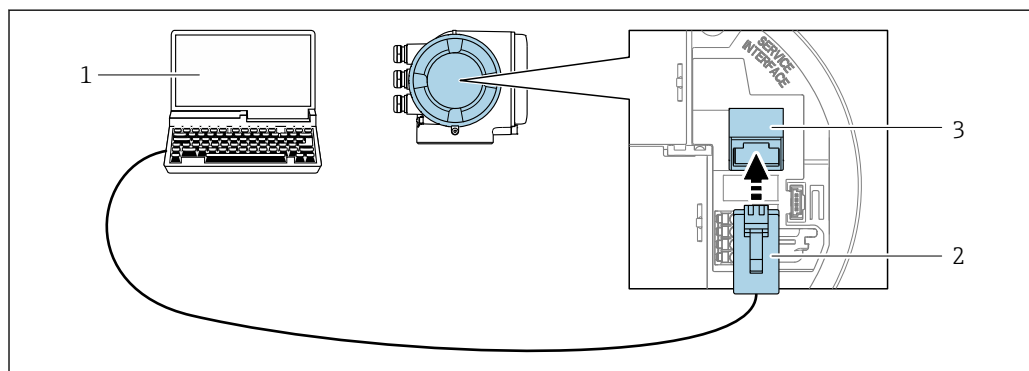
图 84 通过服务接口 (CDI-RJ45) 连接
