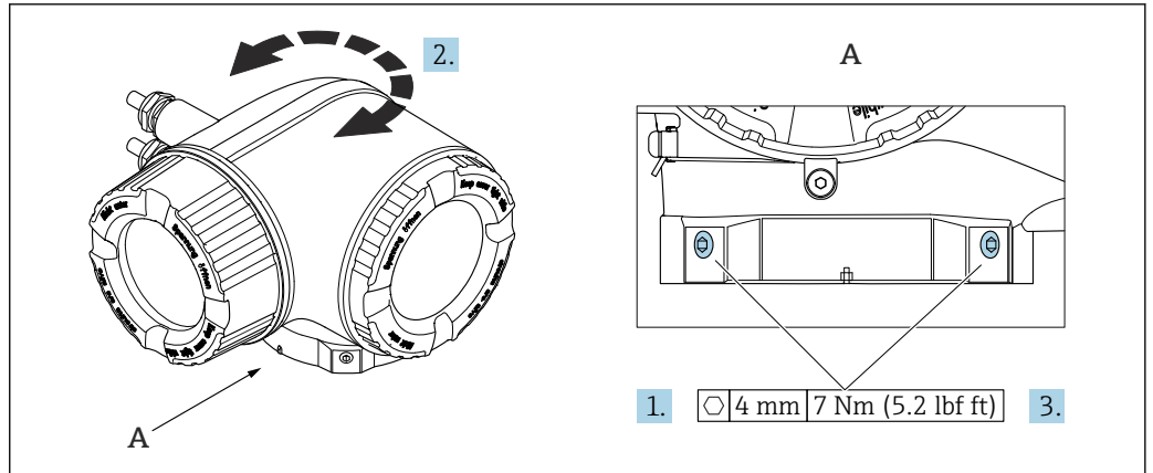
15 防爆型外壳
