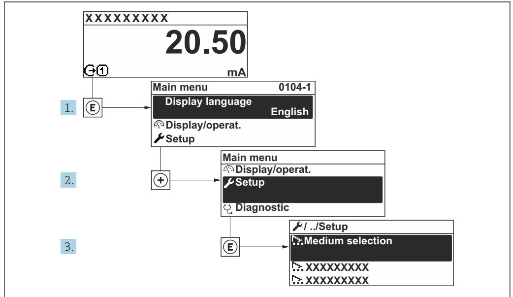
35 现场显示单元示例
